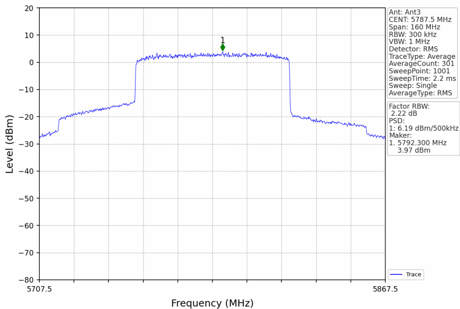
80M_MCH_5787.5MHz_Ant3_NTNV
