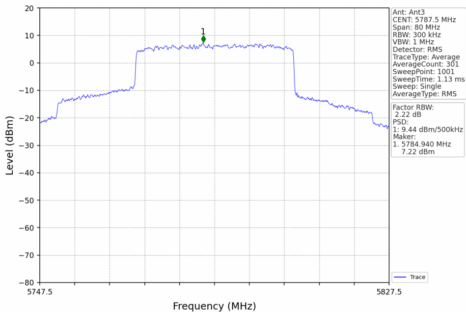
40M_MCH_5787.5MHz_Ant3_NTNV
