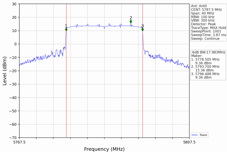
20M_MCH_5787.5MHz_Ant0_NTNV
