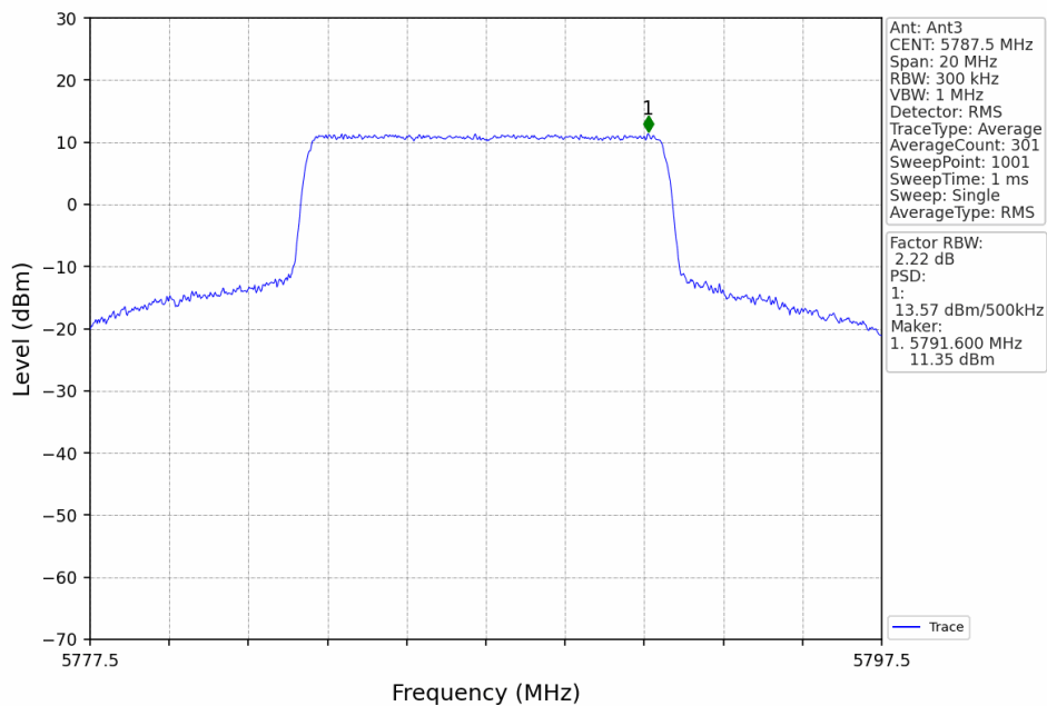
10M_MCH_5787.5MHz_Ant3_NTNV
