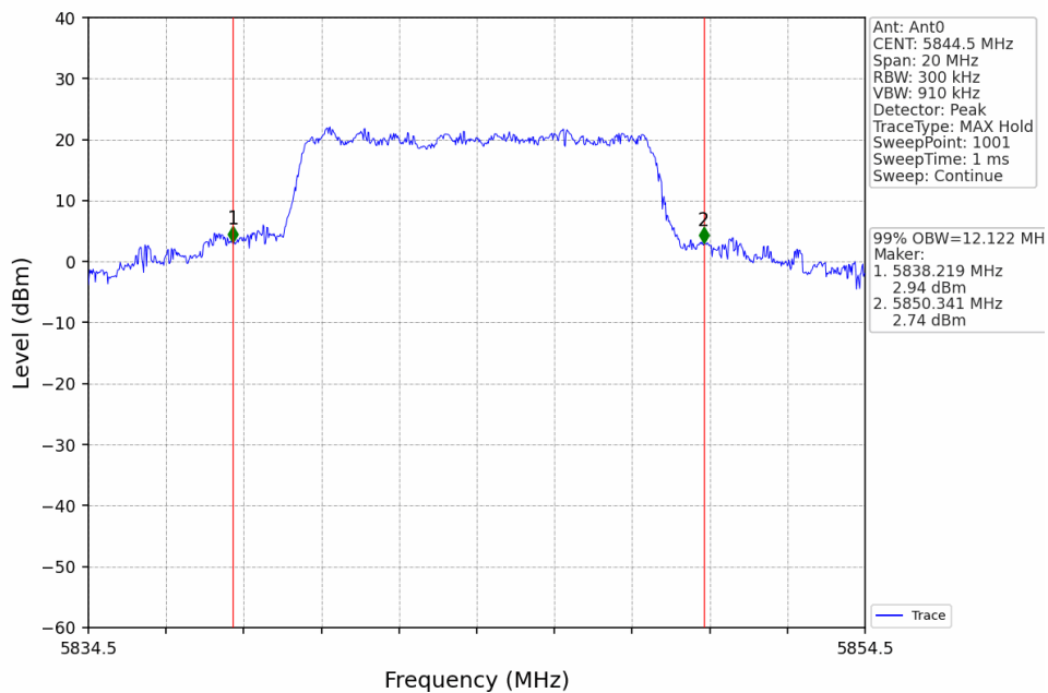
10M_HCH_5844.5MHz_Ant0_NTNV
