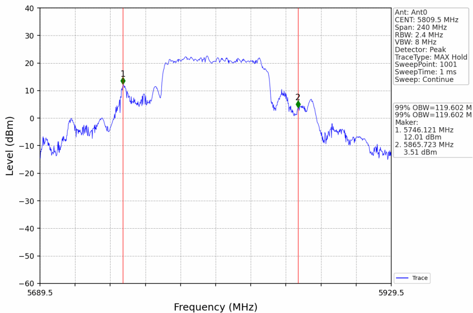
80M_HCH_5809.5MHz_Ant0_NTNV
