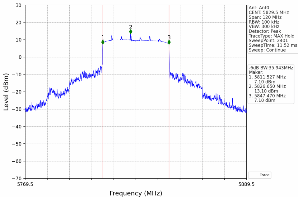
40M_HCH_5829.5MHz_Ant0_NTNV
