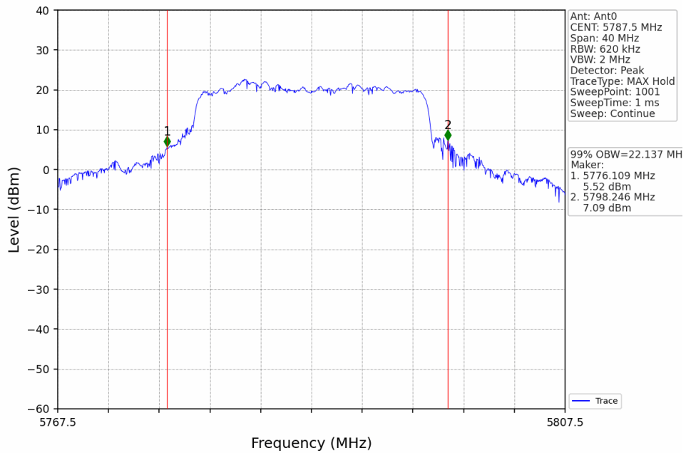
20M_MCH_5787.5MHz_Ant0_NTNV
