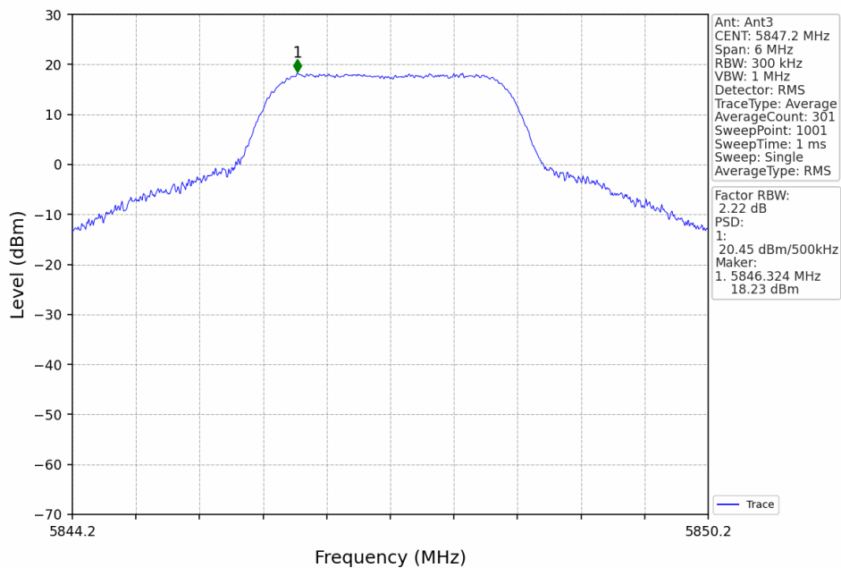
3M_HCH_5847.2MHz_Ant3_NTNV
