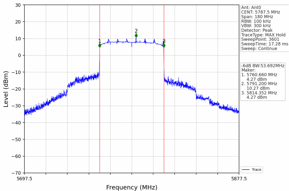
60M_MCH_5787.5MHz_Ant0_NTNV
