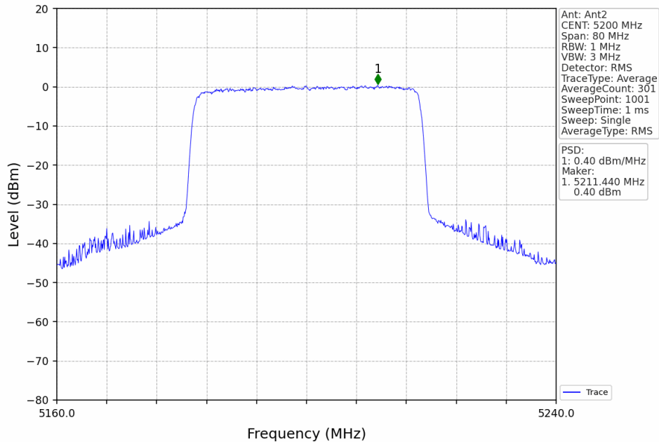
40M_MCH_5200MHz_MIMO_NTNV
