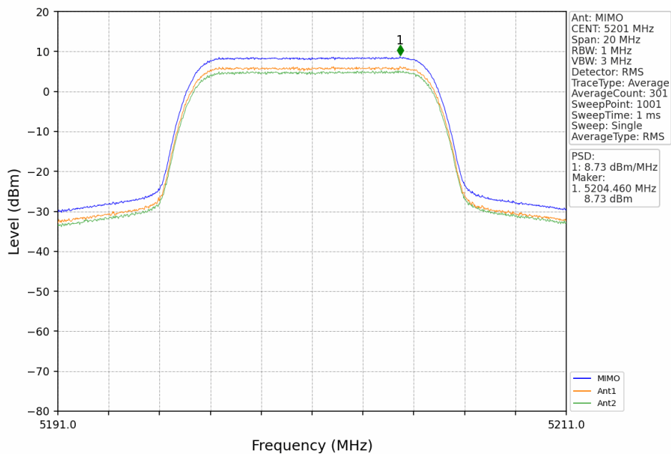
10M_MCH_5201MHz_MIMO_NTNV
