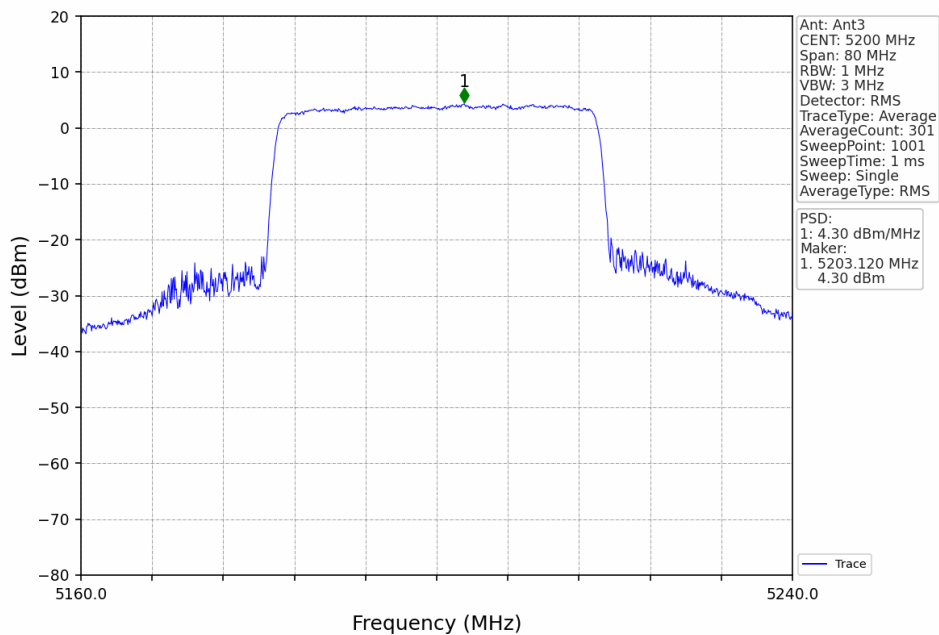
40M_MCH_5200MHz_Ant3_NTNV
