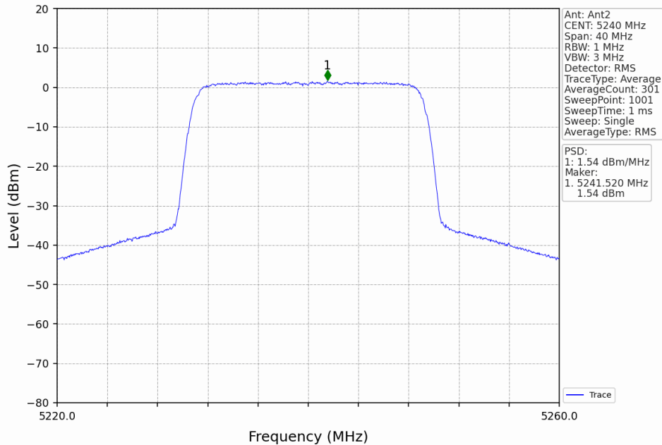
20M_HCH_5240MHz_MIMO_NTNV
