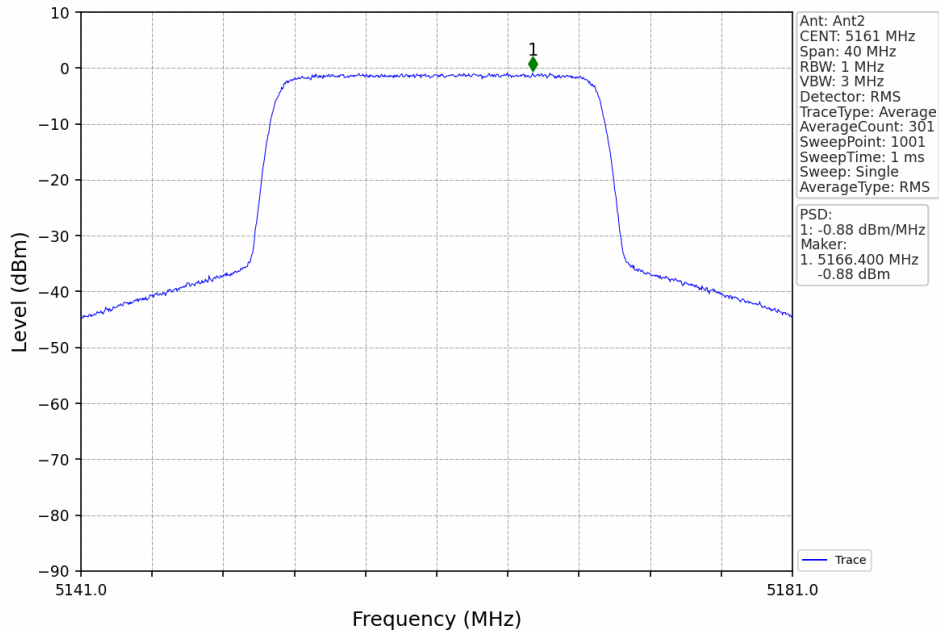
20M_LCH_5161MHz_MIMO_NTNV
