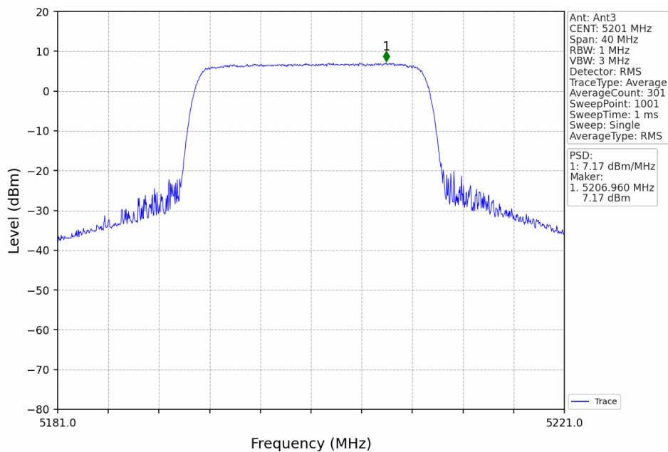
20M_MCH_5201MHz_Ant3_NTNV
