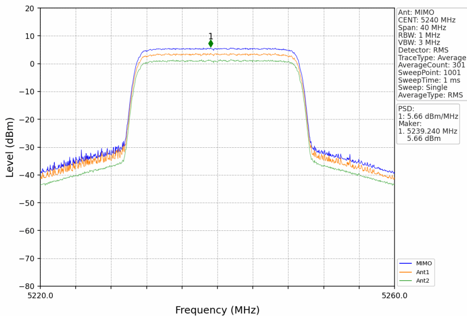
20M_HCH_5240MHz_MIMO_NTNV
