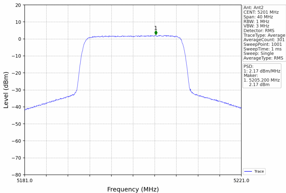
20M_MCH_5201MHz_Ant2_NTNV
