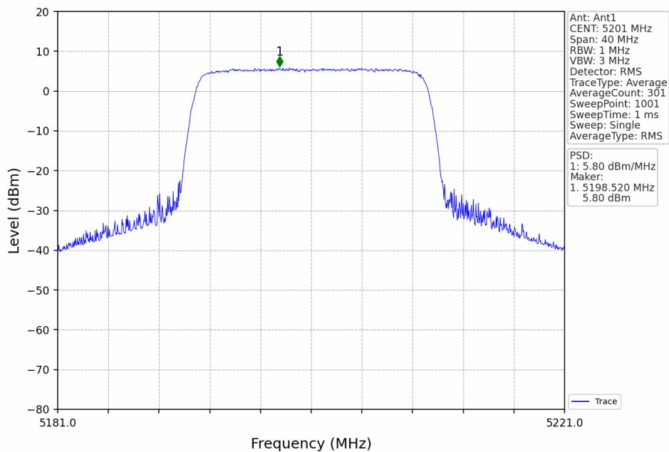
20M_MCH_5201MHz_Ant1_NTNV
