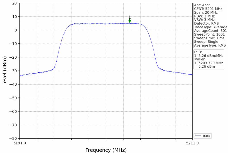
10M_MCH_5201MHz_MIMO_NTNV
