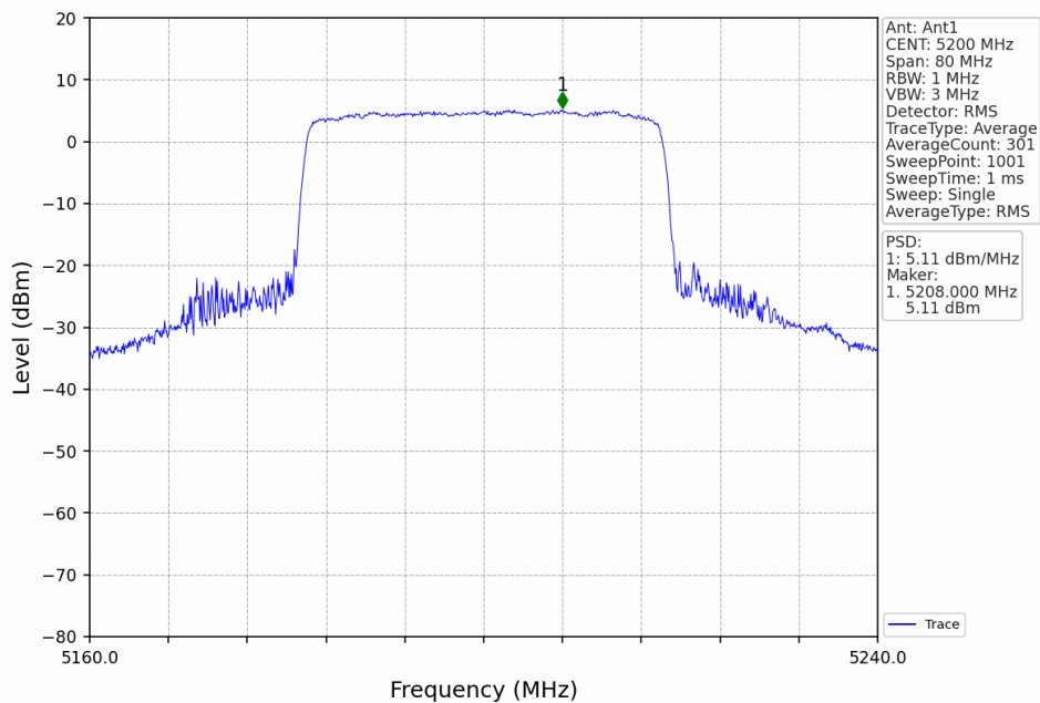
40M_MCH_5200MHz_Ant1_NTNV
