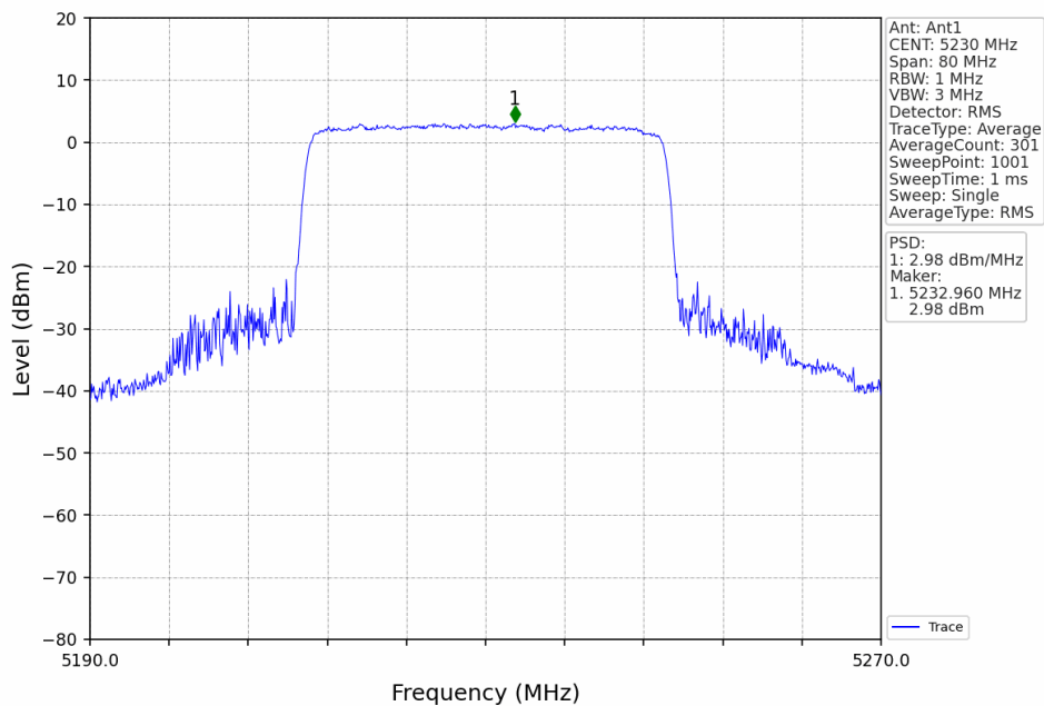
40M_HCH_5230MHz_Ant1_NTNV
