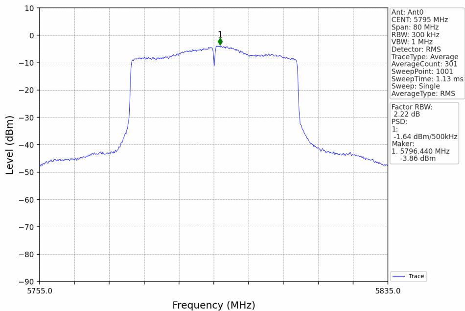
802.11ax(HEW40)_HCH_5795MHz_RU484_Left_Ant0_NTNV
