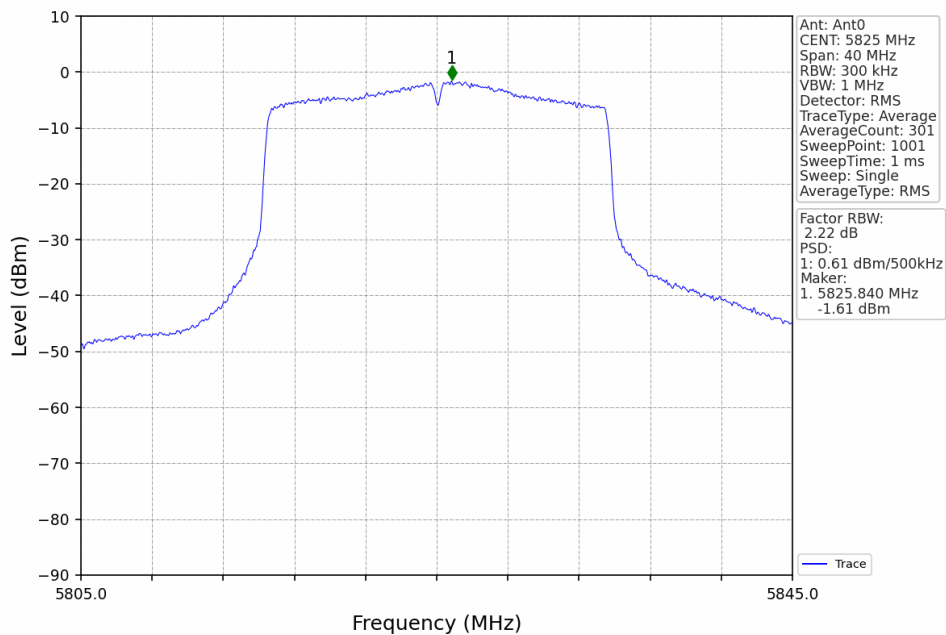
802.11ax(HEW20)_HCH_5825MHz_RU242_Left_Ant0_NTNV
