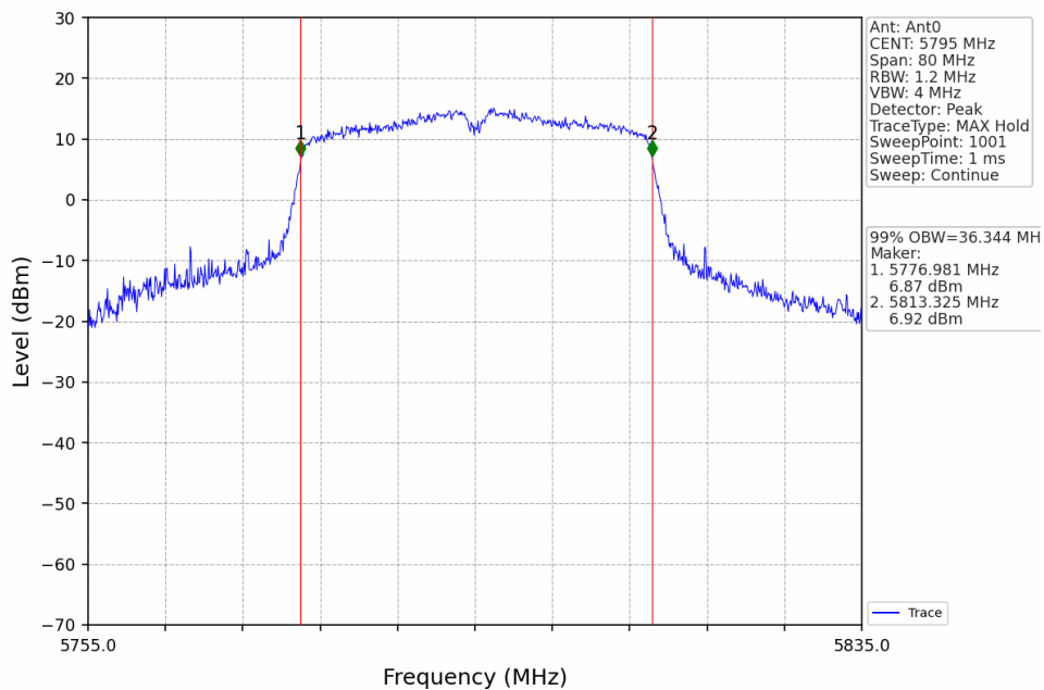
802.11ac(VHT40)_HCH_5795MHz_Ant0_NTNV
