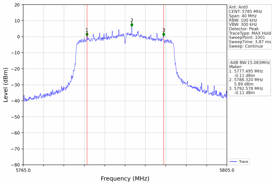
802.11ax(HEW20)_MCH_5785MHz_RU242_Left_Ant0_NTNV
