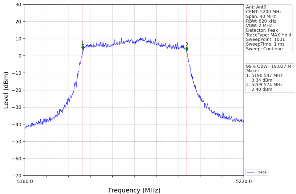
802.11ax(HEW20)_MCH_5200MHz_RU242_Left_Ant0_NTNV
