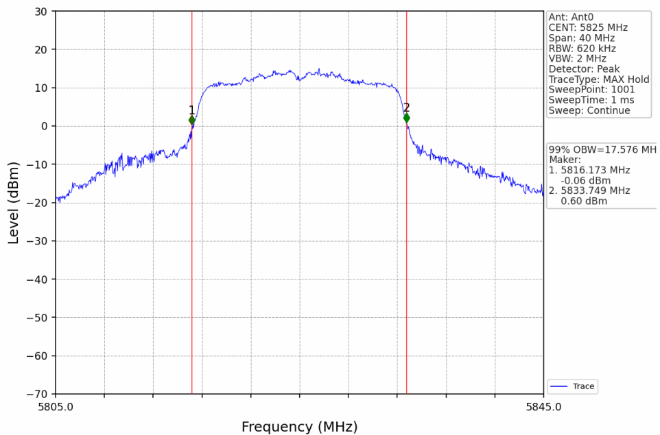
802.11a_HCH_5825MHz_Ant0_NTNV
