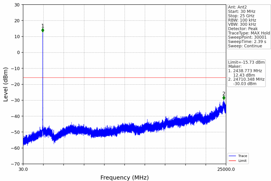
10M_MCH_2437.5MHz_Ant2_NTNV
