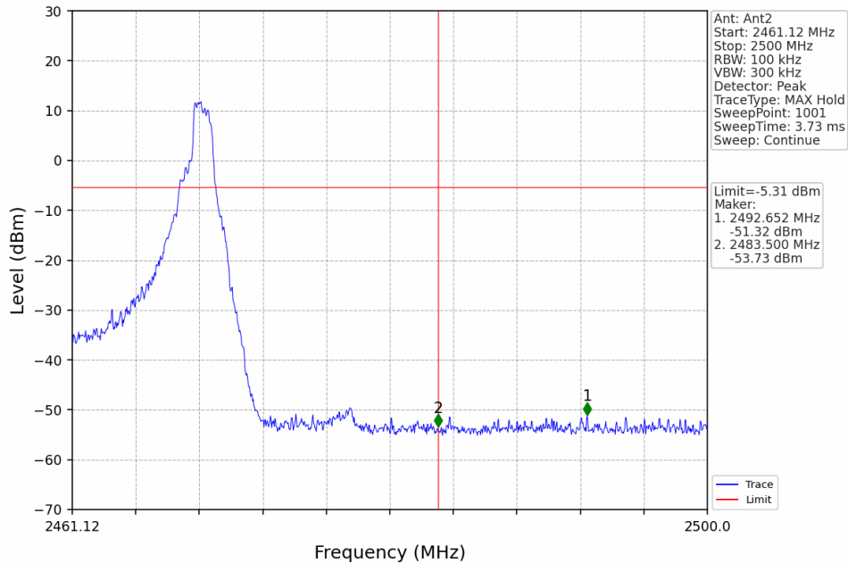
1.4M_HCH_2469.12MHz_Ant2_NTNV
