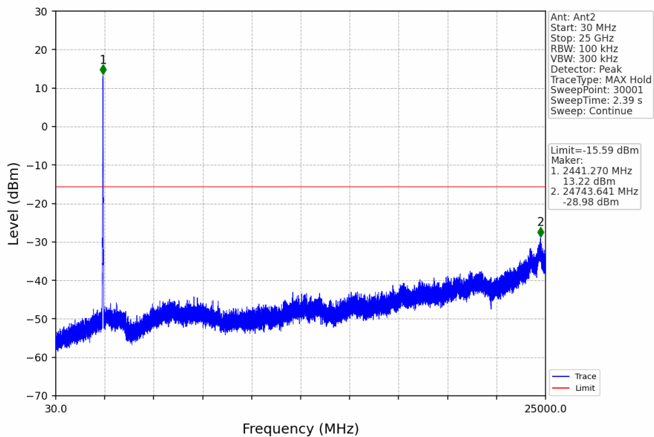
20M_MCH_2437.5MHz_Ant2_NTNV
