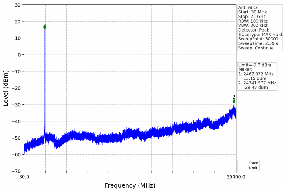
3M_HCH_2468.2MHz_Ant2_NTNV
