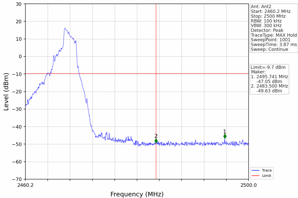
3M_HCH_2468.2MHz_Ant2_NTNV
