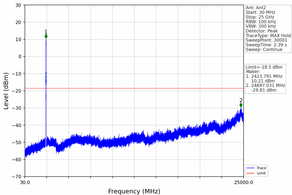
40M_MCH_2437.5MHz_Ant2_NTNV
