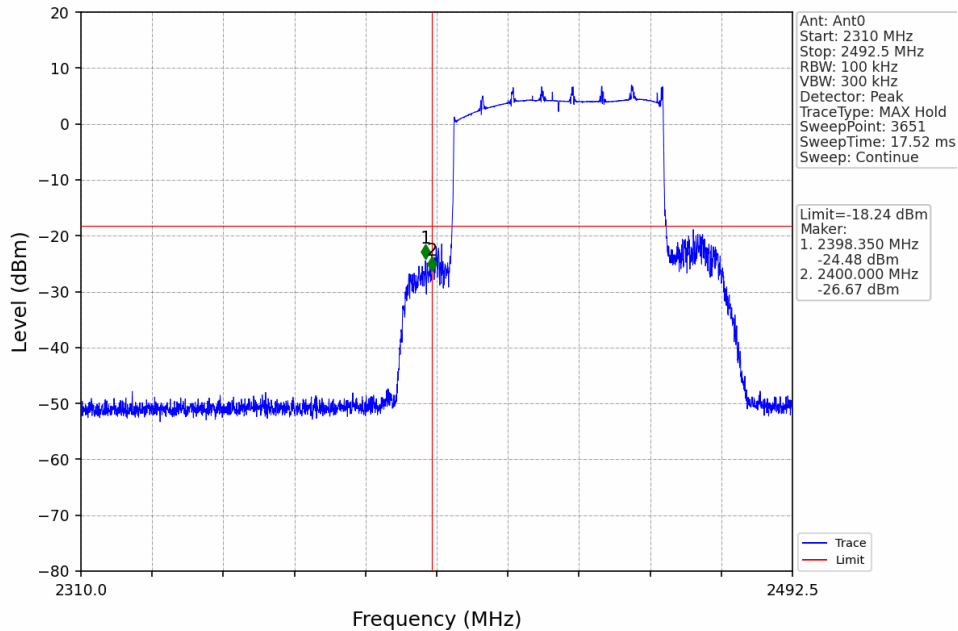
60M_LCH_2432.5MHz_Ant0_NTNV
