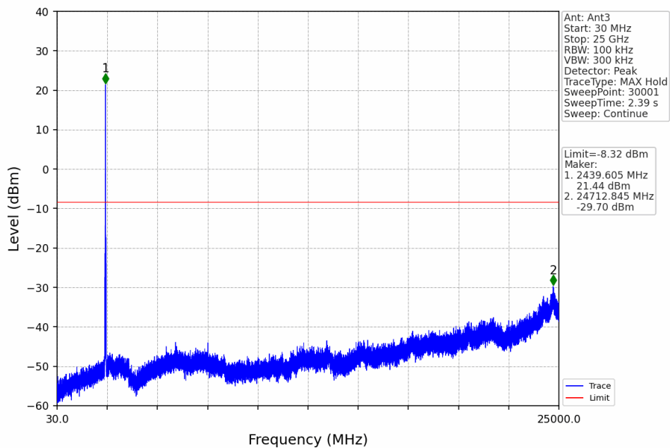
5M_MCH_2437.74MHz_Ant3_NTNV
