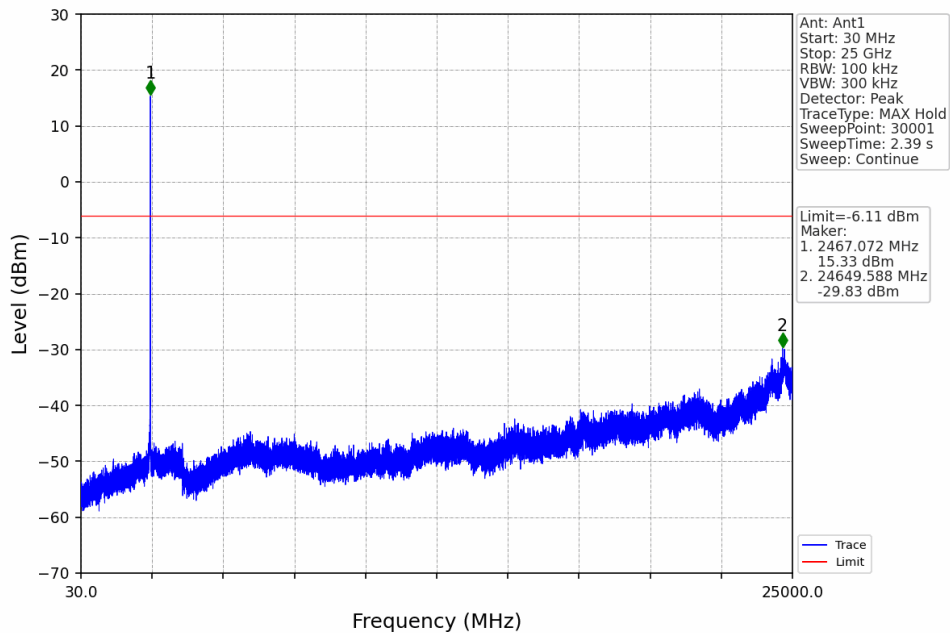
3M_HCH_2468.2MHz_Ant1_NTNV
