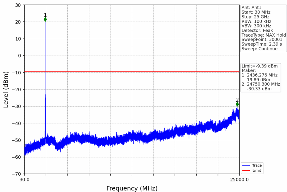
5M_MCH_2437.74MHz_Ant1_NTNV
