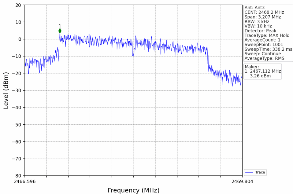
3M_HCH_2468.2MHz_Ant3_NTNV
