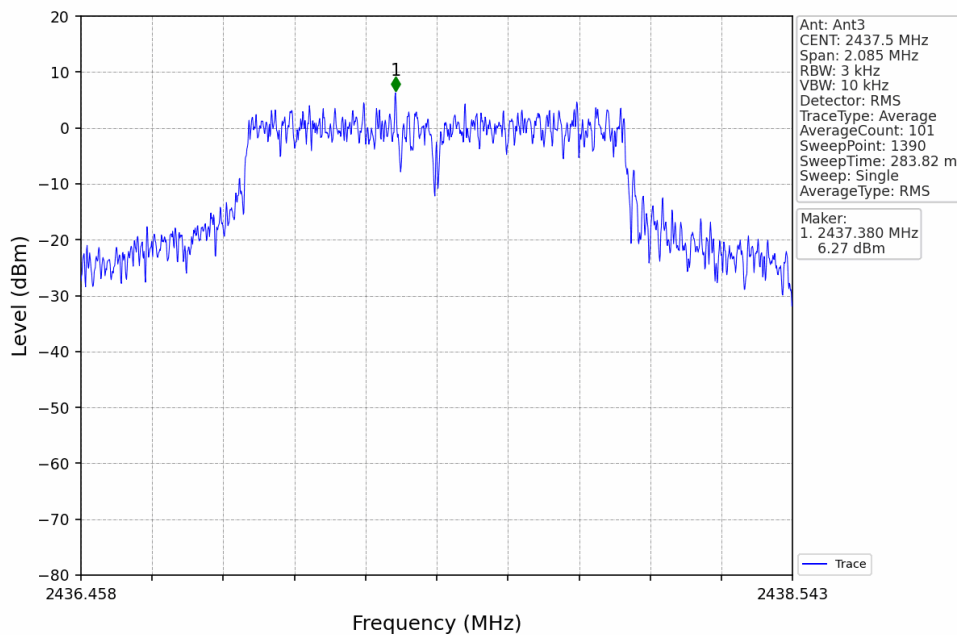
1.4M_MCH_2437.5MHz_Ant3_NTNV
