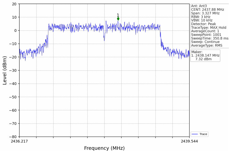
3M_MCH_2437.88MHz_Ant3_NTNV
