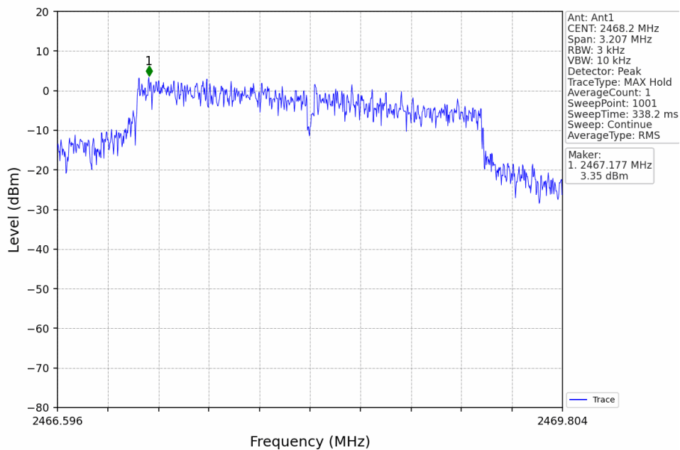
3M_HCH_2468.2MHz_Ant1_NTNV
