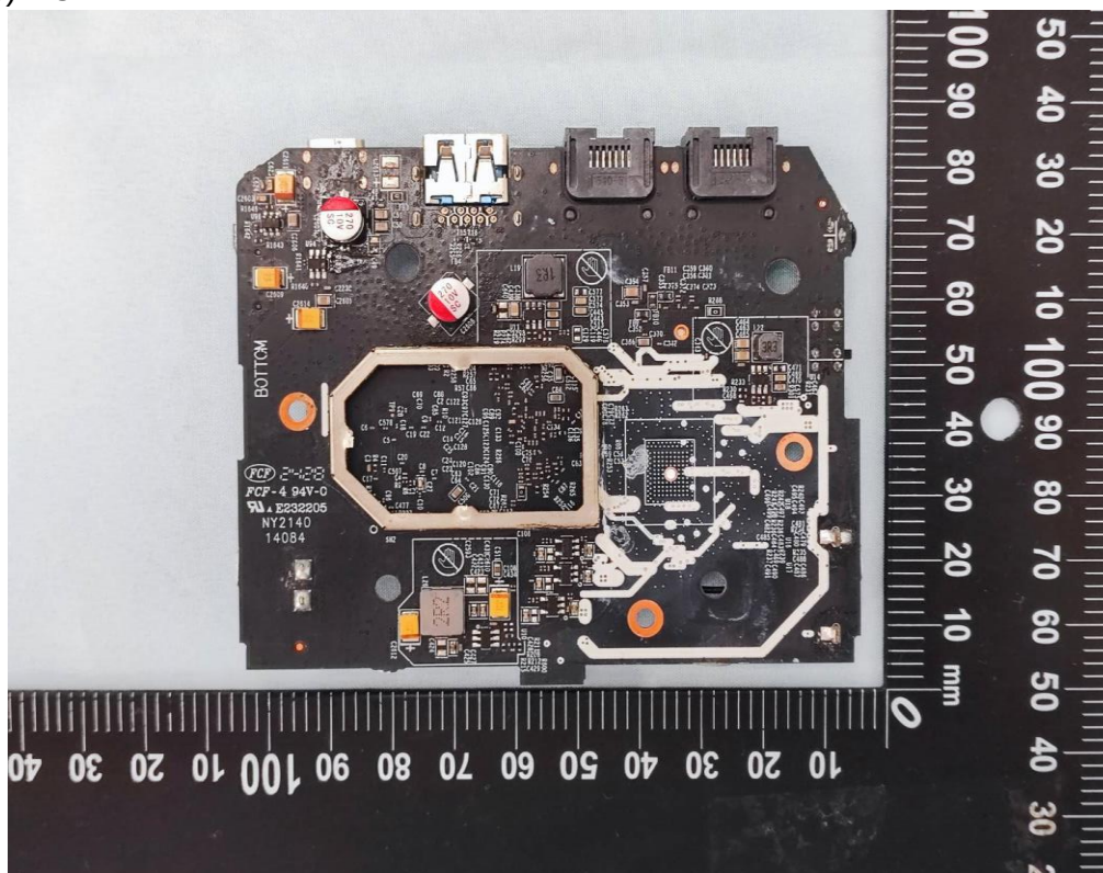
(18) EUT Photo
