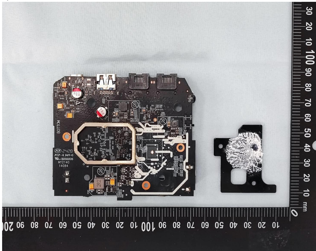
(18) EUT Photo
