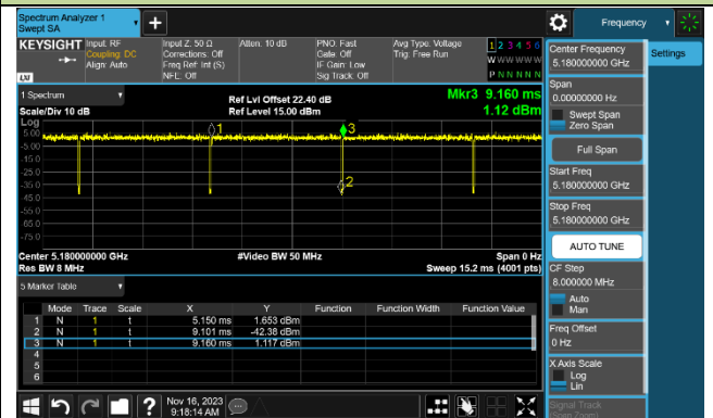
802.11be-EHT20
