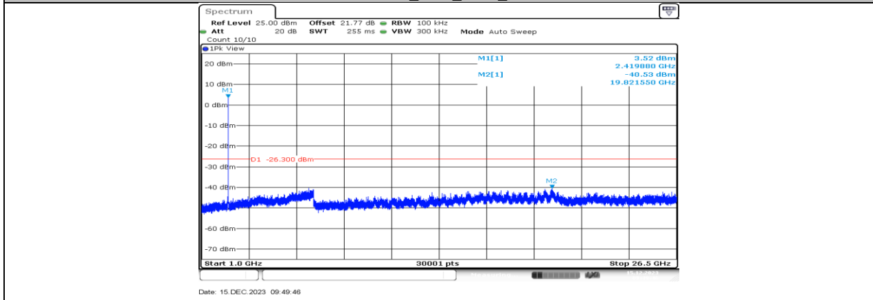
11AX20MIMO_Ant2_2417_1000~26500
