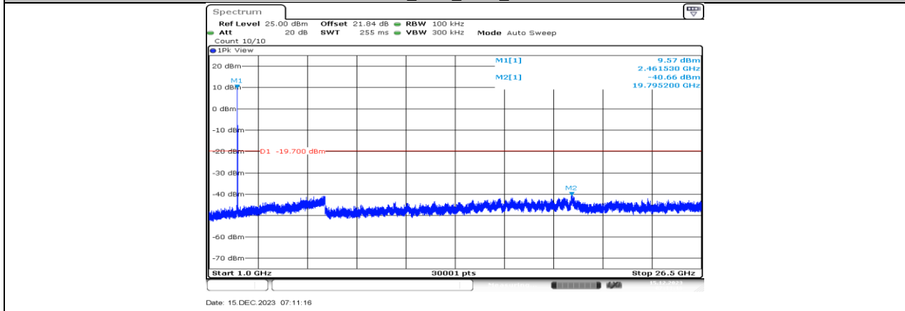
11B-CDD_Ant1_2462_1000~26500
