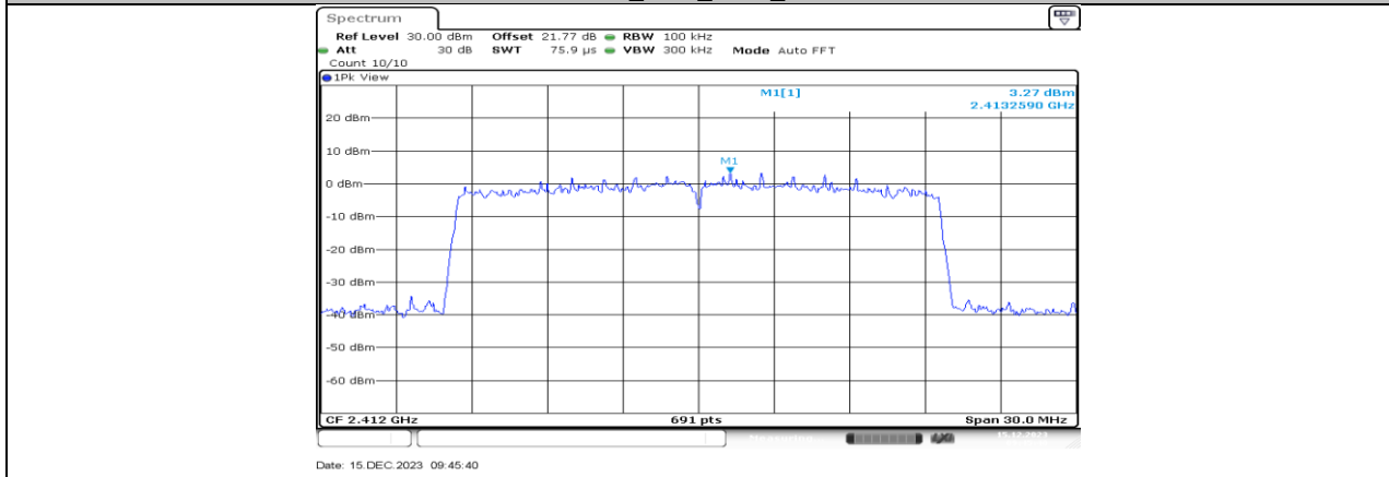
11AX20MIMO_Ant2_2412_0~Reference
