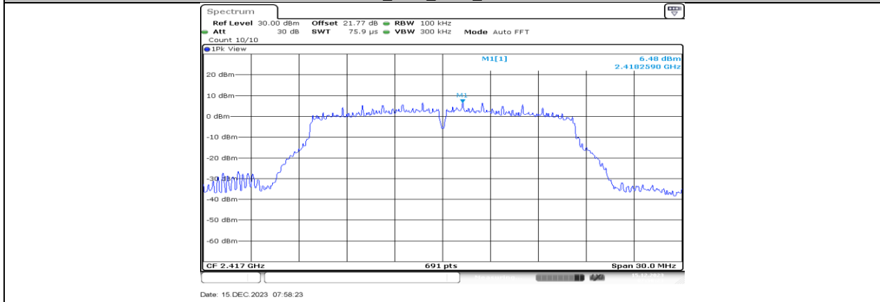
11G-CDD_Ant2_2417_0~Reference
