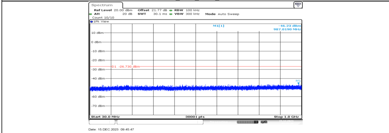
11AX20MIMO_Ant2_2412_30~1000
