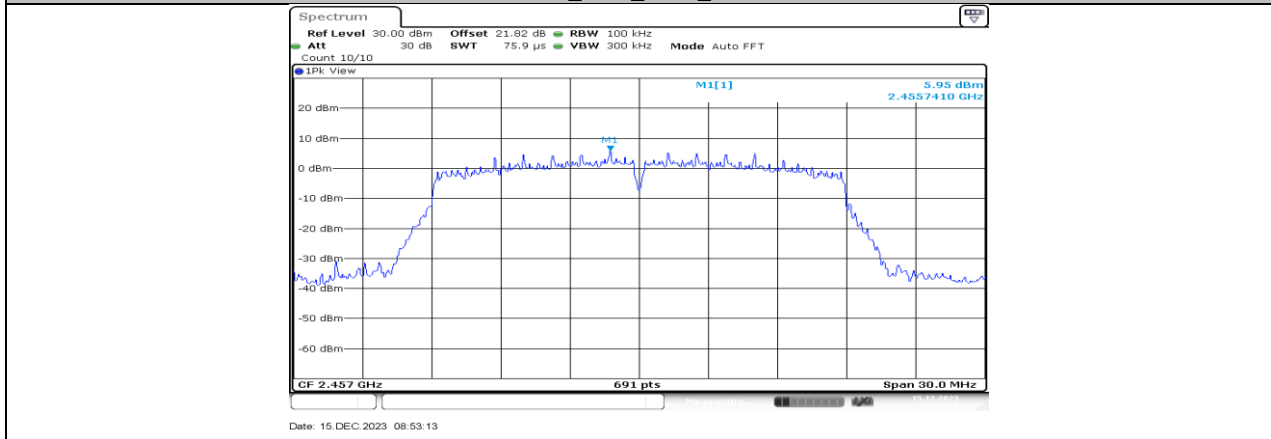
11N20MIMO_Ant2_2457_0~Reference
