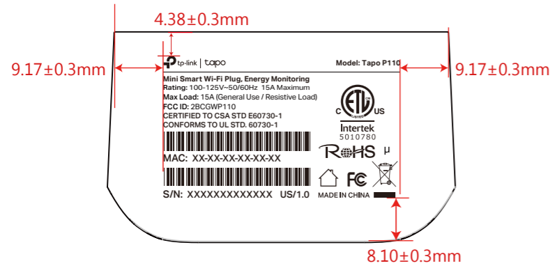
尺寸图
