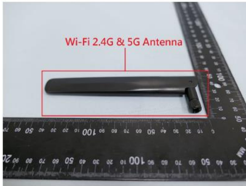
(14) EUT Photo
