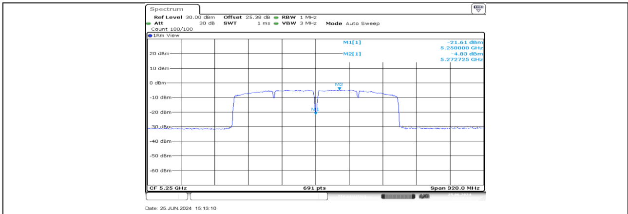
11AC160MIMO_Ant1_5250_UNII-2A
