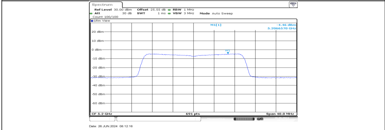
11AX20MIMO_Ant3_5200
