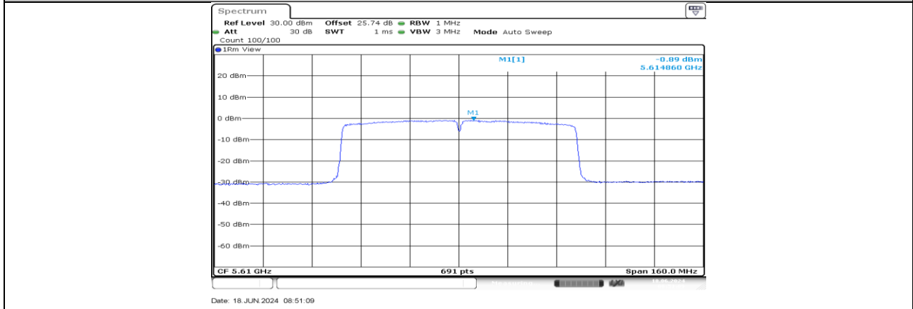
11AC80MIMO_Ant2_5610
