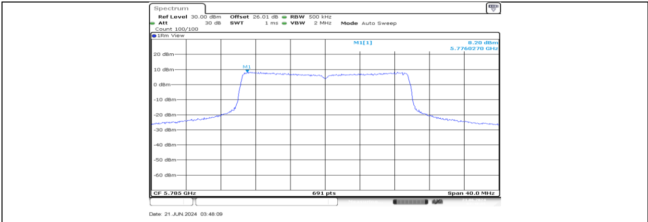
11AX20MIMO_Ant1_5785
