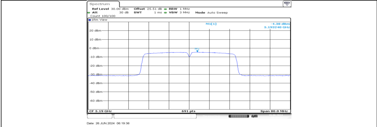
11AC40MIMO_Ant3_5190
