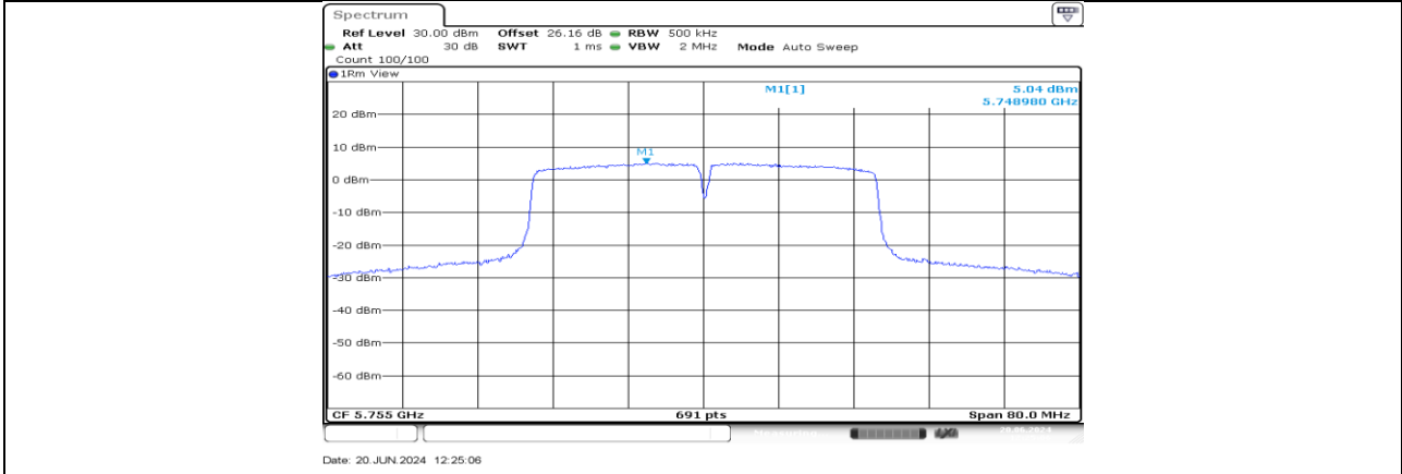
11AC40MIMO_Ant2_5755
