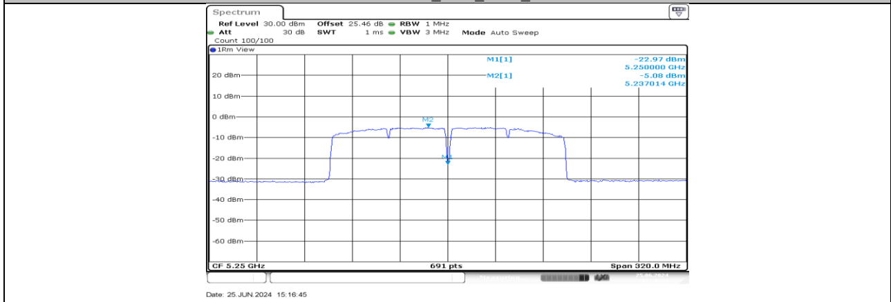
11AC160MIMO_Ant4_5250_UNII-1
