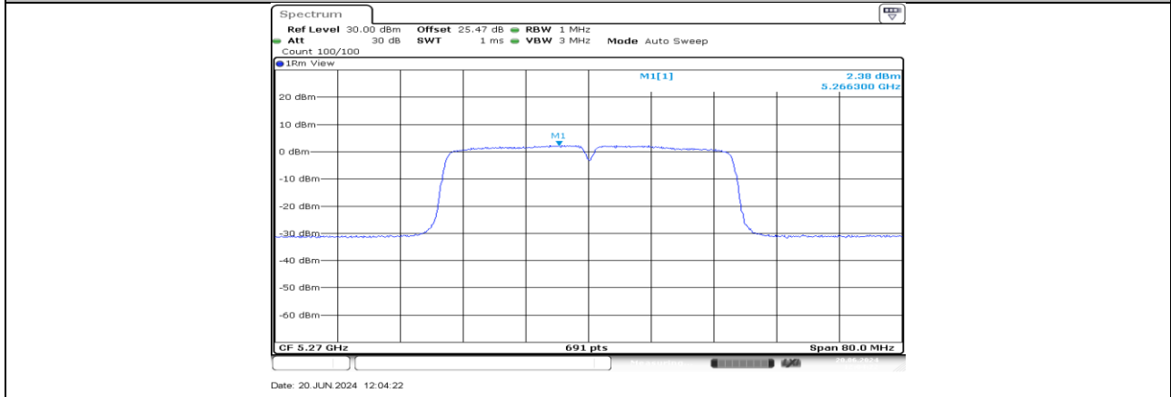
11AC40MIMO_Ant4_5270
