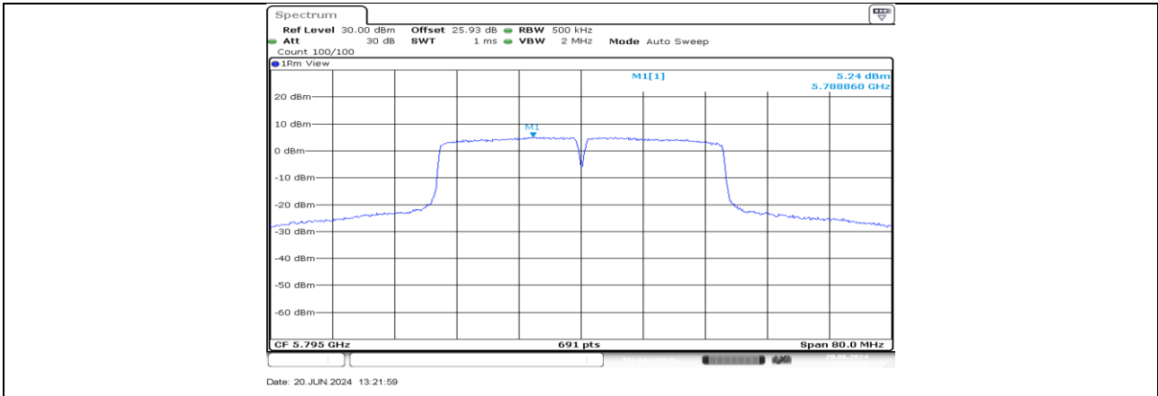
11AC40MIMO_Ant2_5795
