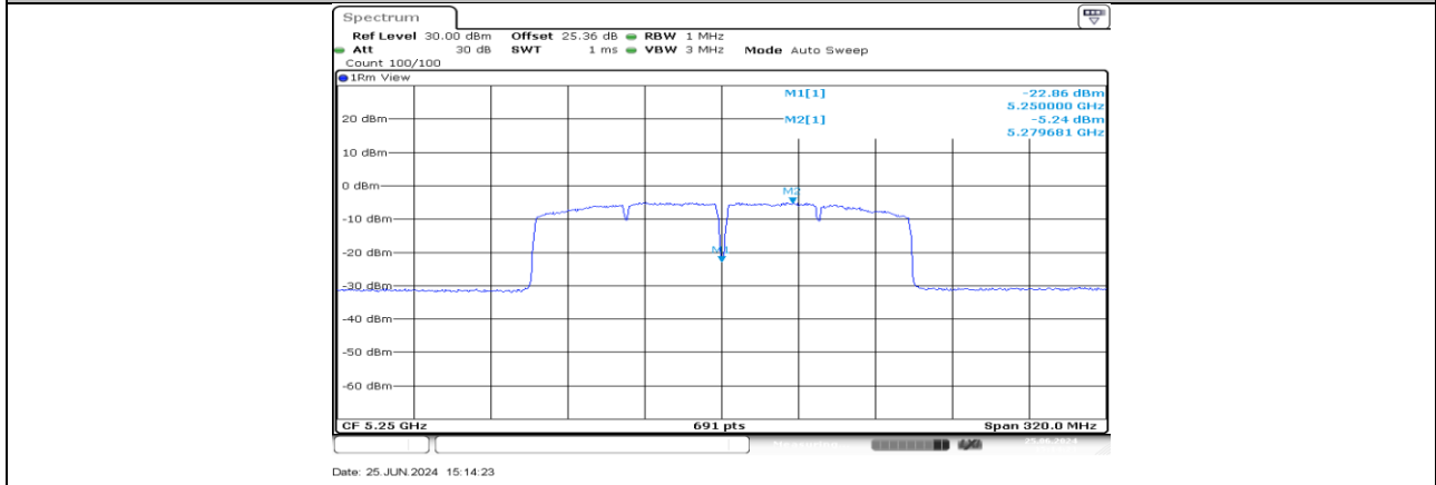
11AC160MIMO_Ant2_5250_UNII-2A
