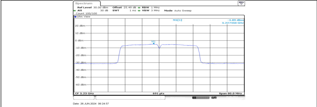
11AC40MIMO_Ant4_5230
