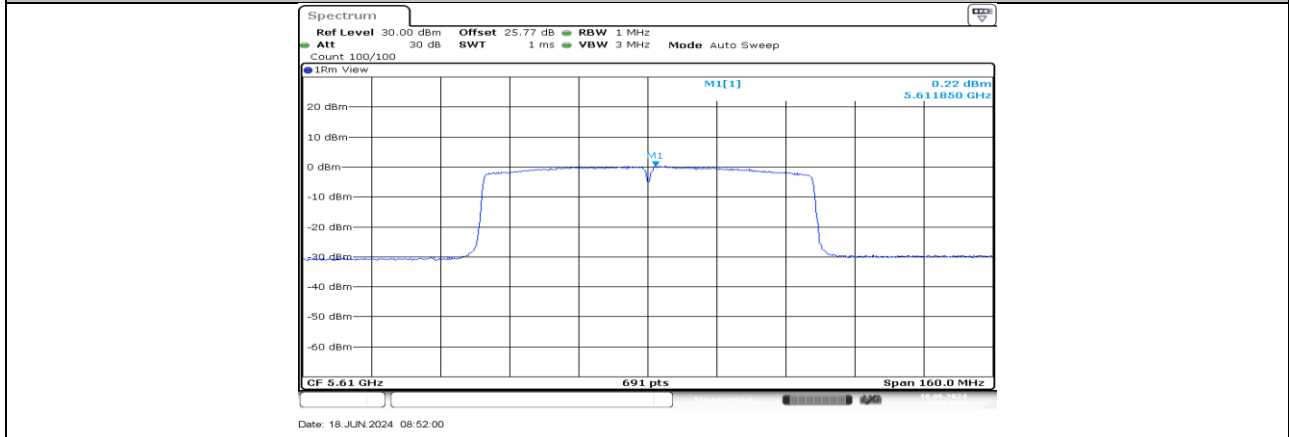
11AC80MIMO_Ant3_5610
