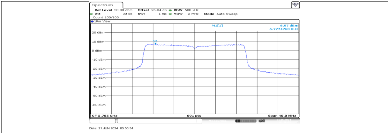
11AX20MIMO_Ant4_5785
