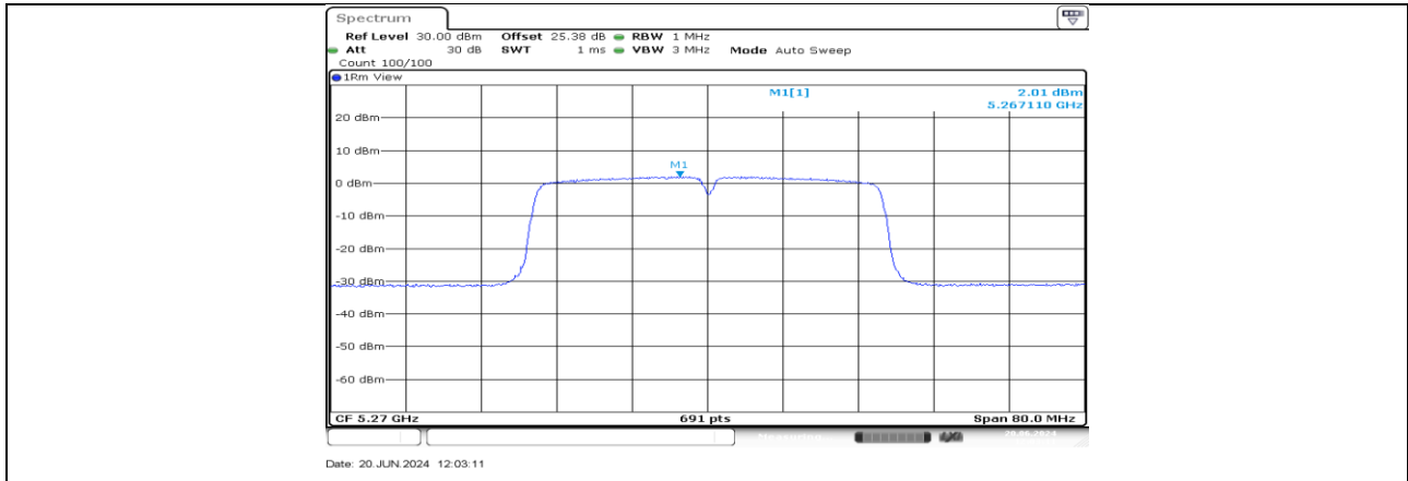
11AC40MIMO_Ant2_5270
