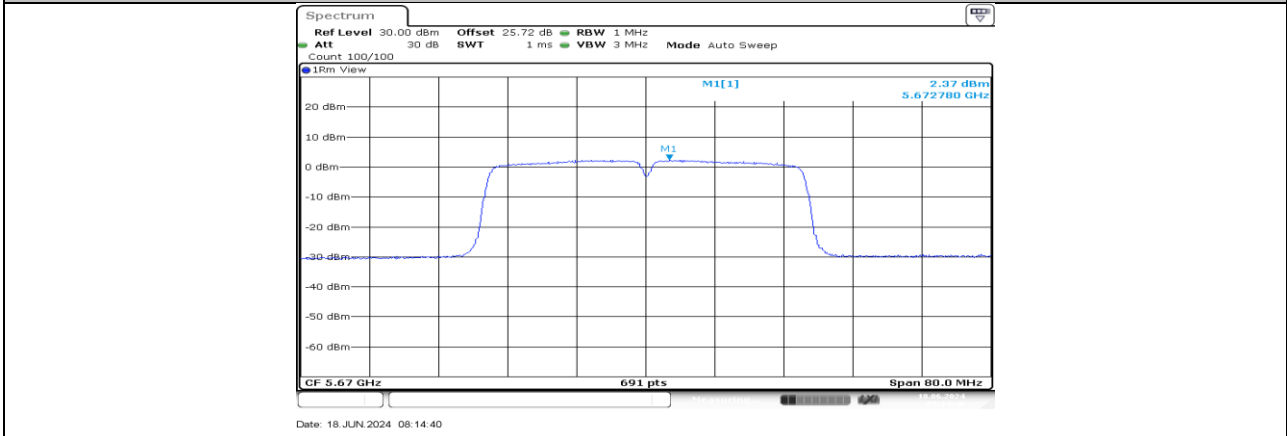
11AC40MIMO_Ant2_5670
