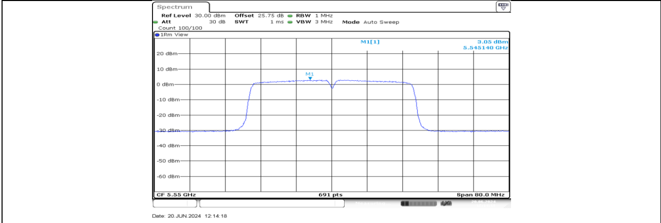
11AC40MIMO_Ant3_5550
