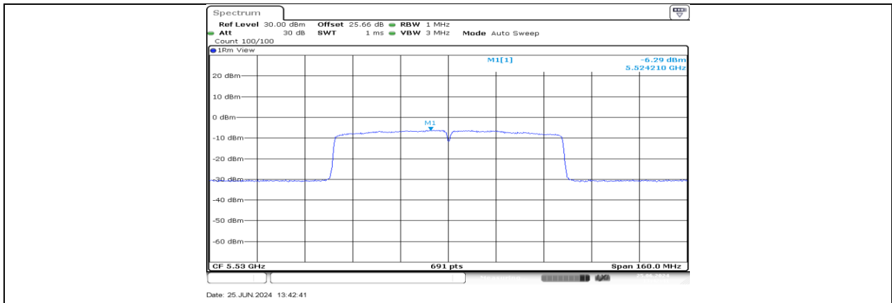
11AC80MIMO_Ant2_5530
