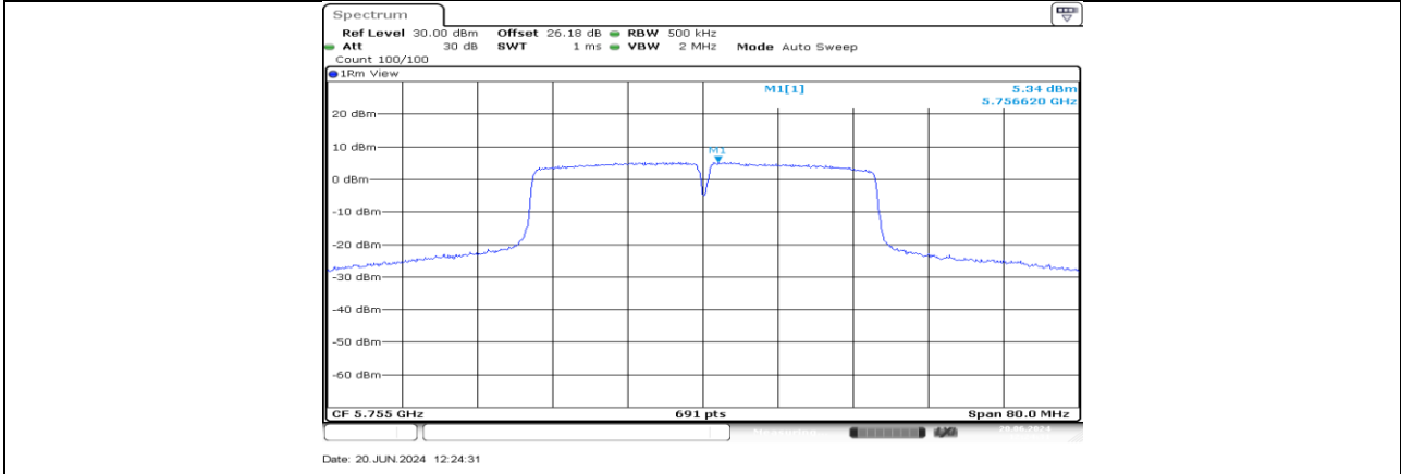
11AC40MIMO_Ant1_5755
