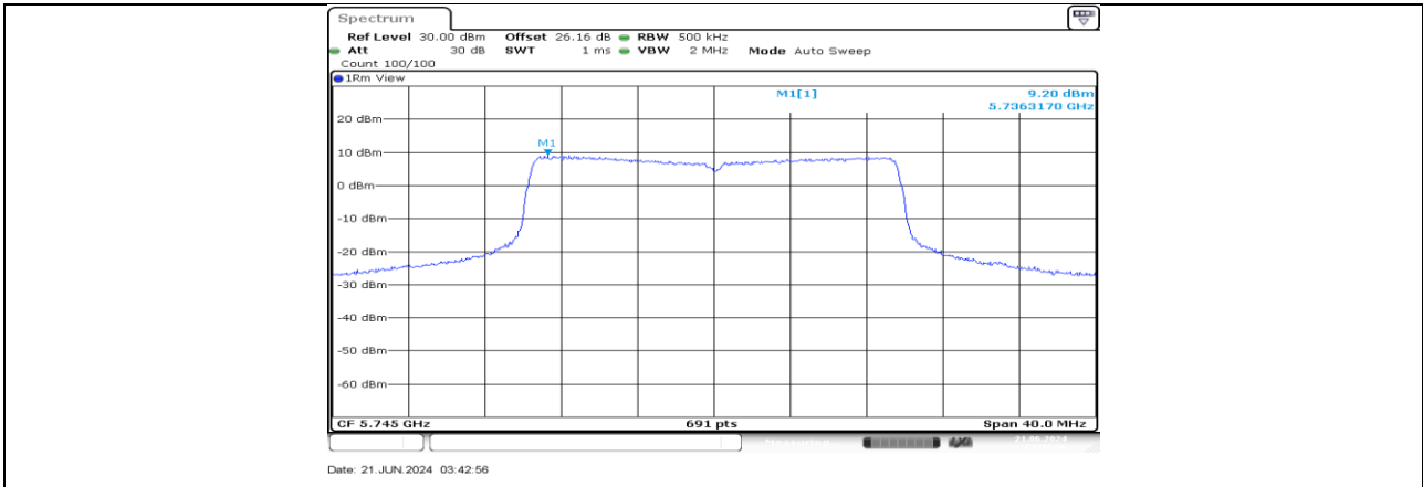
11AX20MIMO_Ant2_5745
