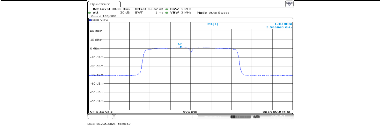
11AC40MIMO_Ant4_5510
