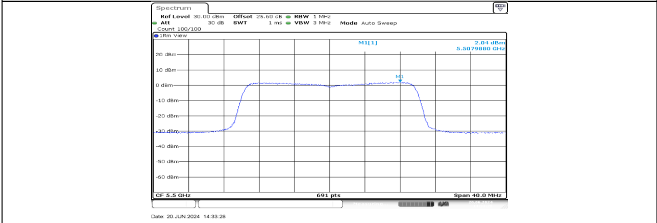
11AX20MIMO_Ant4_5500
