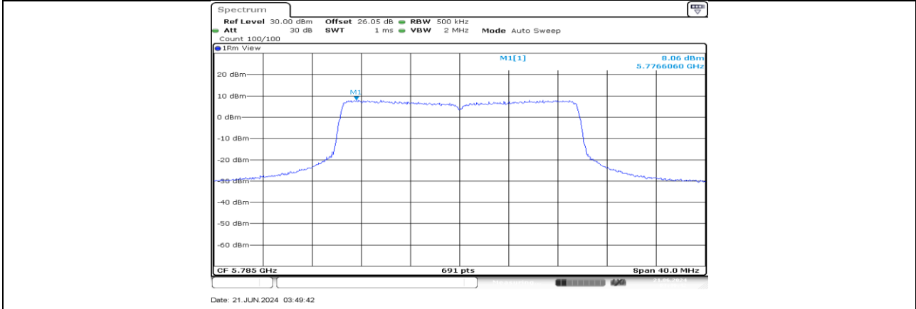
11AX20MIMO_Ant3_5785
