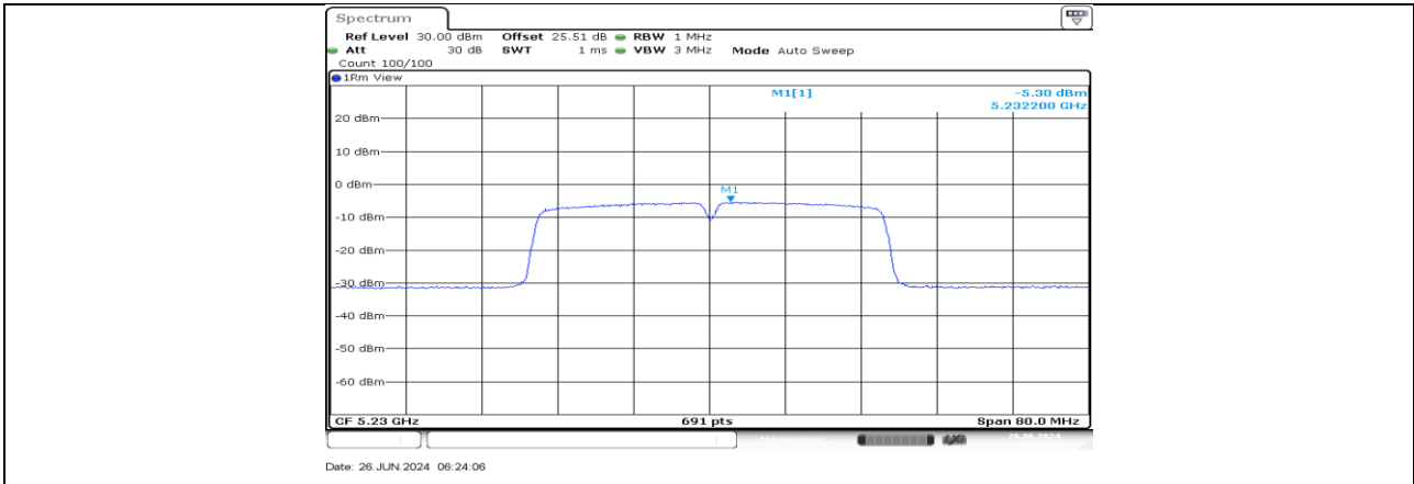
11AC40MIMO_Ant3_5230
