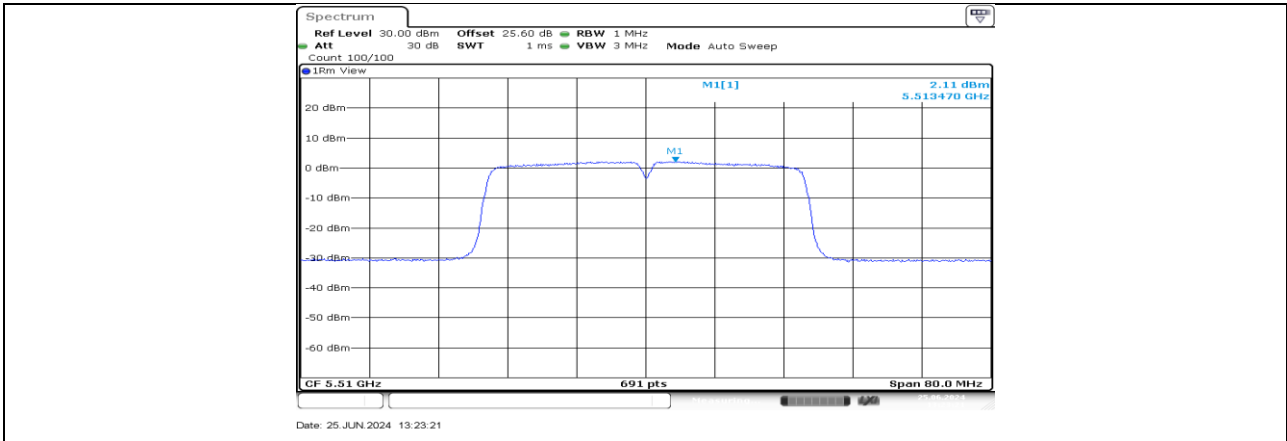
11AC40MIMO_Ant3_5510
