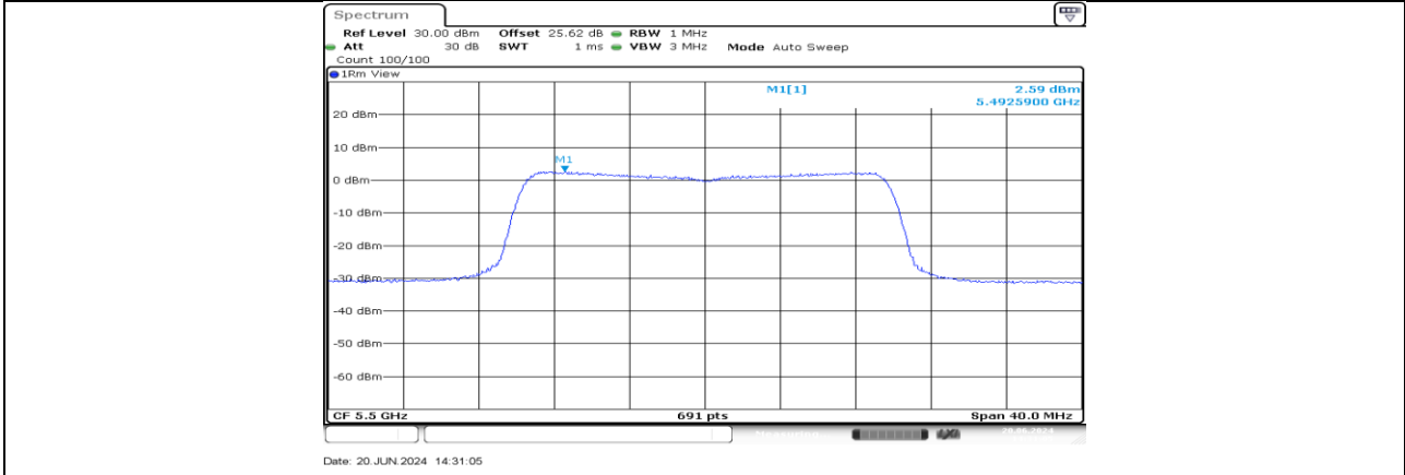
11AX20MIMO_Ant1_5500
