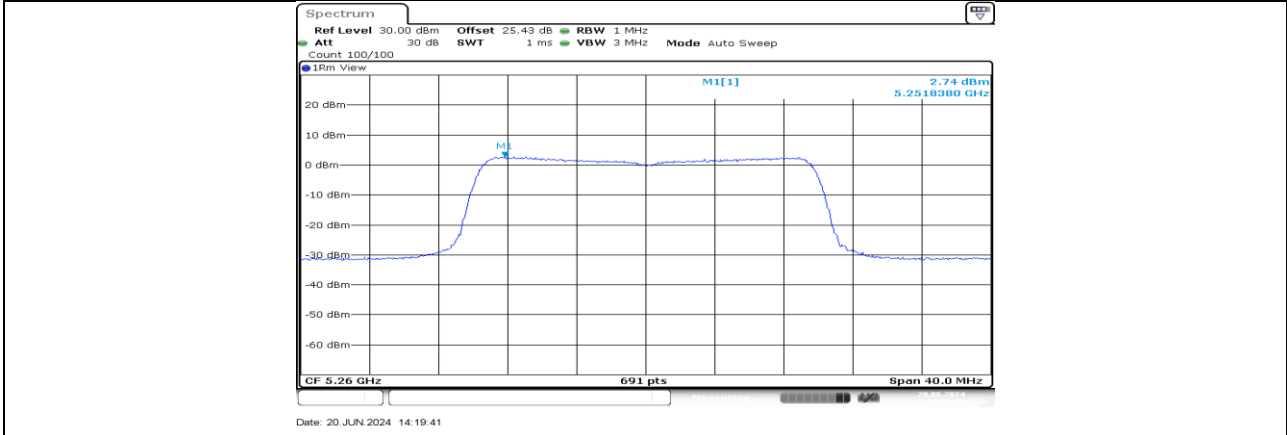
11AX20MIMO_Ant1_5260
