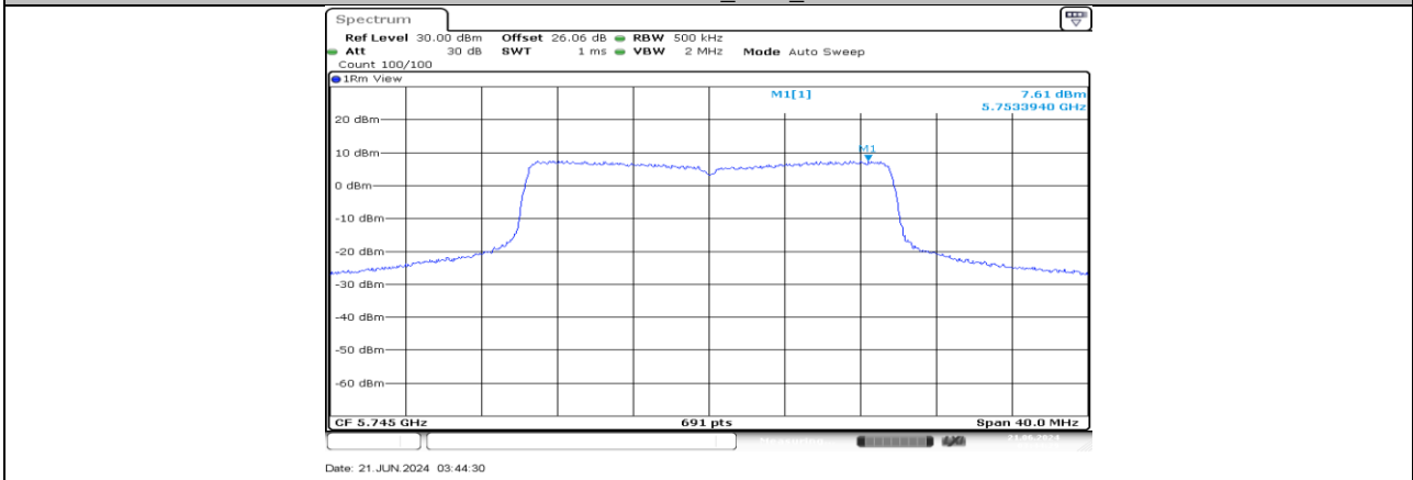
11AX20MIMO_Ant4_5745
