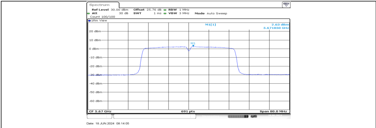
11AC40MIMO_Ant1_5670
