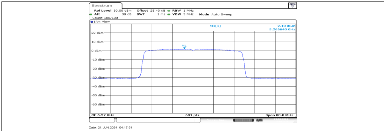
11AX40MIMO_Ant3_5270
