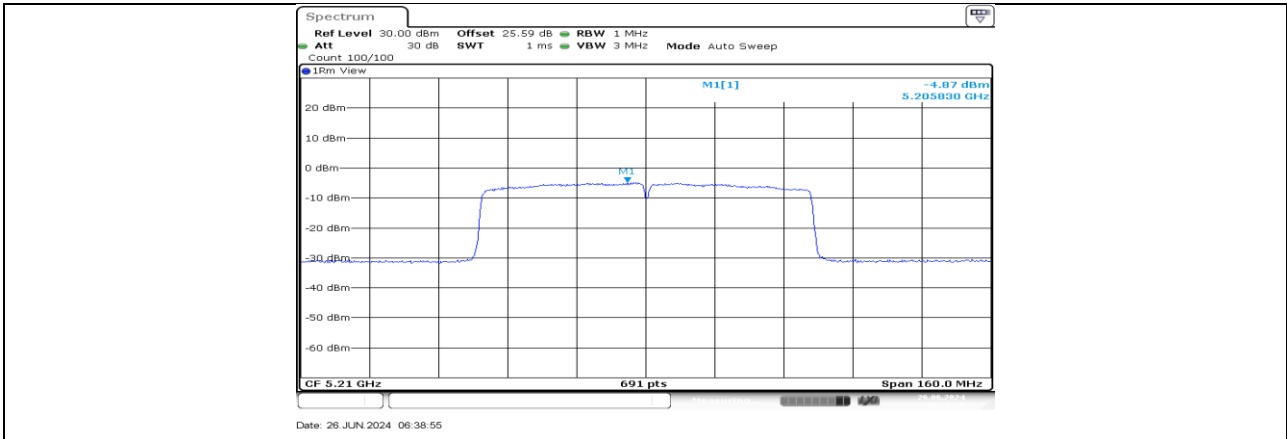
11AC80MIMO_Ant4_5210
