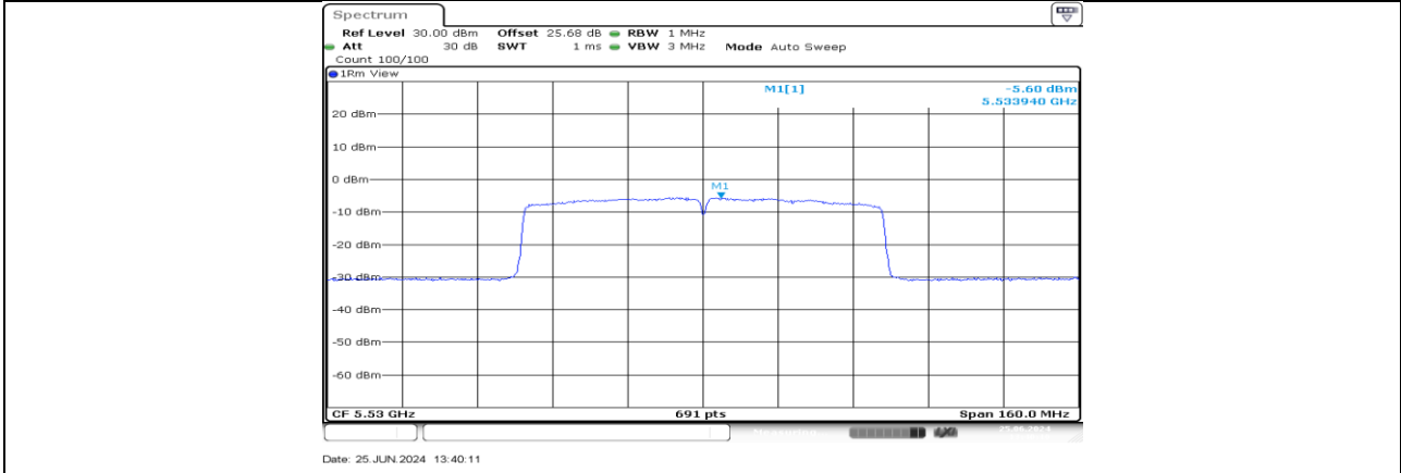
11AC80MIMO_Ant1_5530
