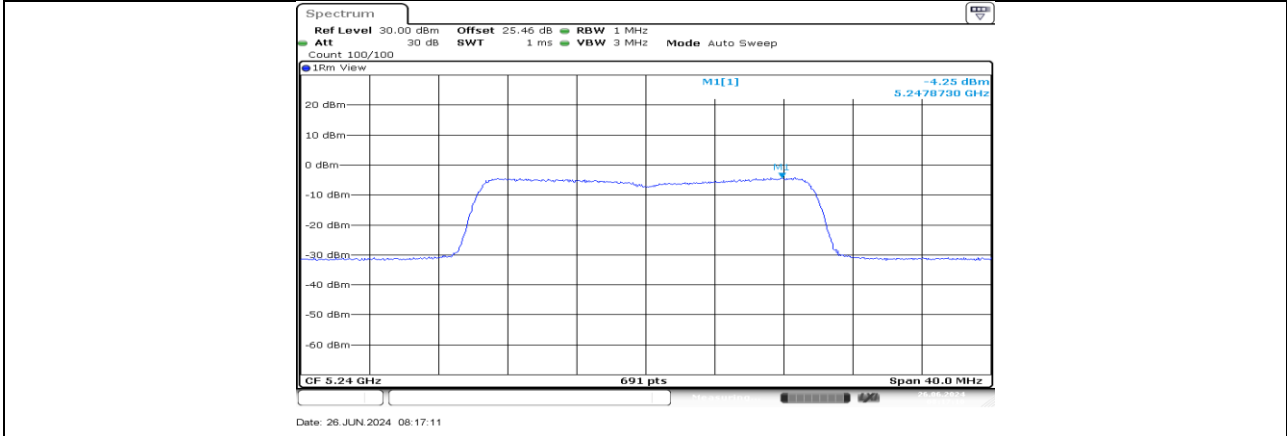
11AX20MIMO_Ant4_5240
