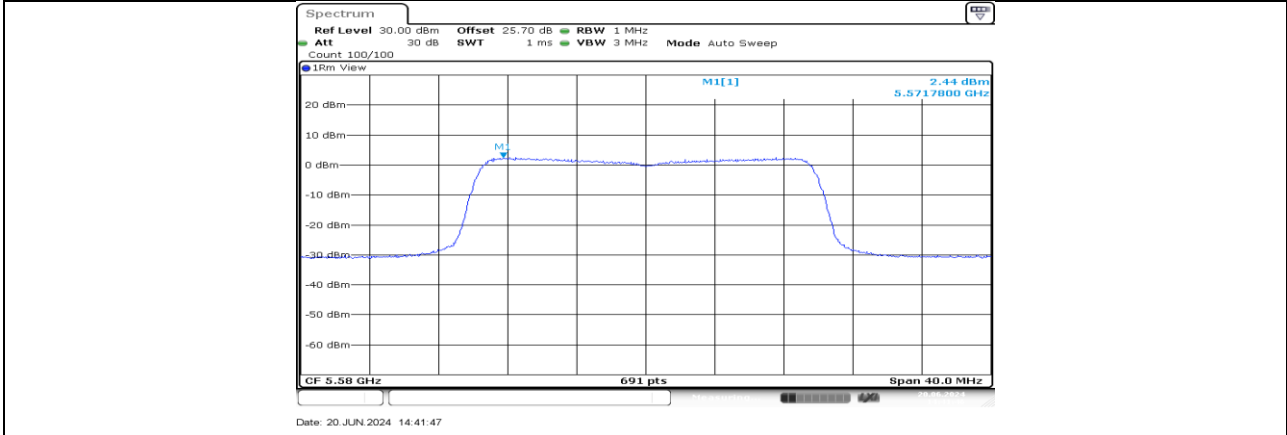
11AX20MIMO_Ant3_5580
