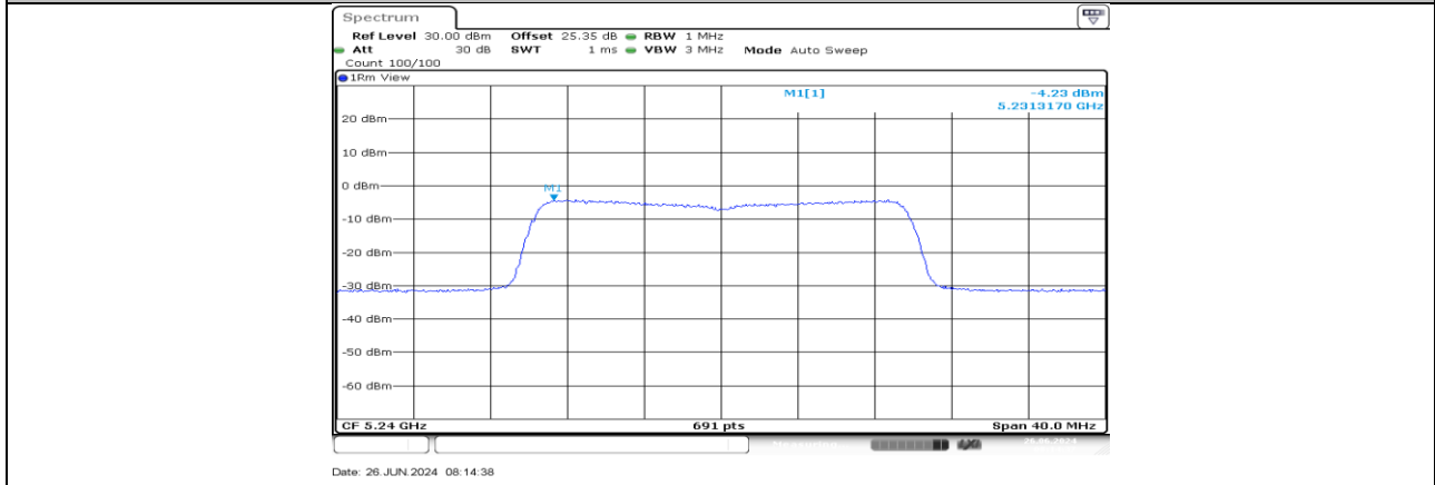
11AX20MIMO_Ant1_5240
