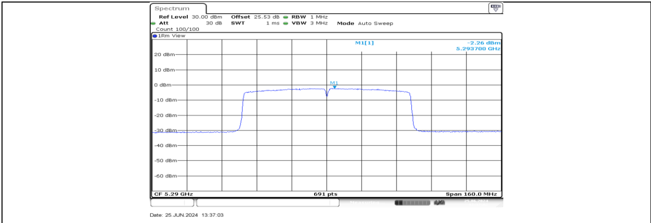
11AC80MIMO_Ant3_5290
