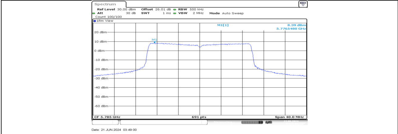
11AX20MIMO_Ant2_5785
