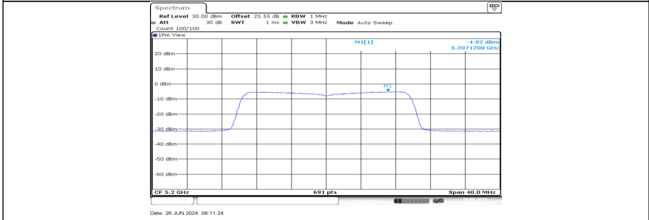
11AX20MIMO_Ant2_5200
