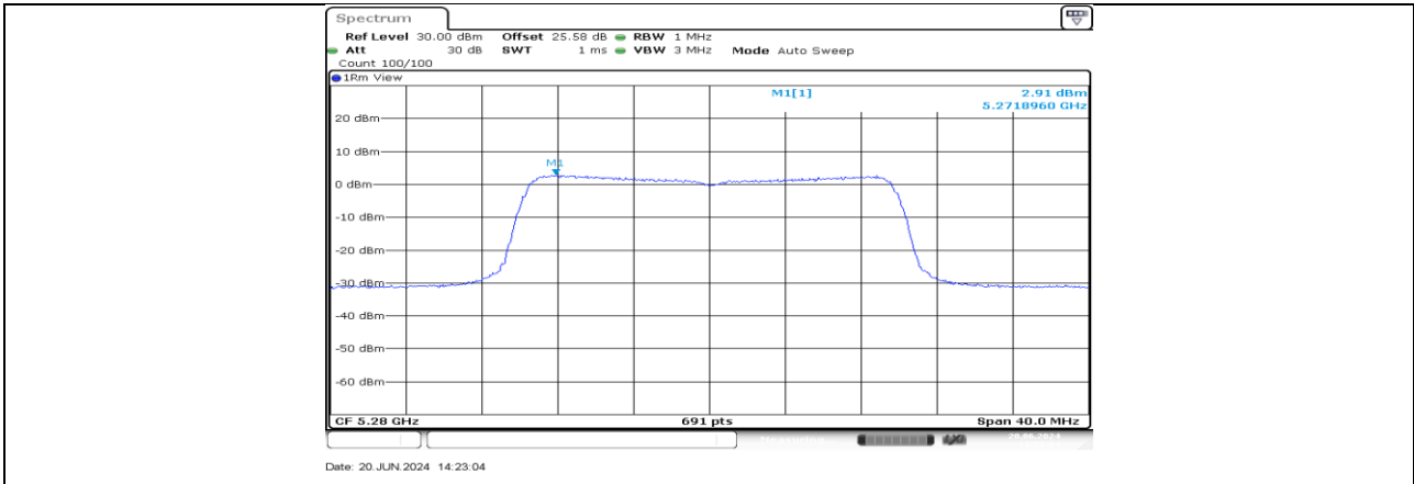
11AX20MIMO_Ant1_5280
