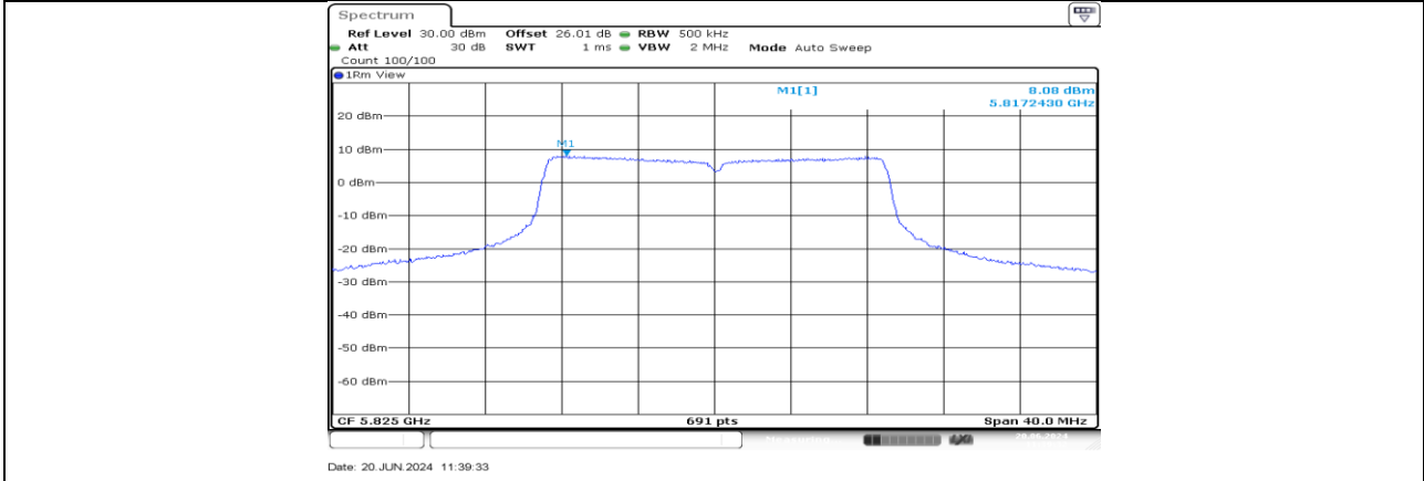
11AC20MIMO_Ant1_5825
