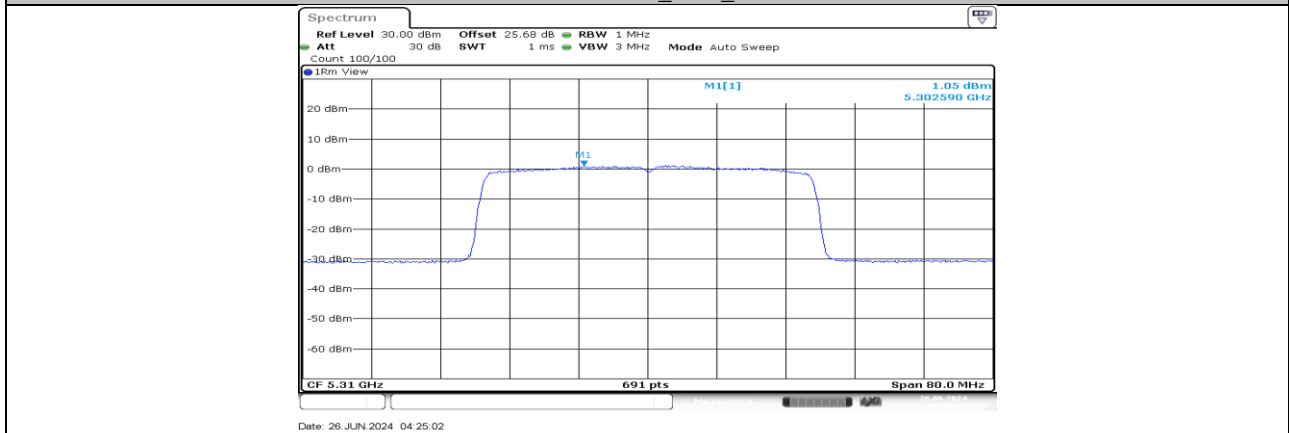
11AX40MIMO_Ant1_5310
