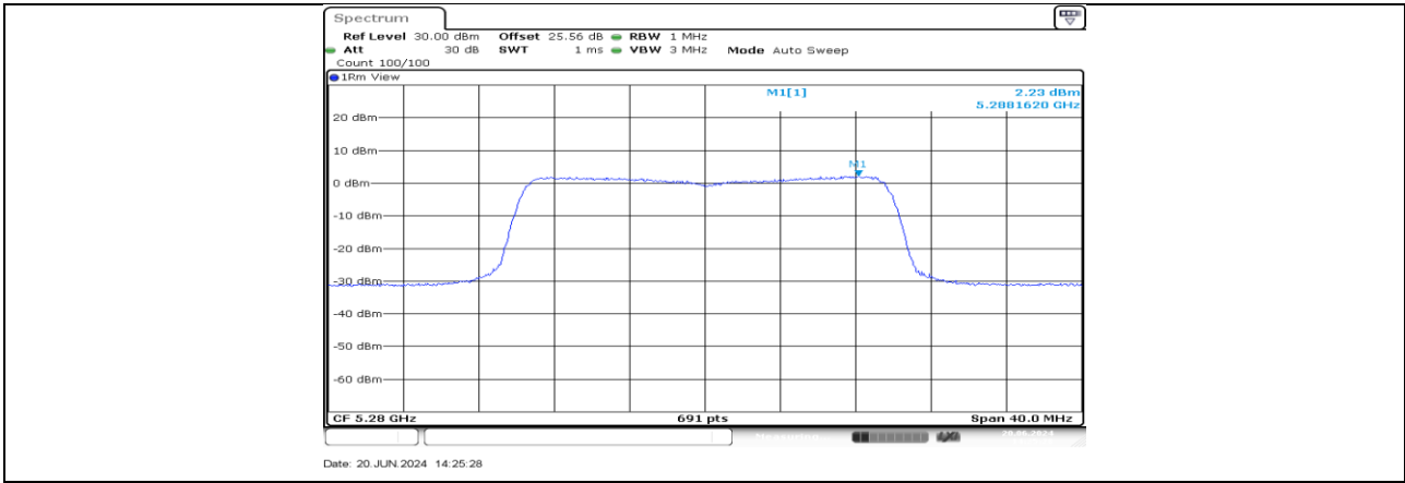
11AX20MIMO_Ant4_5280
