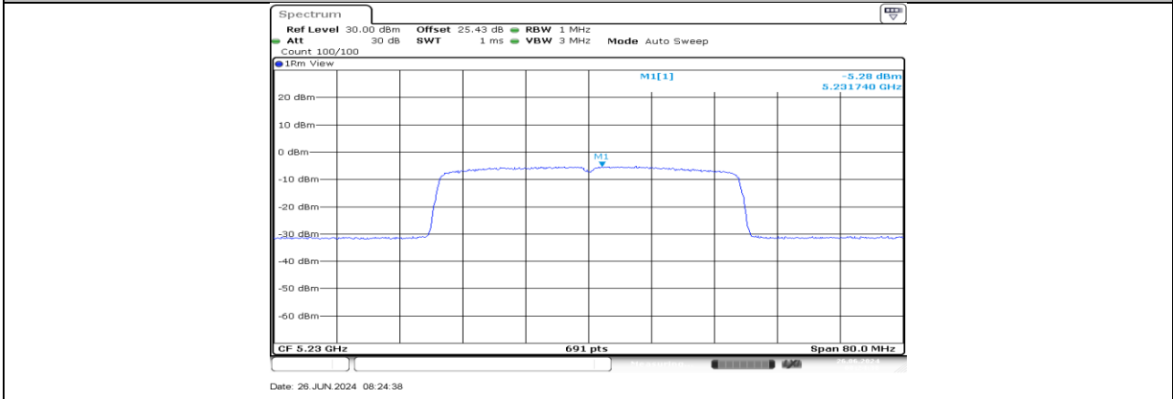
11AX40MIMO_Ant2_5230
