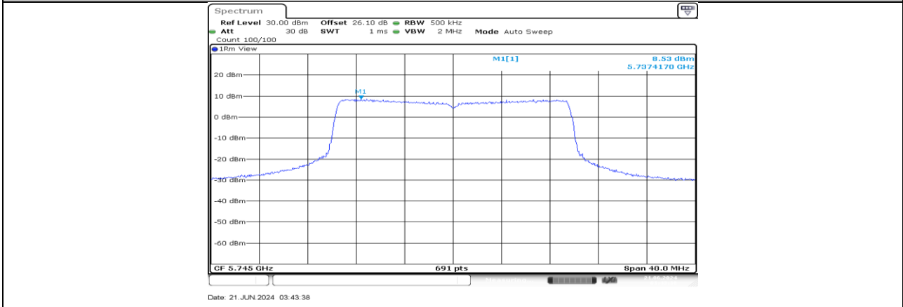
11AX20MIMO_Ant3_5745
