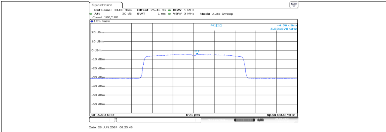
11AX40MIMO_Ant1_5230
