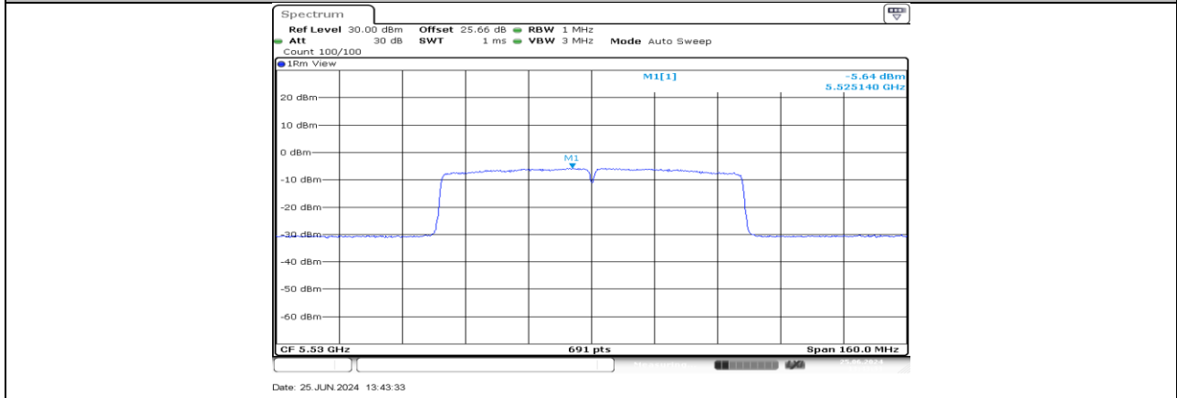
11AC80MIMO_Ant3_5530
