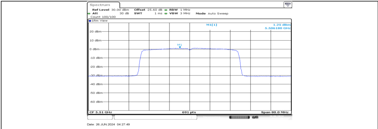
11AX40MIMO_Ant1_5510
