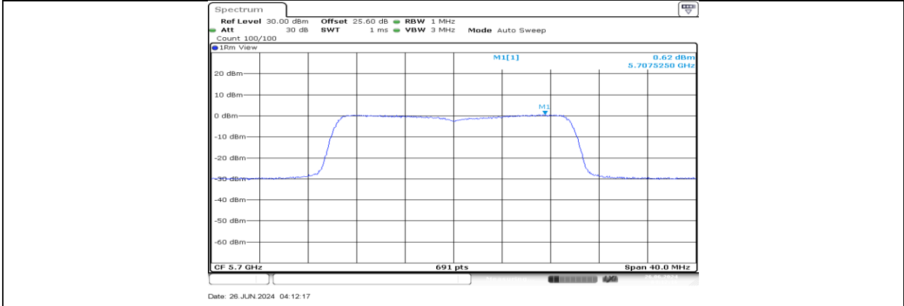
11AX20MIMO_Ant4_5700
