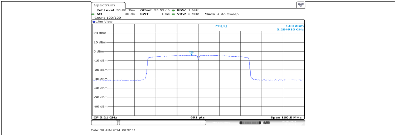
11AC80MIMO_Ant1_5210
