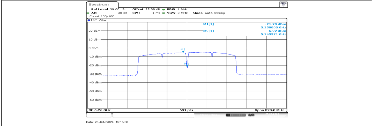
11AC160MIMO_Ant3_5250_UNII-1
