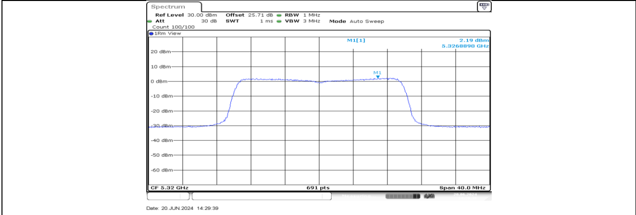
11AX20MIMO_Ant4_5320
