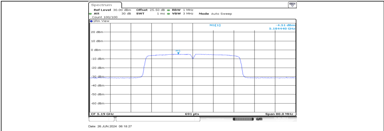
11AC40MIMO_Ant1_5190
