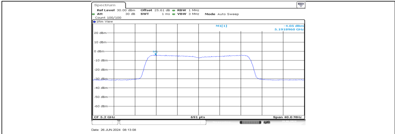
11AX20MIMO_Ant4_5200
