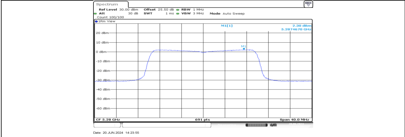
11AX20MIMO_Ant2_5280
