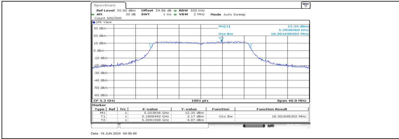
11AC20MIMO_Ant3_5200
