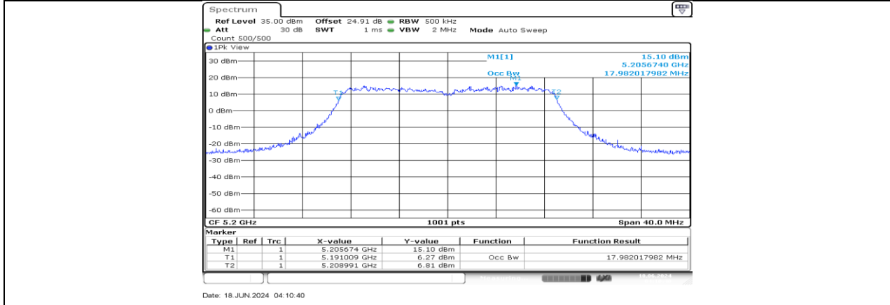
11AC20MIMO_Ant4_5200
