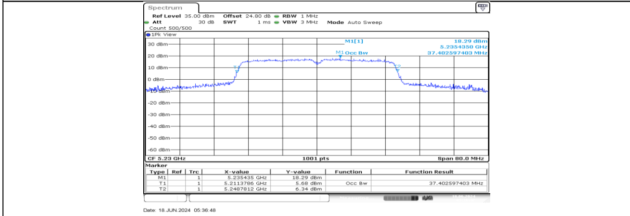
11AC40MIMO_Ant4_5230
