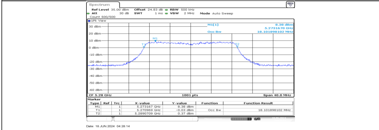
11AC20MIMO_Ant2_5280
