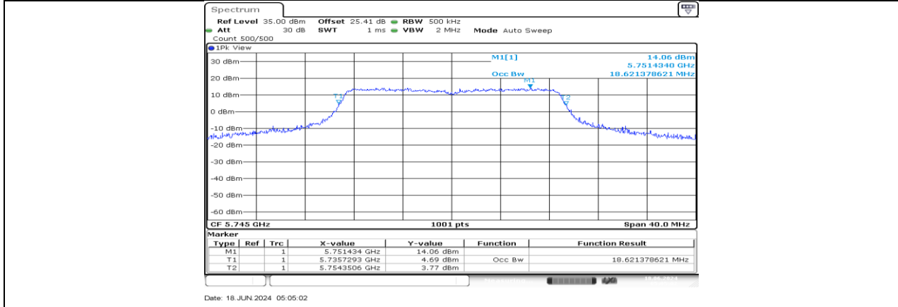
11AC20MIMO_Ant3_5745
