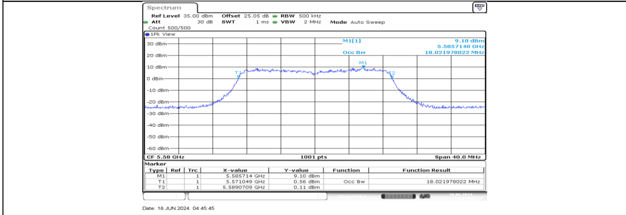
11AC20MIMO_Ant4_5580
