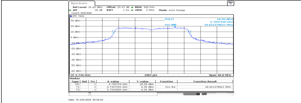
11AC20MIMO_Ant2_5745
