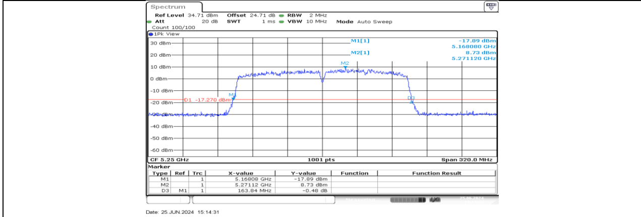
11AC160MIMO_Ant3_5250
