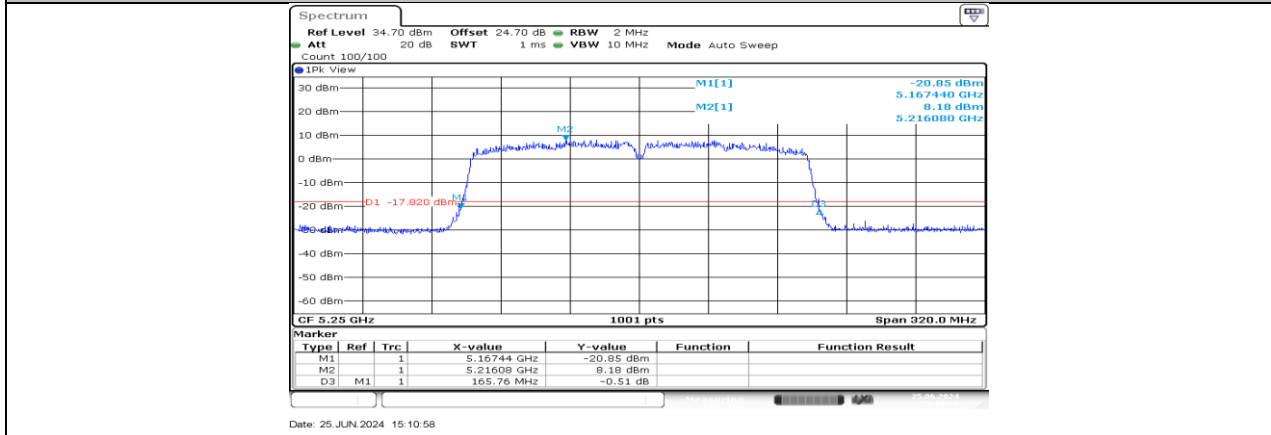
11AC160MIMO_Ant1_5250
