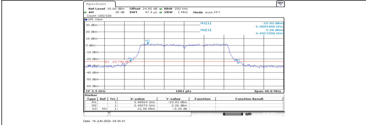
11AC20MIMO_Ant2_5500
