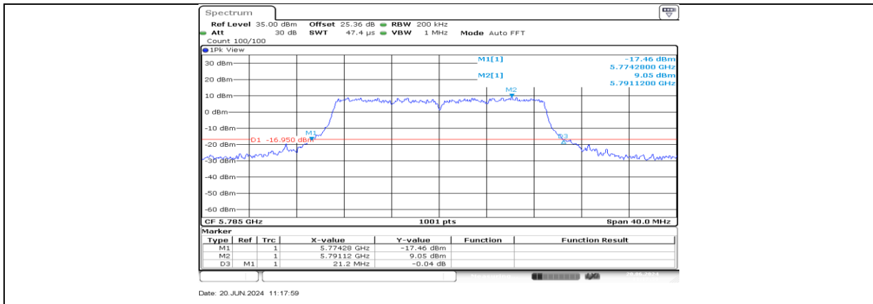
11AC20MIMO_Ant3_5785
