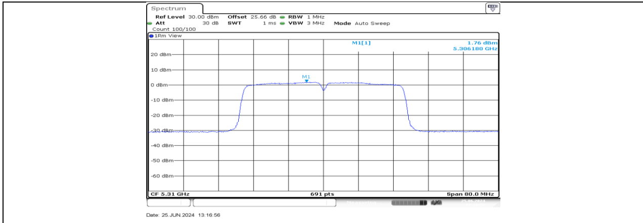
11AC40MIMO_Ant4_5310
