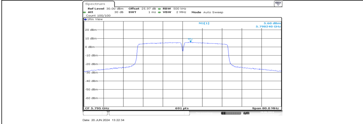
11AC40MIMO_Ant3_5795
