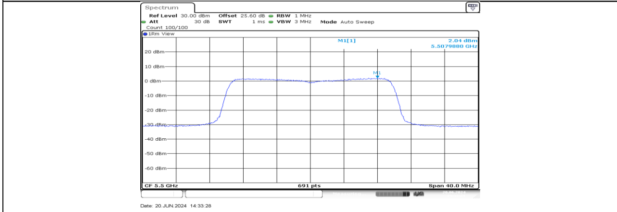
11AX20MIMO_Ant4_5500
