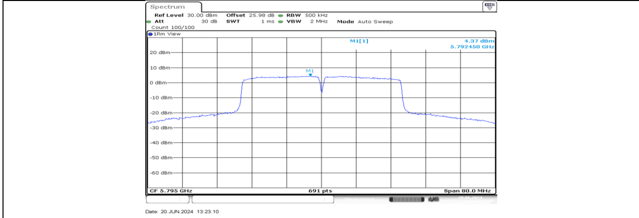
11AC40MIMO_Ant4_5795
