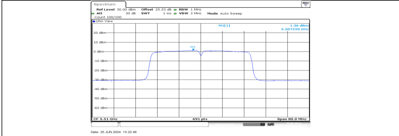
11AC40MIMO_Ant2_5510
