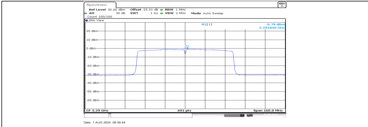
11AC80MIMO_Ant3_5290
