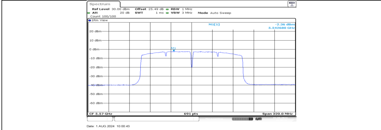
11AC160MIMO_Ant2_5570
