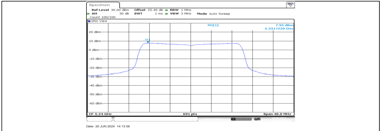
11AX20MIMO_Ant3_5240
