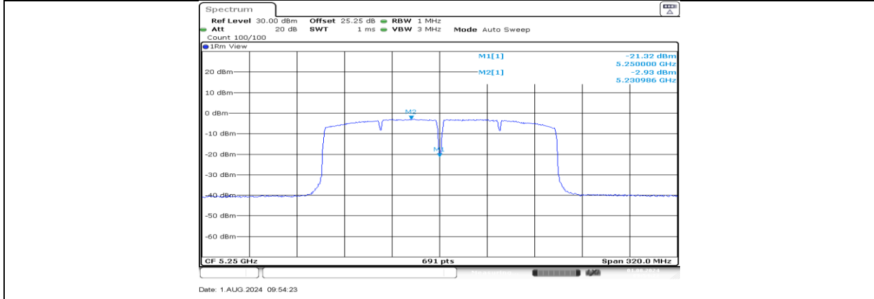
11AC160MIMO_Ant3_5250_UNII-1
