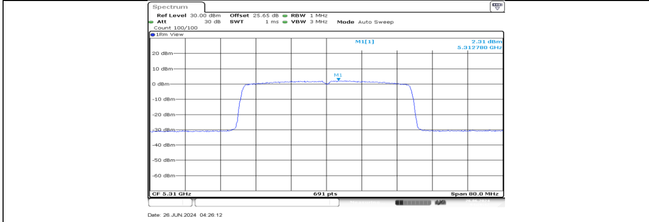
11AX40MIMO_Ant3_5310
