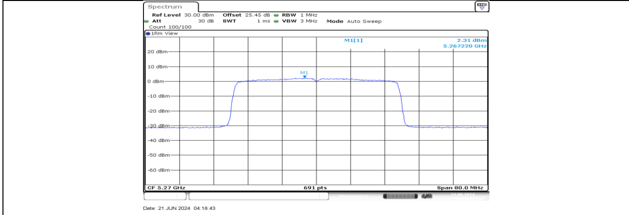
11AX40MIMO_Ant4_5270
