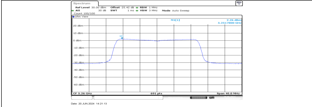
11AX20MIMO_Ant3_5260
