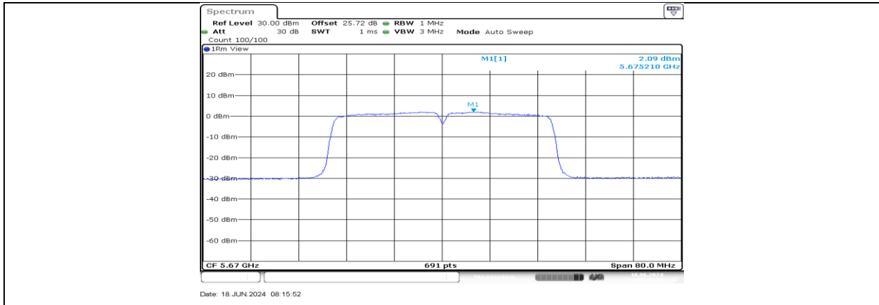
11AC40MIMO_Ant4_5670
