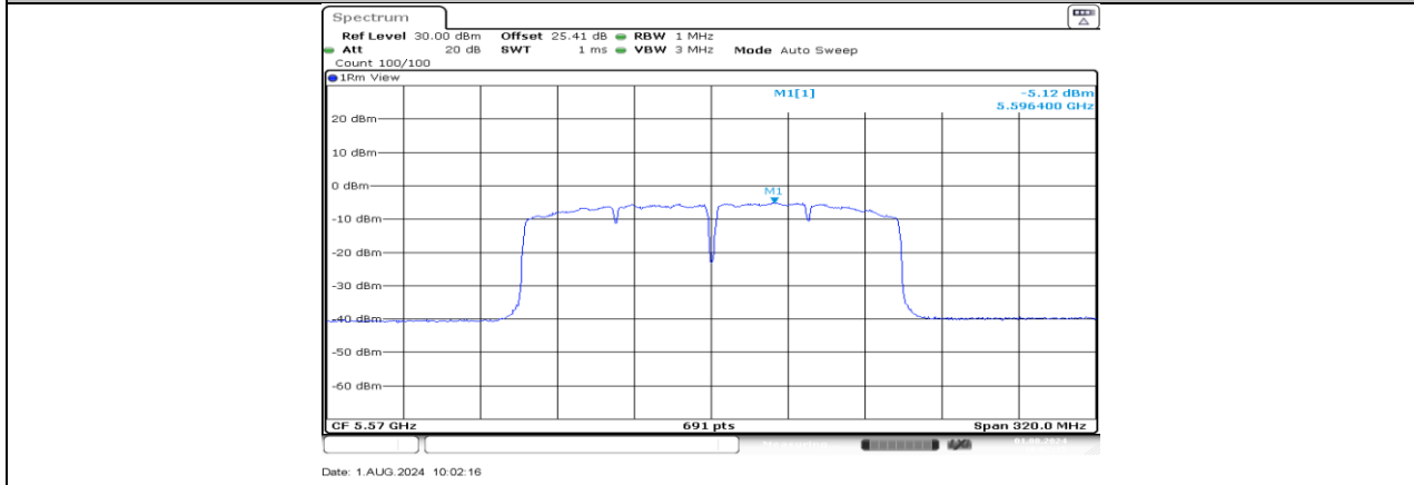
11AC160MIMO_Ant4_5570
