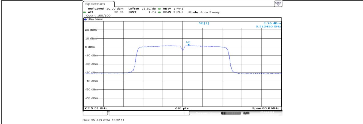
11AC40MIMO_Ant1_5510
