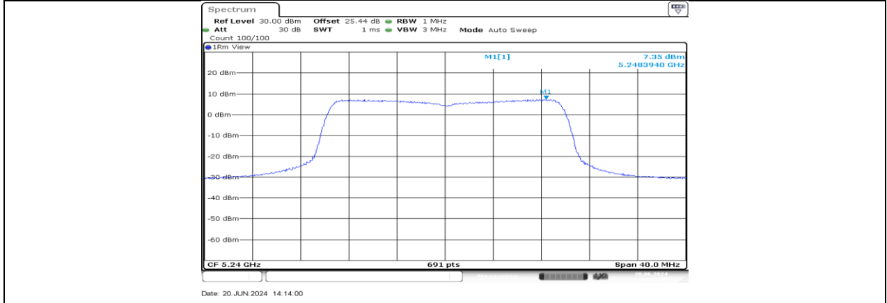
11AX20MIMO_Ant4_5240
