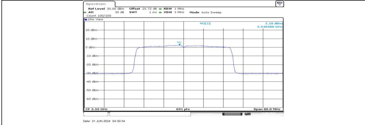
11AX40MIMO_Ant4_5550
