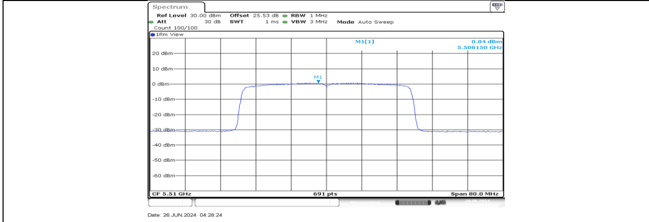
11AX40MIMO_Ant2_5510
