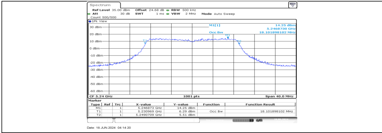
11AC20MIMO_Ant2_5240
