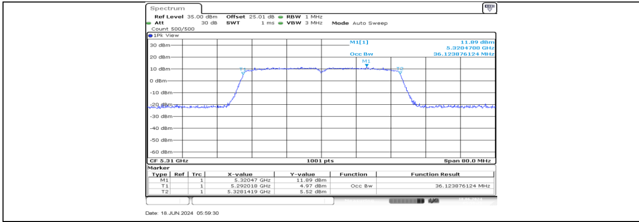
11AC40MIMO_Ant1_5310
