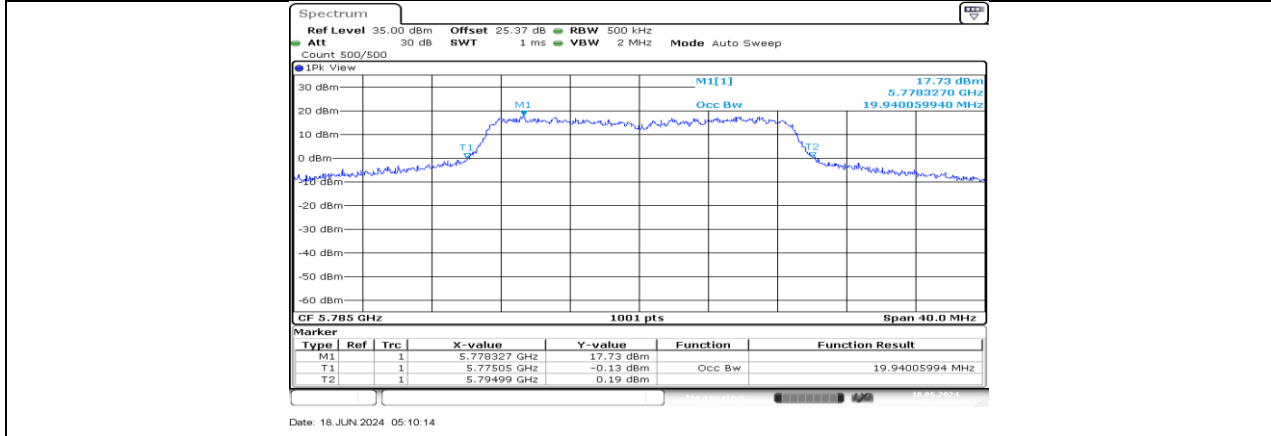
11AC20MIMO_Ant4_5785
