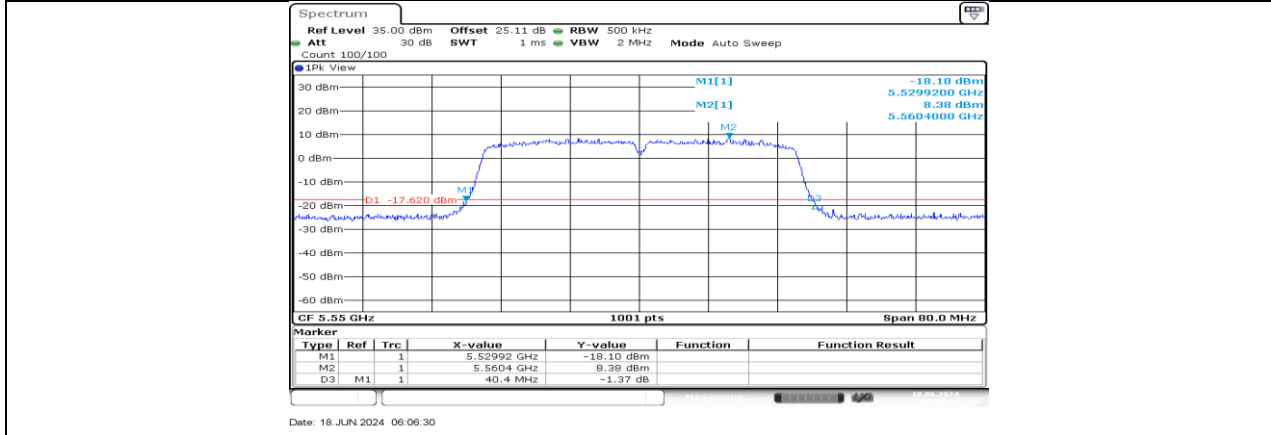
11AC40MIMO_Ant1_5550
