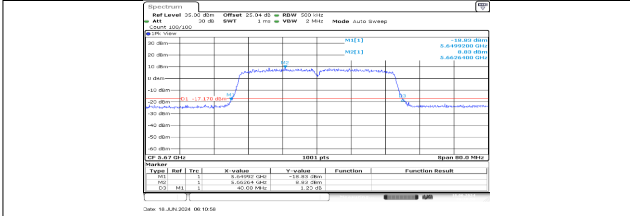
11AC40MIMO_Ant2_5670
