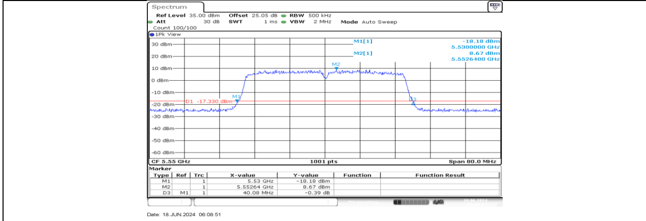
11AC40MIMO_Ant4_5550
