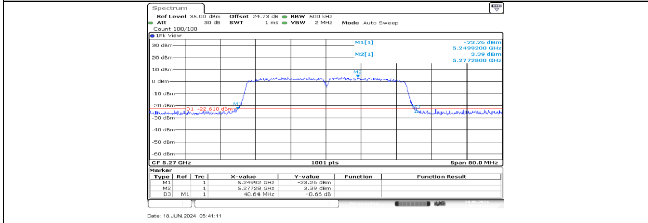
11AC40MIMO_Ant3_5270
