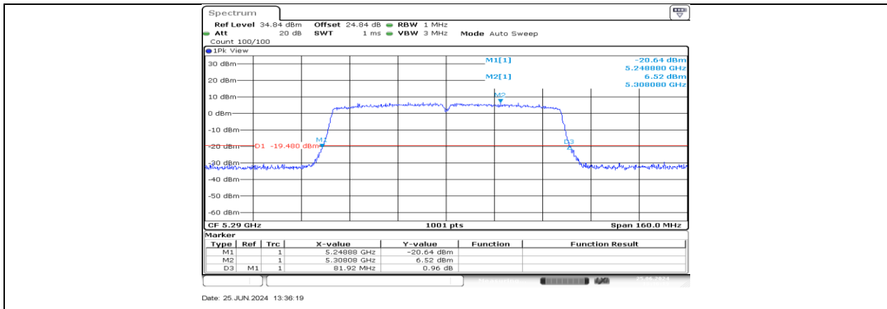
11AC80MIMO_Ant3_5290
