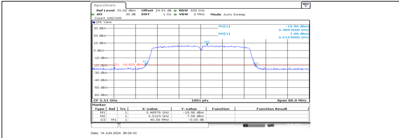
11AC40MIMO_Ant3_5510
