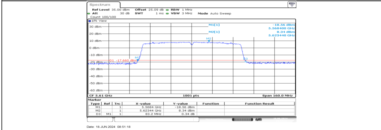
11AC80MIMO_Ant3_5610
