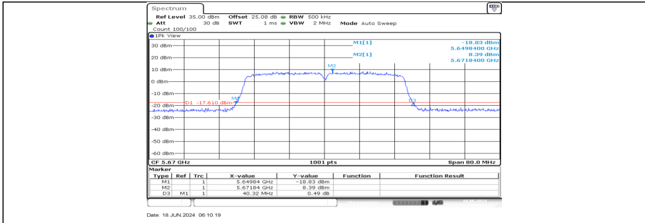
11AC40MIMO_Ant1_5670
