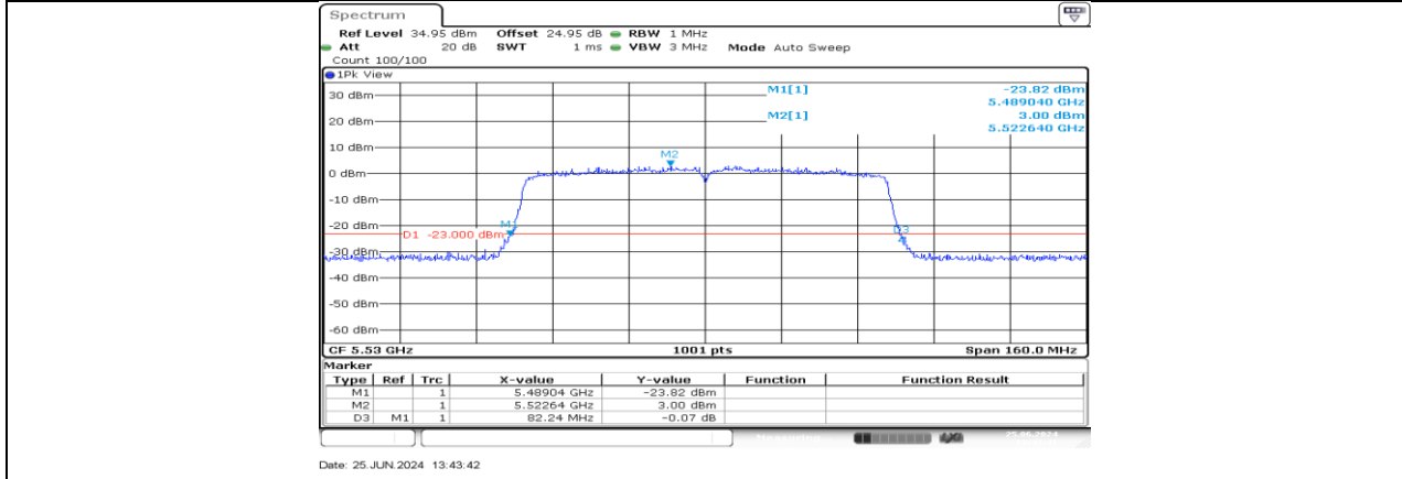
11AC80MIMO_Ant4_5530
