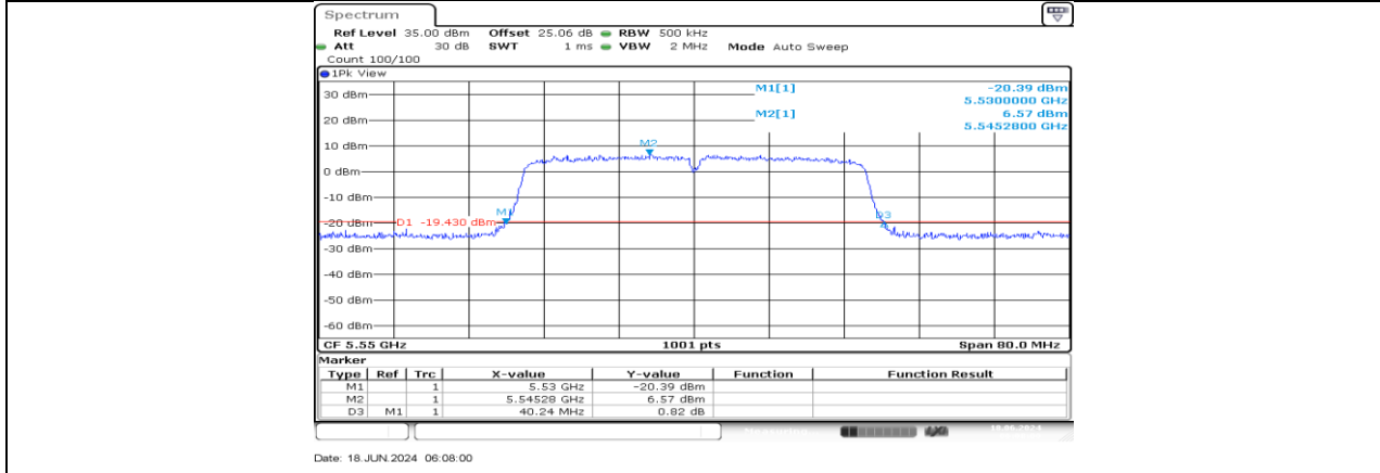
11AC40MIMO_Ant3_5550
