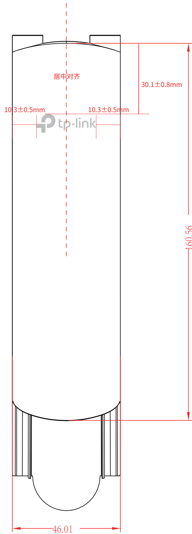
尺寸图
