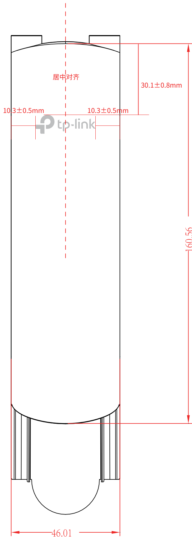
尺寸图
