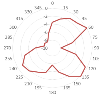
2450MHz_theta=90°
