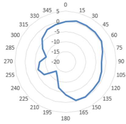
2450MHz_theta=90
