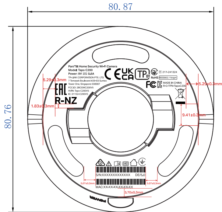
尺寸图
