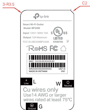
尺寸图 (54.00*29.00 ±0.2mm)
