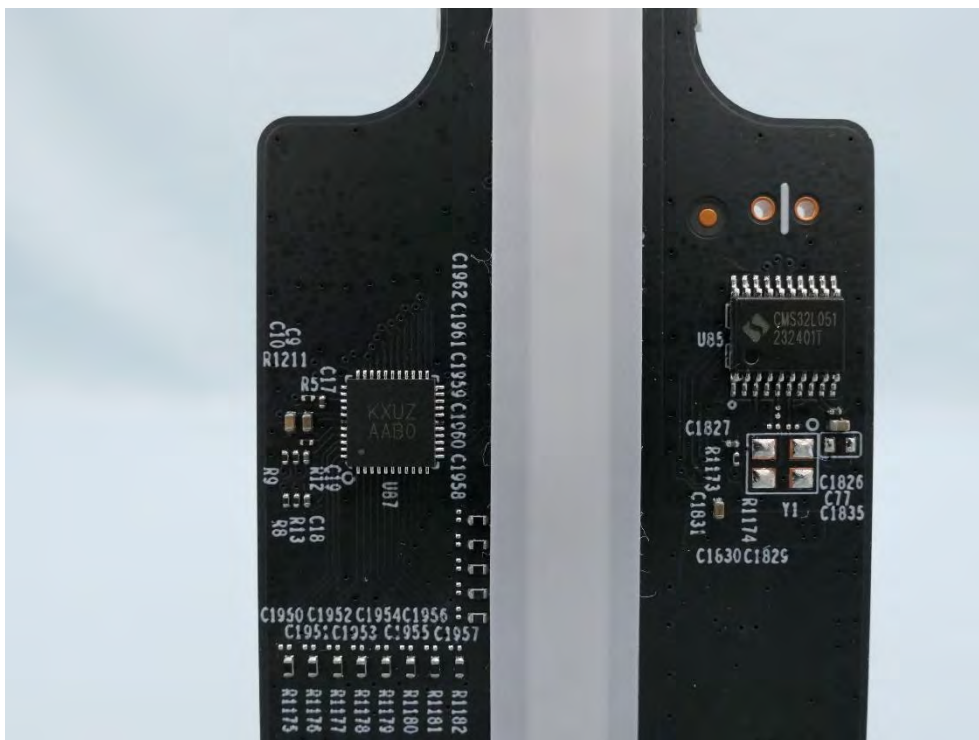
(28) EUT Photo – Archer BE700
