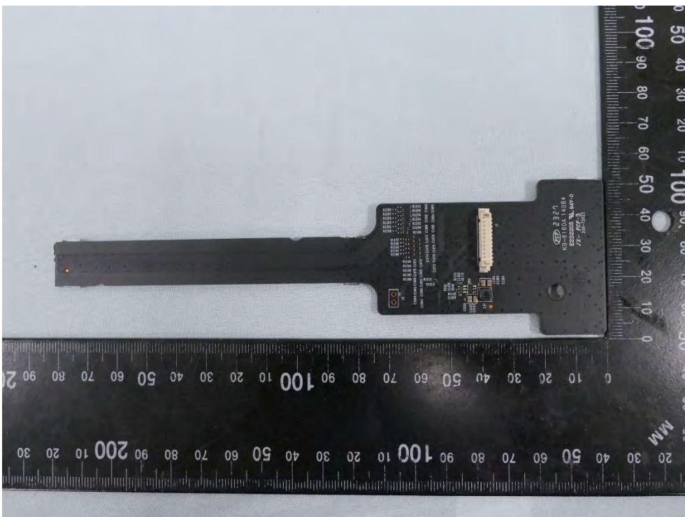
(58) EUT Photo – Archer BE700 Pro
