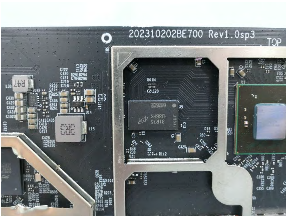
(16) EUT Photo – Archer BE700
