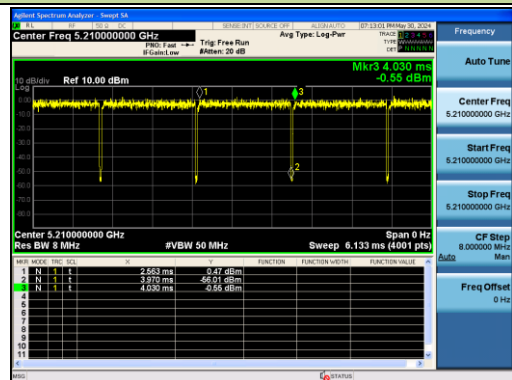
802.11ax-HE20
