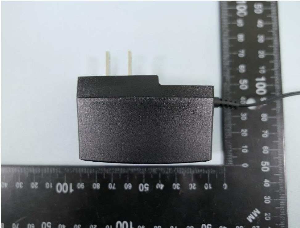
(9) EUT Photo
