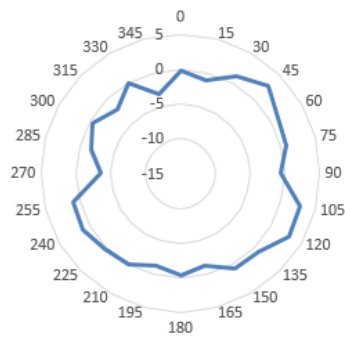
5250MHz-theta90
