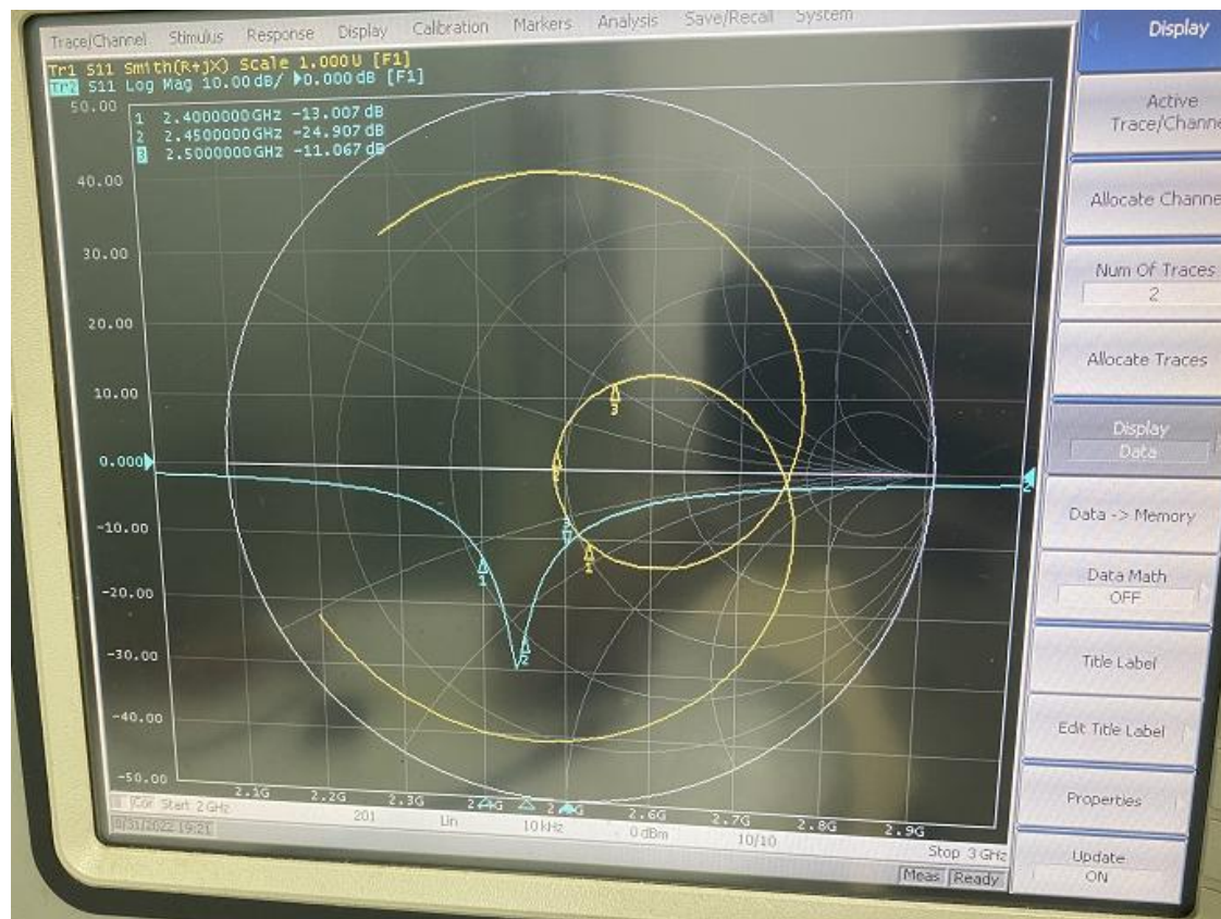
无源S11—(BT ANT)
