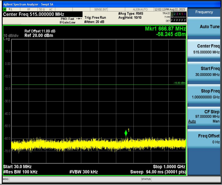
BLE_2M-Ant1-2402-30~1000-PASS
