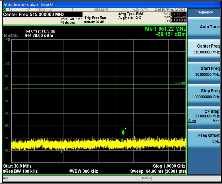
BLE_2M-Ant1-2440-30~1000-PASS
