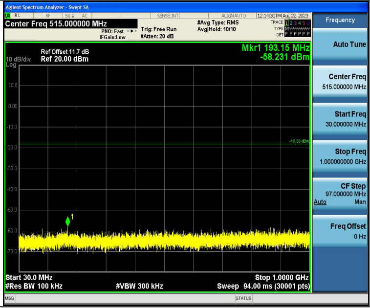
BLE_2M-Ant1-2480-30~1000-PASS
