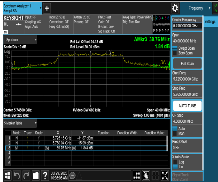
11A-CDD_Ant2_5745
