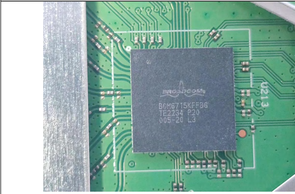
EUT Photo
