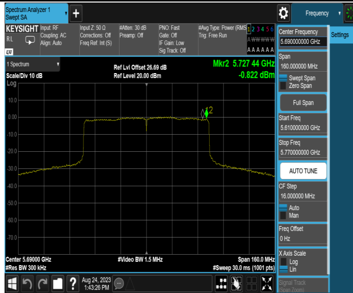
11AX80MIMO_Ant2_5690_UNII-3
