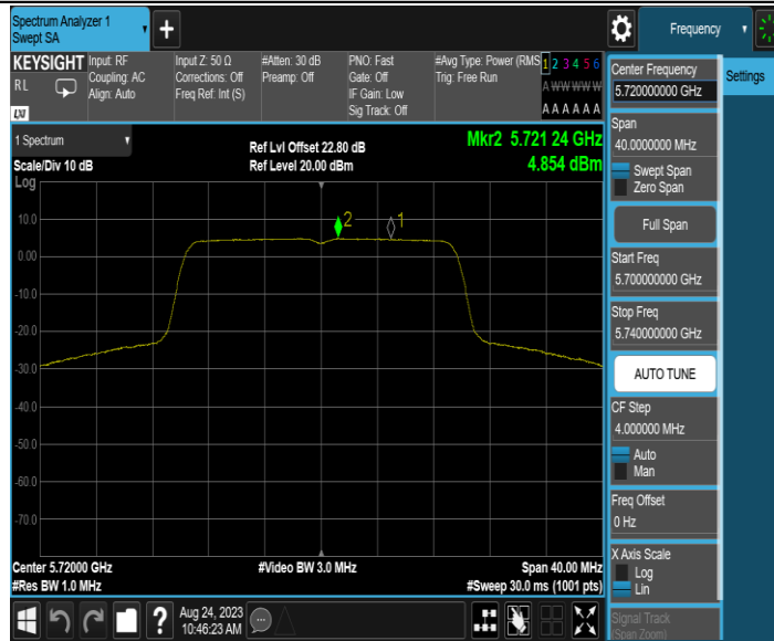
11AX20MIMO_Ant1_5720_UNII-3
