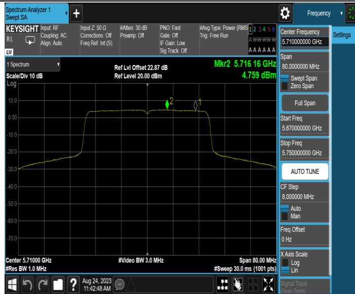
11AX40MIMO_Ant1_5710_UNII-3
