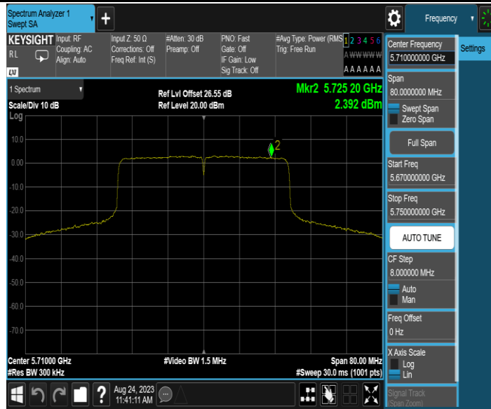
11AX40MIMO_Ant2_5710_UNII-3
