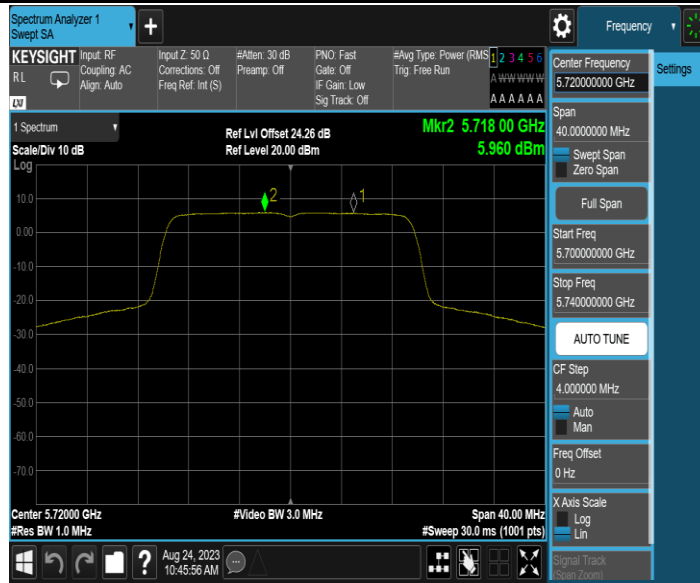
11AX20MIMO_Ant2_5720_UNII-2C
