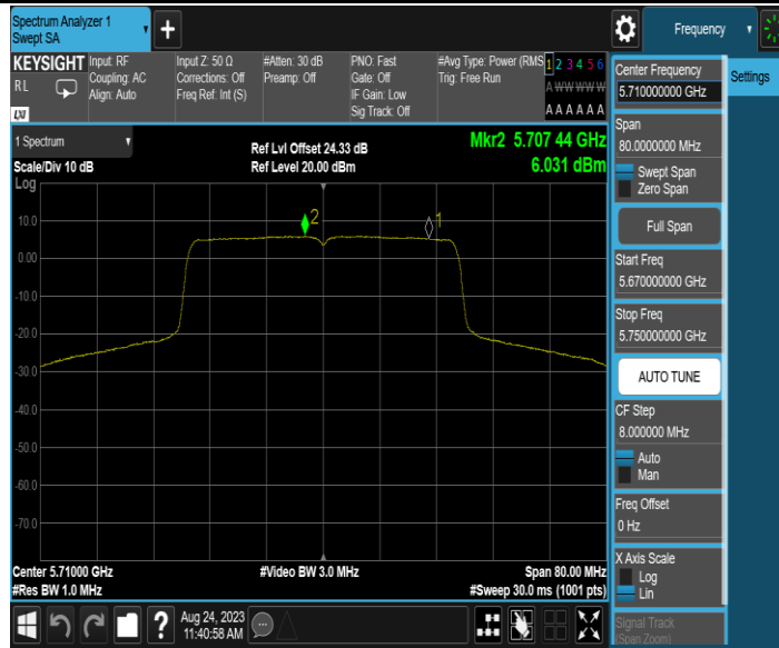
11AX40MIMO_Ant2_5710_UNII-2C
