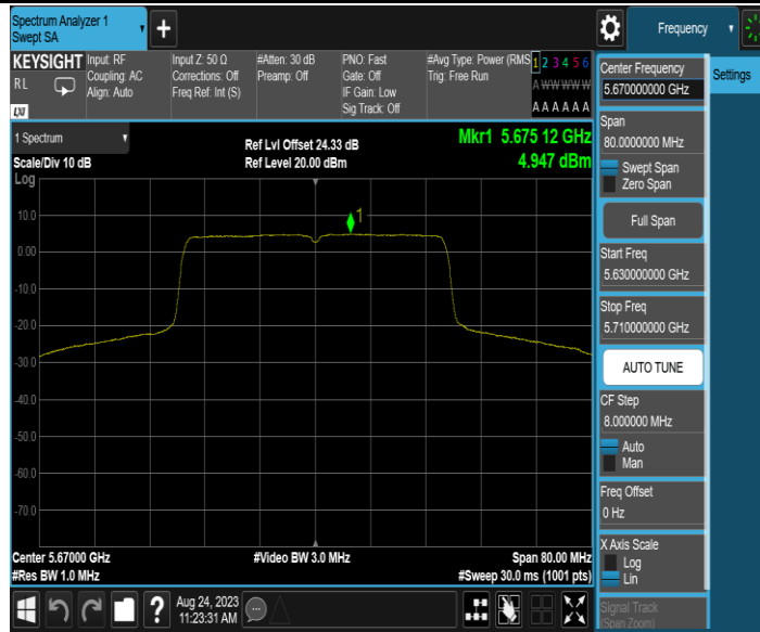
11AX40MIMO_Ant2_5670
