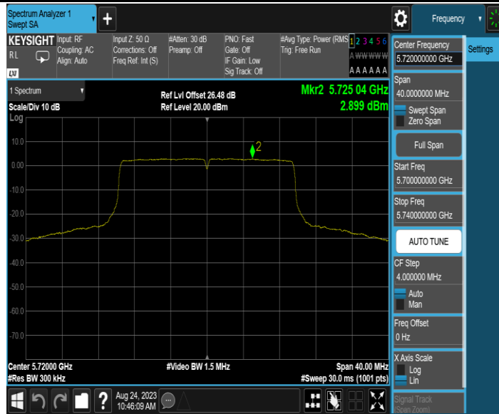
11AX20MIMO_Ant2_5720_UHII-3
