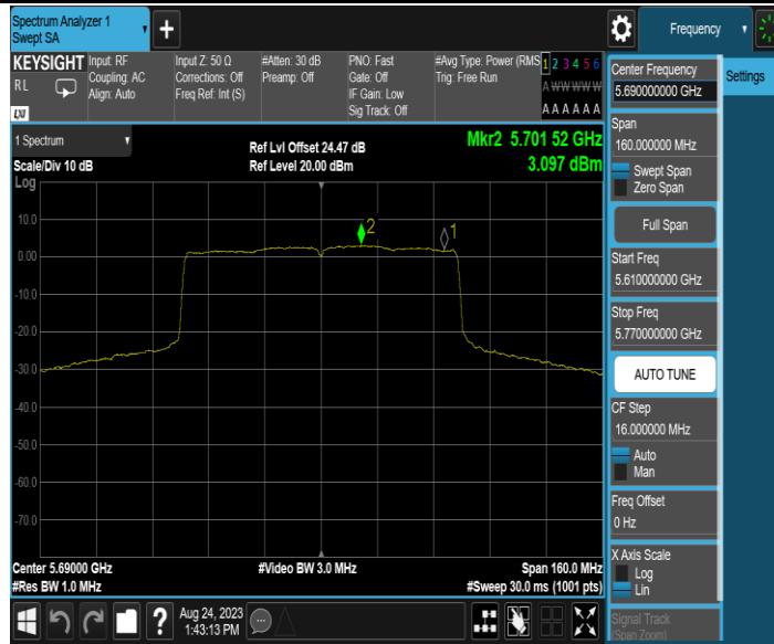
11AX80MIMO_Ant2_5690_UNII-2C
