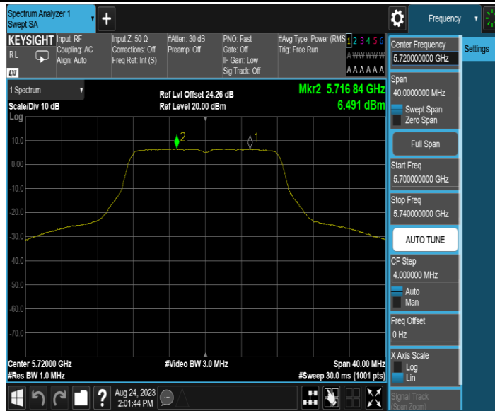
11A_Ant2_5720_UNII-2C
