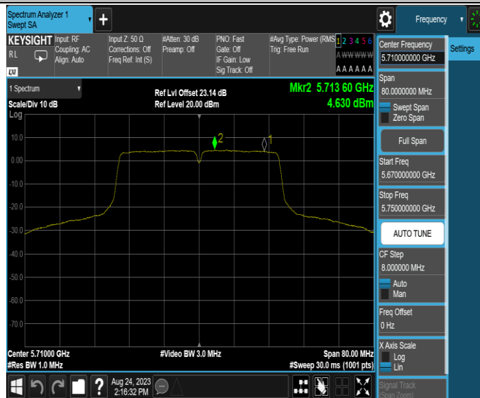
11N40MIMO_Ant1_5710_UNII-3
