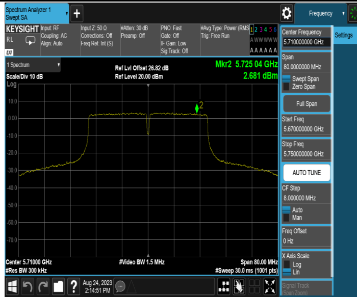
11N40MIMO_Ant2_5710_UNII-3
