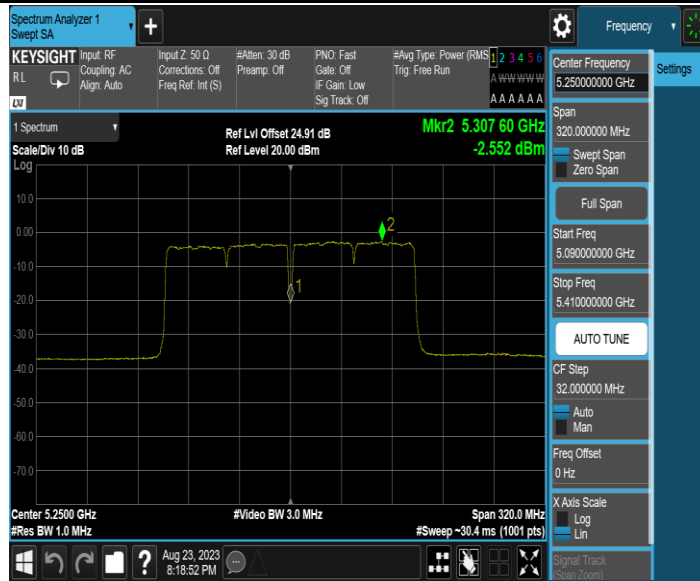
11AC160MIMO_Ant2_5250_UNII-2A
