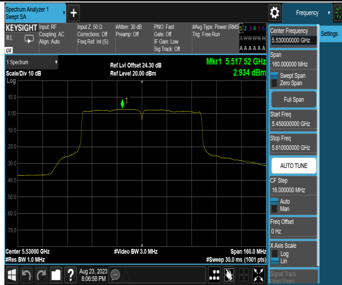
11AC80MIMO_Ant2_5530
