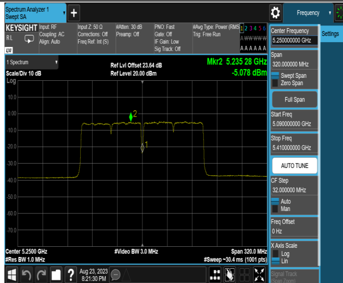
11AC160MIMO_Ant1_5250_UNII-2A
