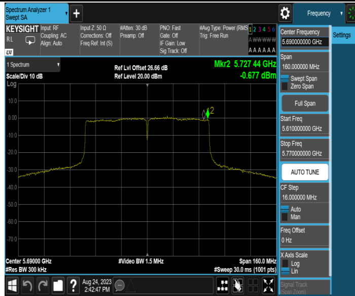
11AC80MIMO_Ant2_5690_U11-3
