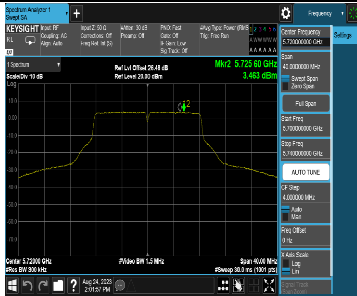
11A_Ant2_5720_UNII-3
