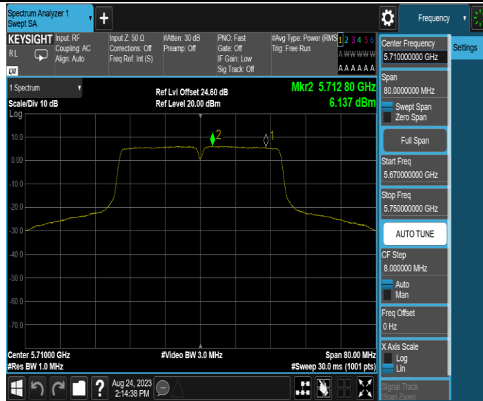
11N40MIMO_Ant2_5710_UNII-2C
