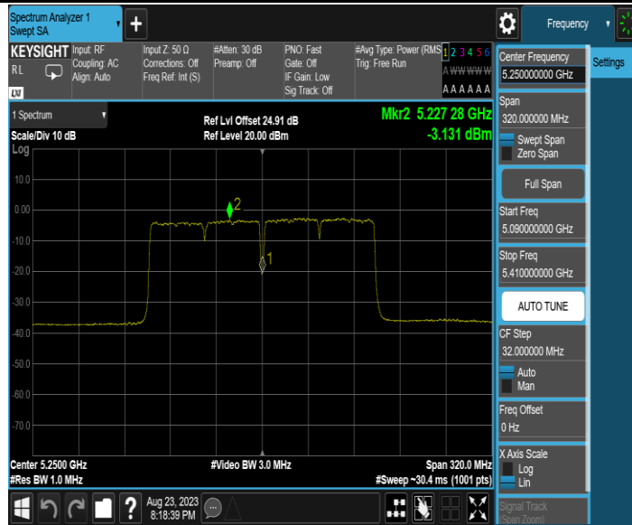
11AC160MIMO_Ant2_5250_UNII-1
