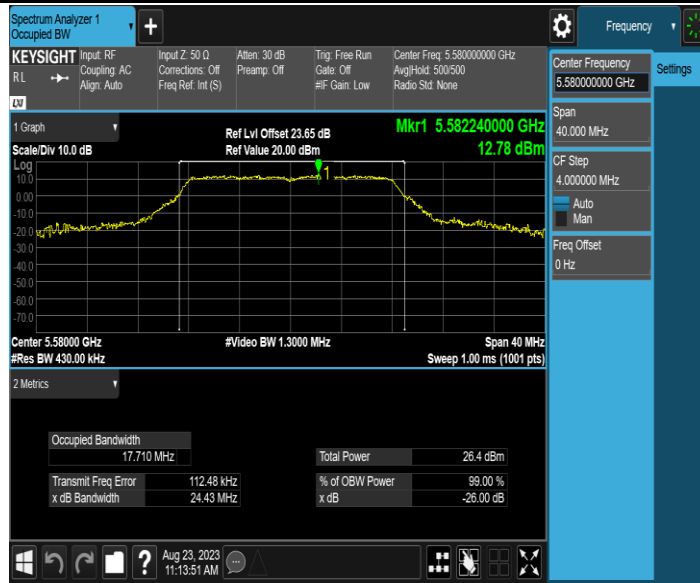
11A_Ant2_5580
