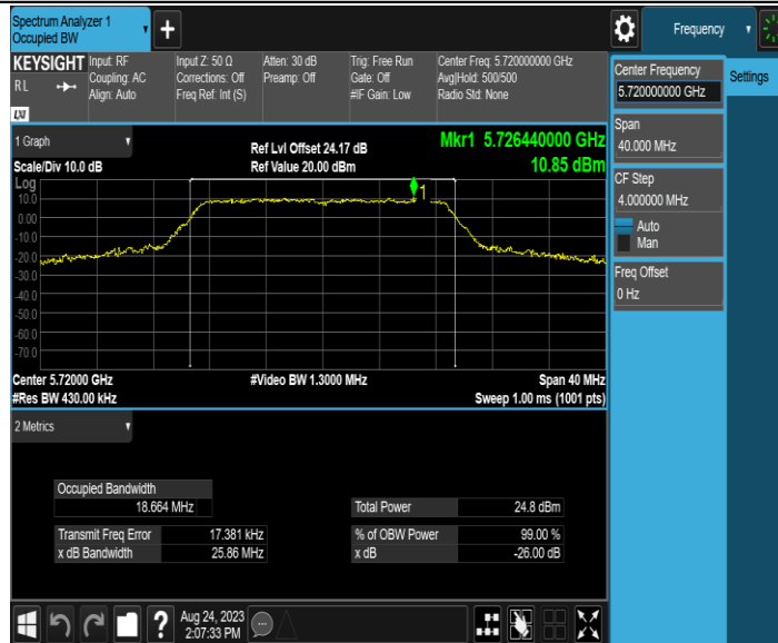
11N20MIMO_Ant2_5720
