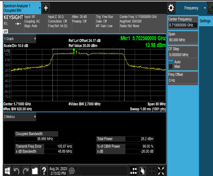
11N40MIMO_Ant2_5710
