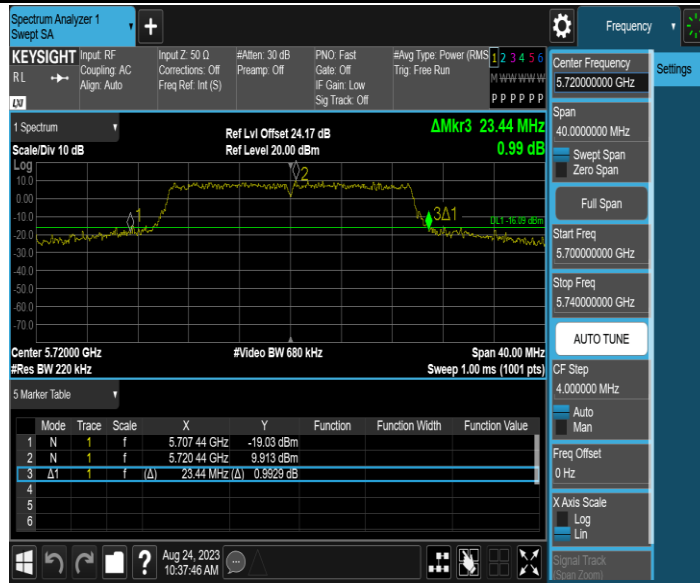
11AX20MIMO_Ant2_5720
