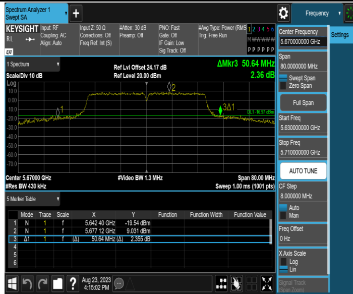
11N40MIMO_Ant2_5670
