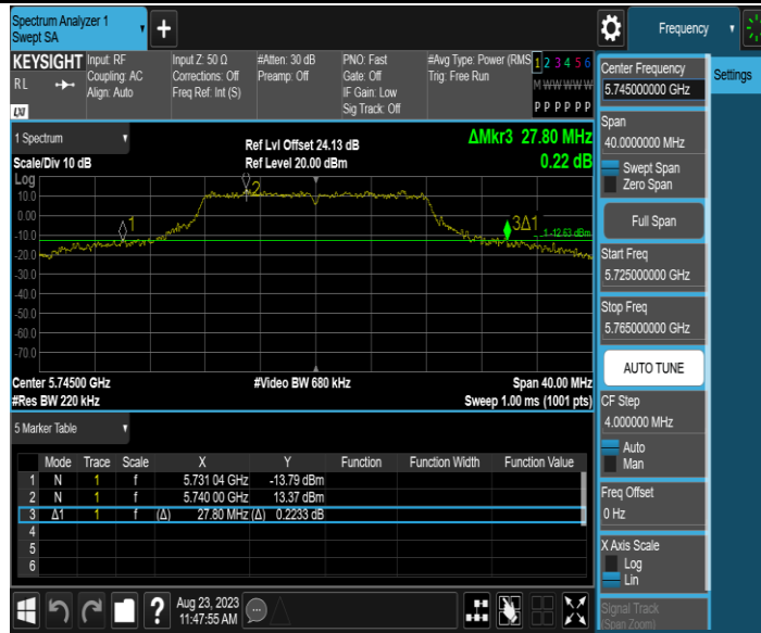
11A_Ant2_5745
