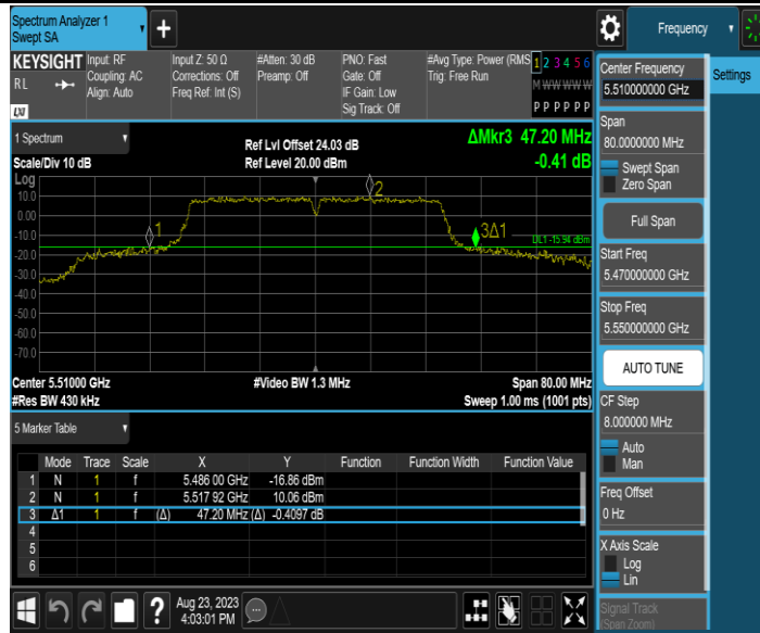
11N40MIMO_Ant2_5510
