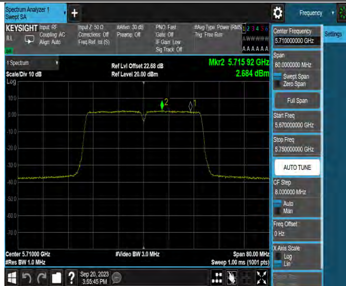
11N40MIMO_Ant3_5710_UNII-2C
