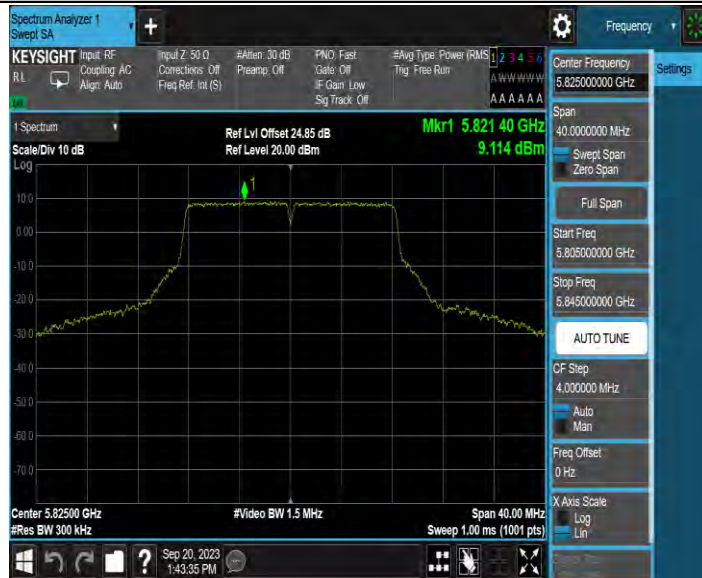
11A-MIMO_Ant3_5825
