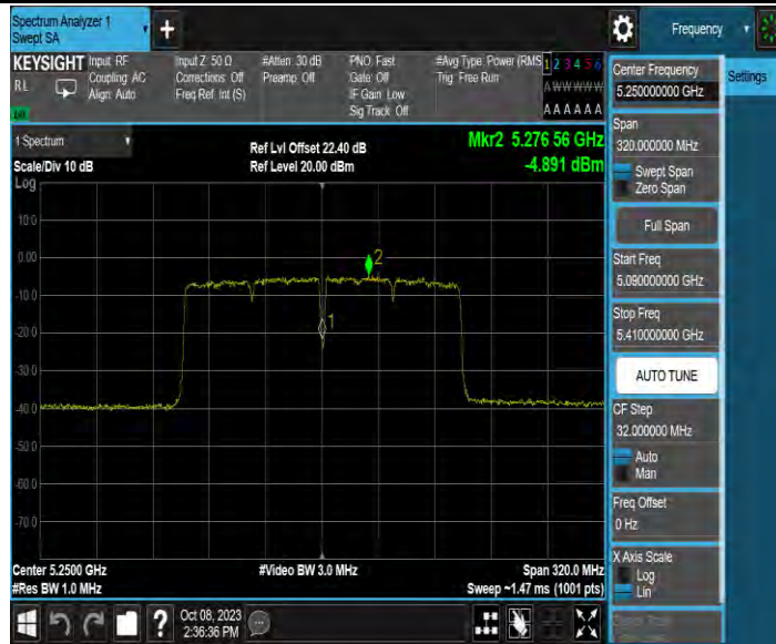
11AC160MIMO_Ant4_5250_UNII-2A
