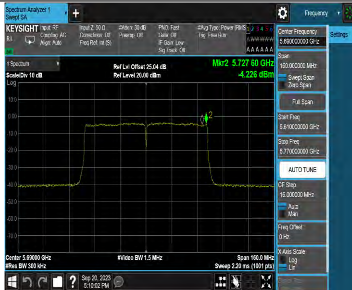
11AC80MIMO_Ant3_5690_UNII-3
