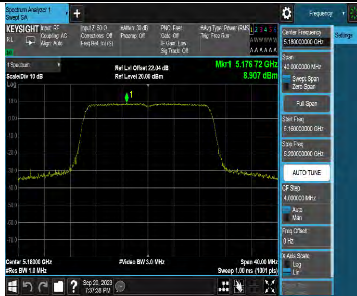
11AX20MIMO_Ant4_5180
