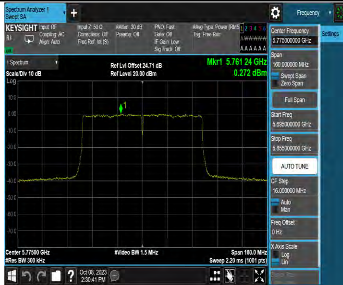
11AC80MIMO_Ant4_5775
