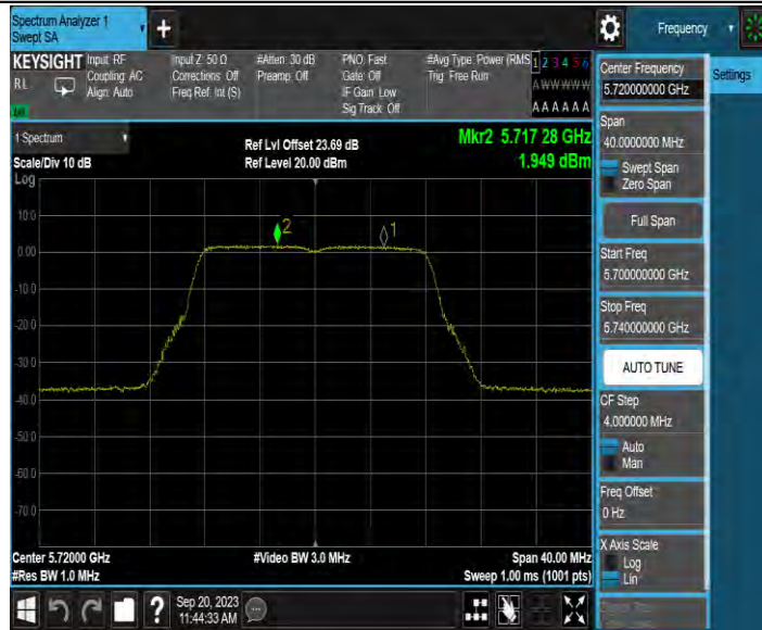
11A-MIMO_Ant1_5720_UNII-3
