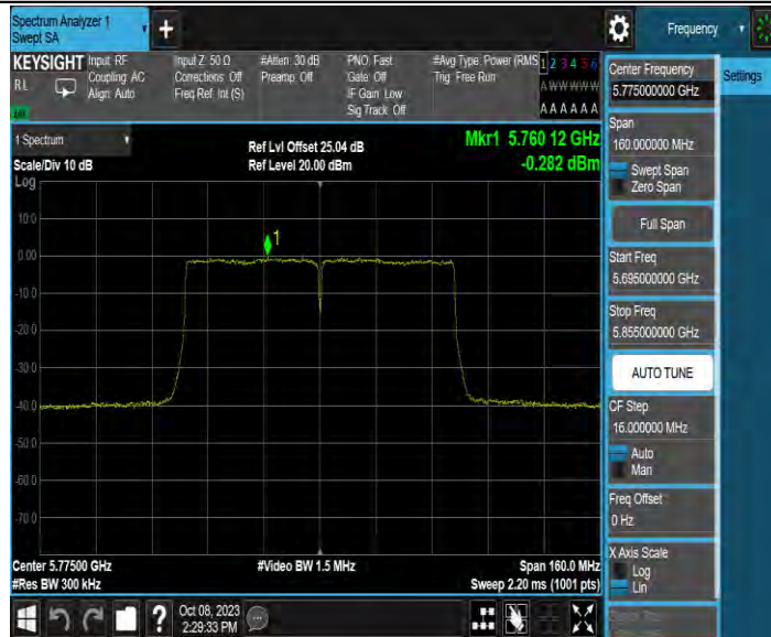
11AC80MIMO_Ant3_5775
