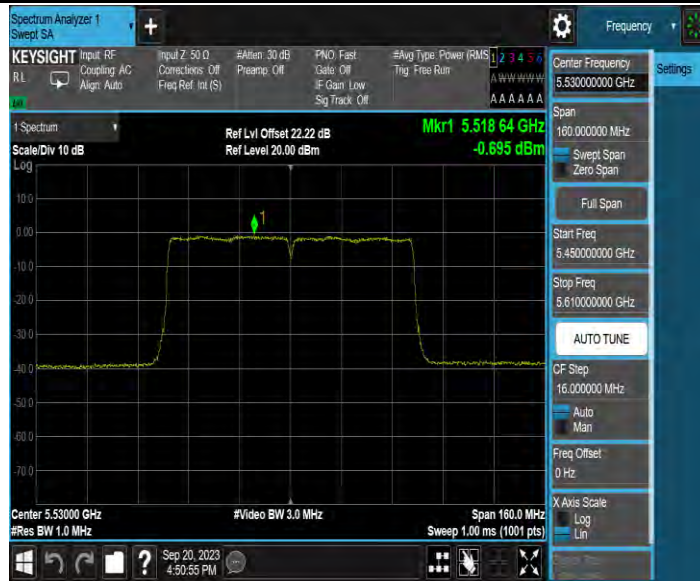
11AC80MIMO_Ant4_5530
