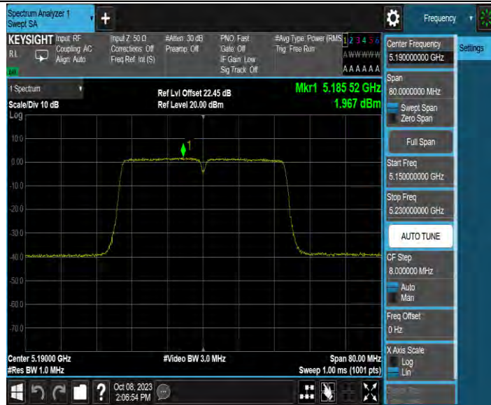
11N40MIMO_Ant3_5190
