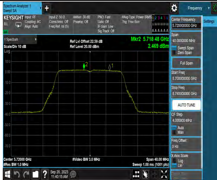
11A-MIMO_Ant2_5720_UNII-2C
