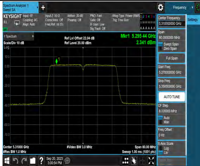
11N40MIMO_Ant4_5310
