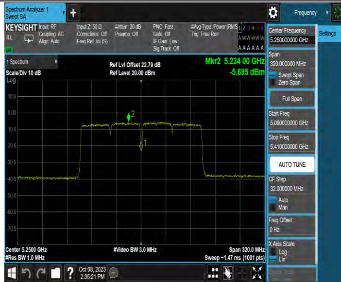
11AC160MIMO_Ant3_5250_UNII-1
