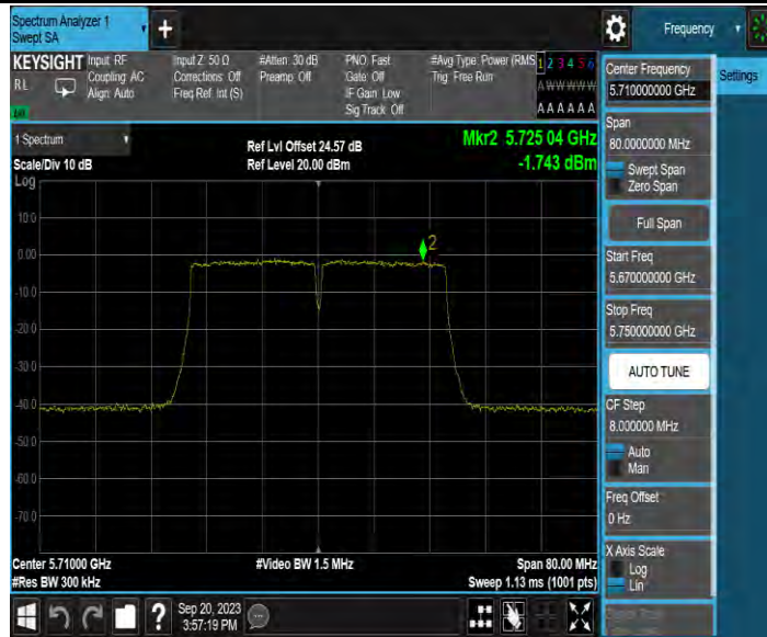
11N40MIMO_Ant4_5710_UNII-3
