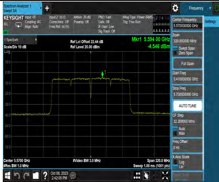
11AC160MIMO_Ant4_5570
