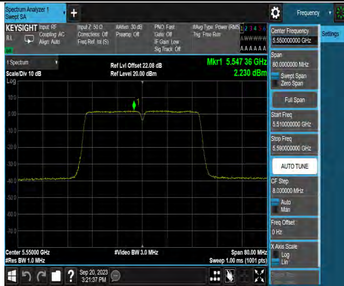
11N40MIMO_Ant4_5550
