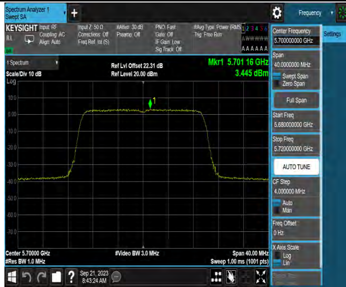
11AX20MIMO_Ant4_5700
