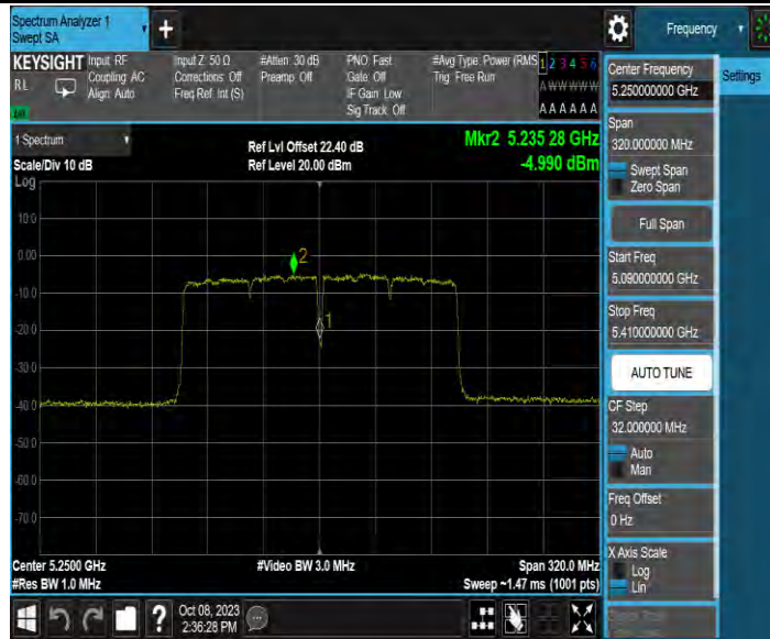
11AC160MIMO_Ant4_5250_UNII-1
