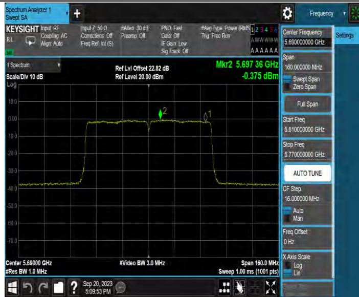
11AC80MIMO_Ant3_5690_UNII-2C
