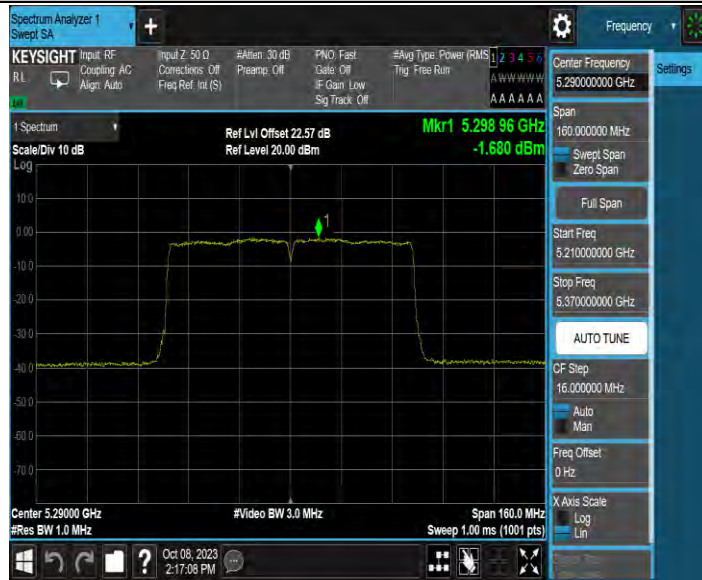
11AC80MIMO_Ant3_5290
