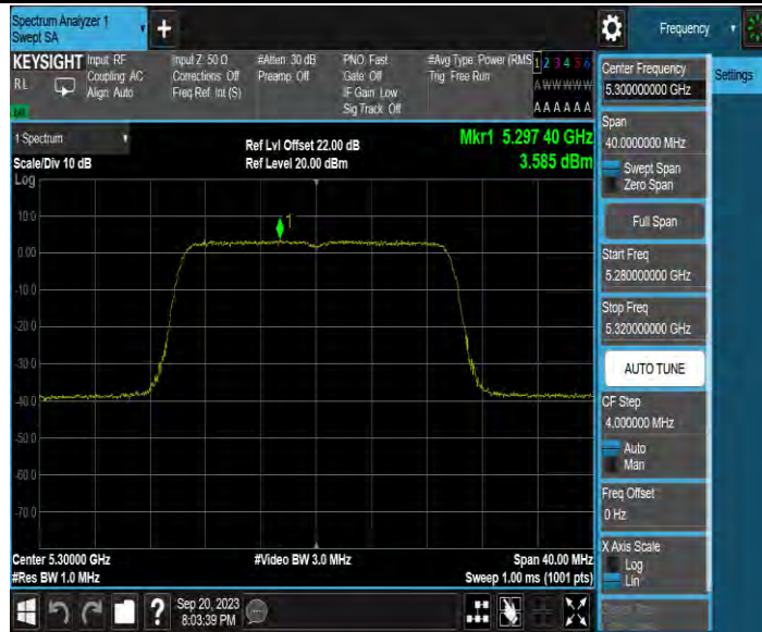
11AX20MIMO_Ant4_5300
