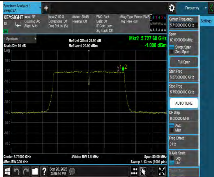
11N40MIMO_Ant3_5710_UNII-3
