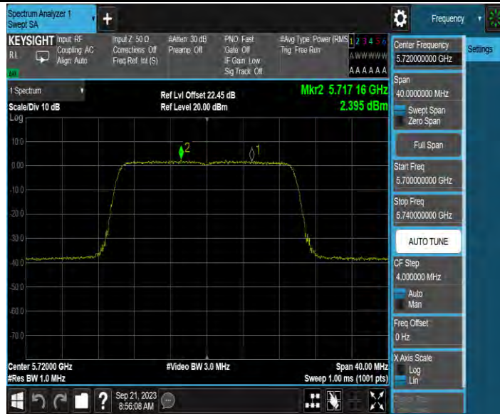
11AX20MIMO_Ant2_5720_UNII-2C
