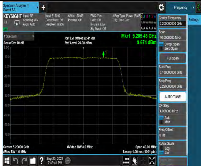
11AX20MIMO_Ant3_5200
