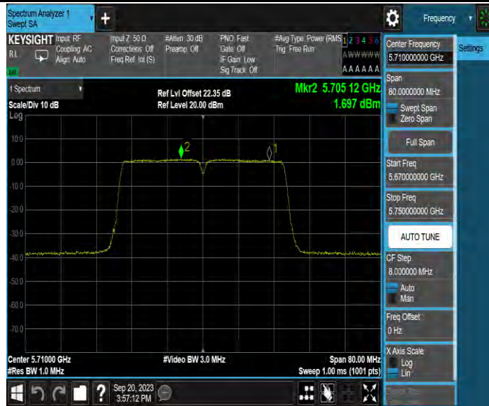
11N40MIMO_Ant4_5710_UNII-2C
