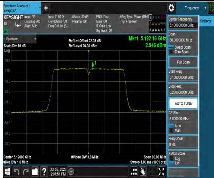
11N40MIMO_Ant4_5190
