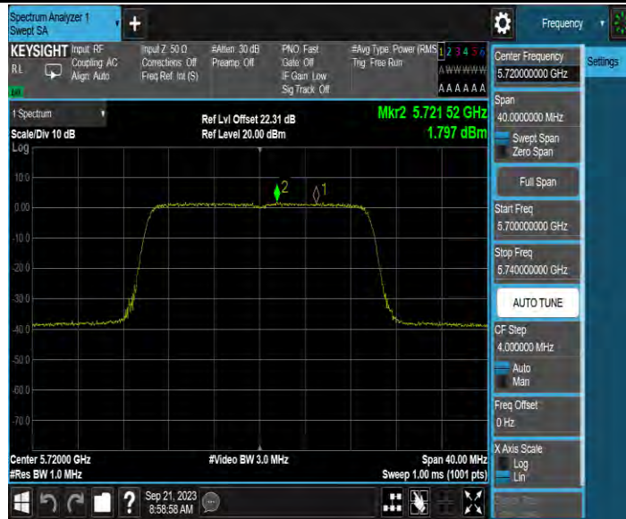
11AX20MIMO_Ant4_5720_UNII-2C
