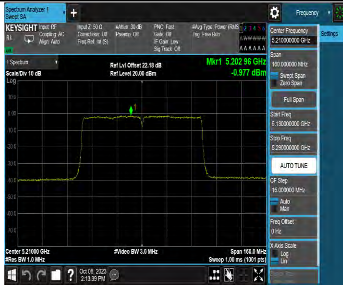
11AC80MIMO_Ant4_5210
