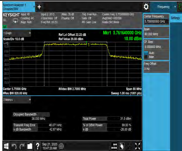
11AX40MIMO_Ant4_5755
