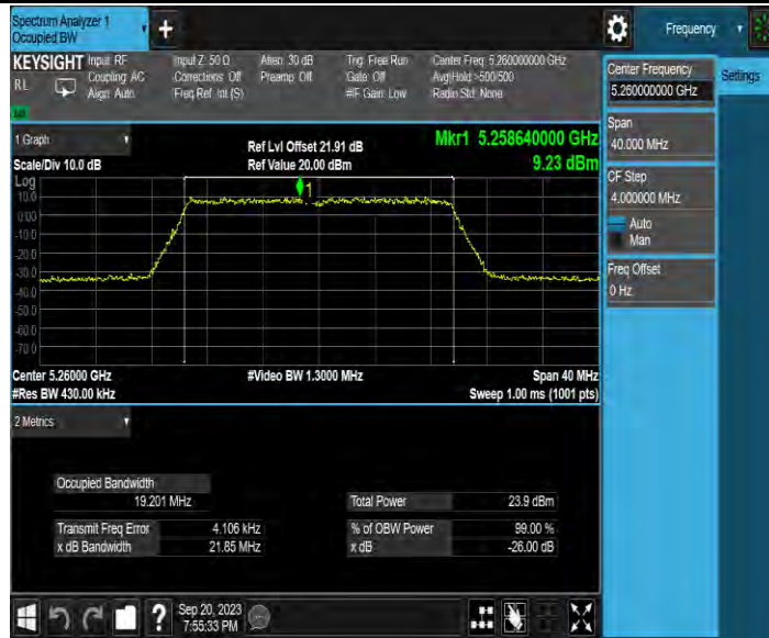
11AX20MIMO_Ant4_5260
