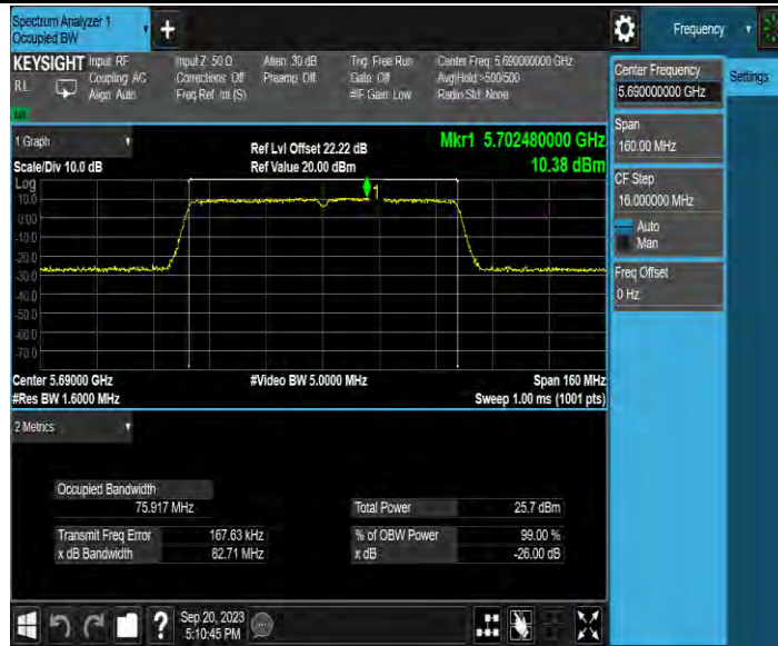
11AC80MIMO_Ant4_5690
