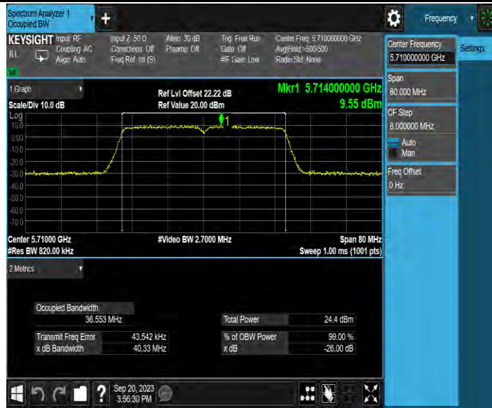
11N40MIMO_Ant4_5710
