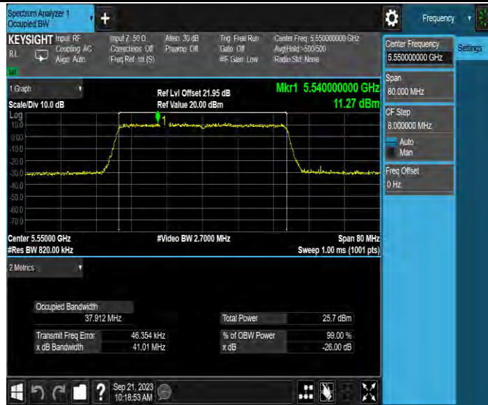
11AX40MIMO_Ant4_5550
