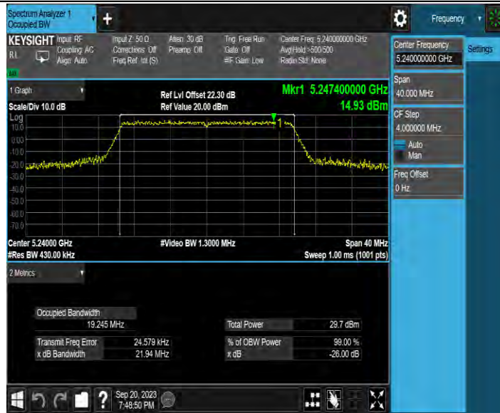
11AX20MIMO_Ant3_5240
