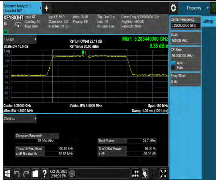
11AC80MIMO_Ant2_5290
