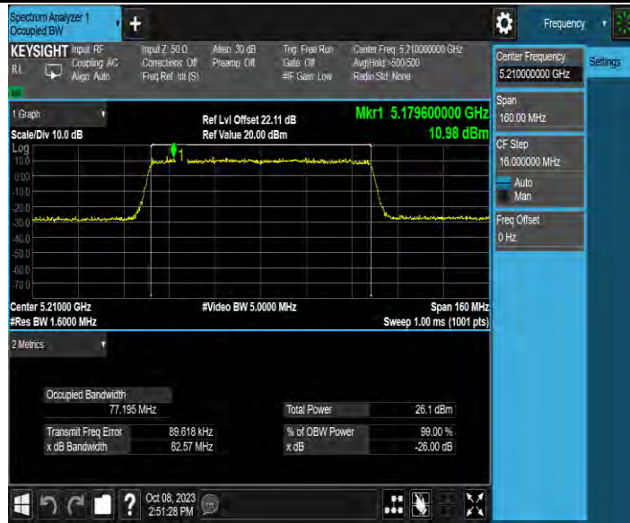
11AX80MIMO_Ant2_5210
