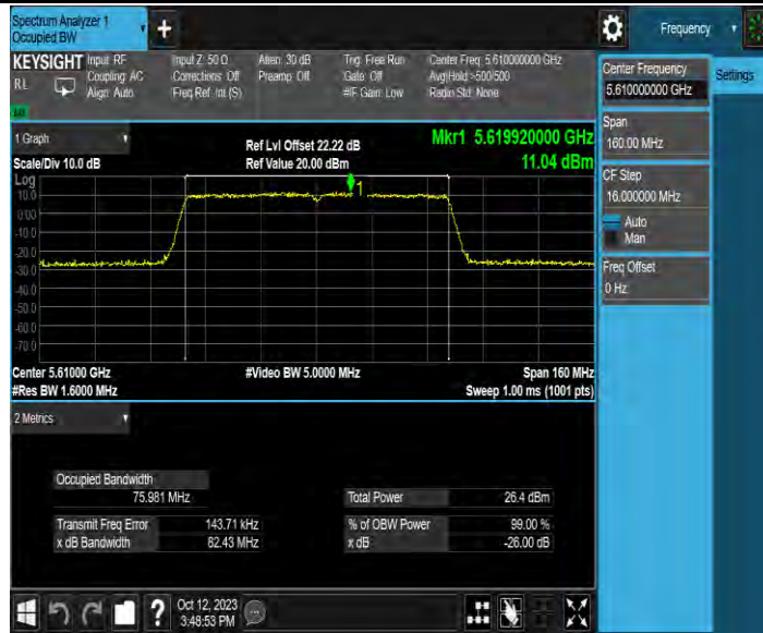
11AC80MIMO_Ant4_5610
