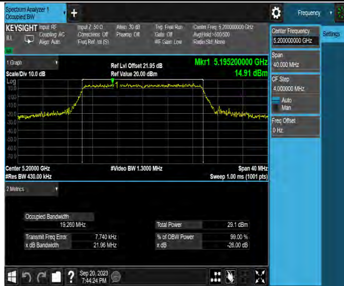
11AX20MIMO_Ant4_5200
