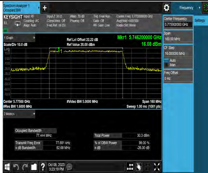
11AX80MIMO_Ant4_5775
