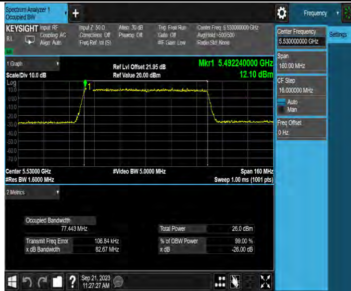
11AX80MIMO_Ant4_5530
