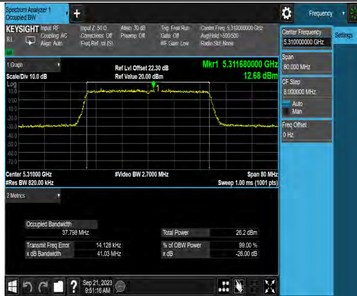
11AX40MIMO_Ant3_5310
