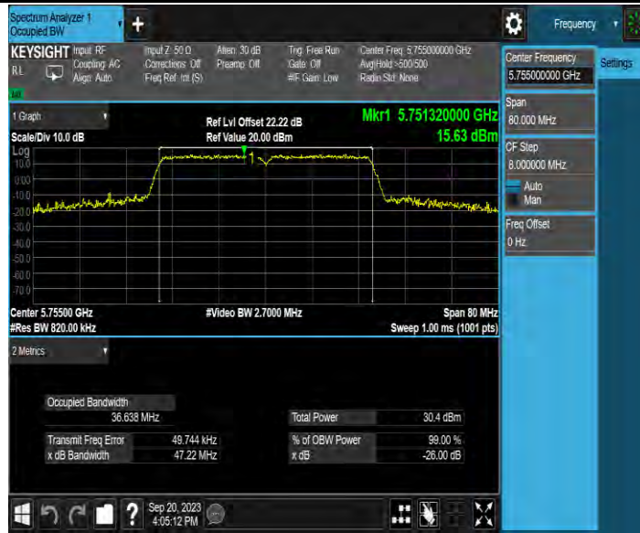
11N40MIMO_Ant4_5755
