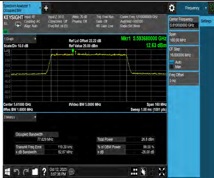
11AX80MIMO_Ant4_5610
