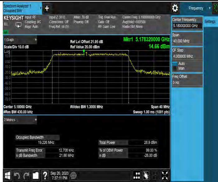
11AX20MIMO_Ant4_5180
