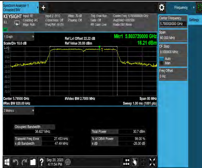
11N40MIMO_Ant4_5795
