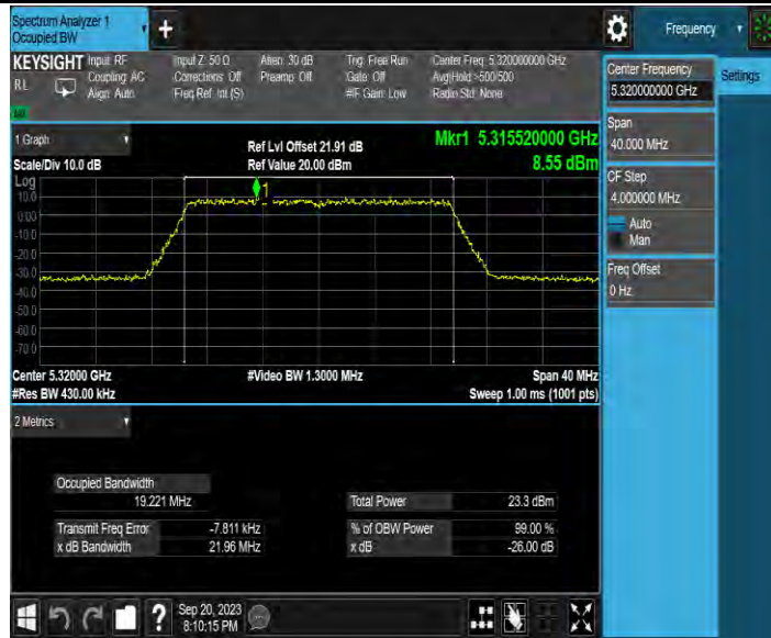
11AX20MIMO_Ant4_5320
