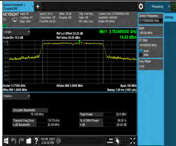
11AC80MIMO_Ant4_5775
