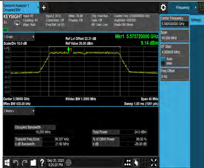
11AX20MIMO_Ant3_5580
