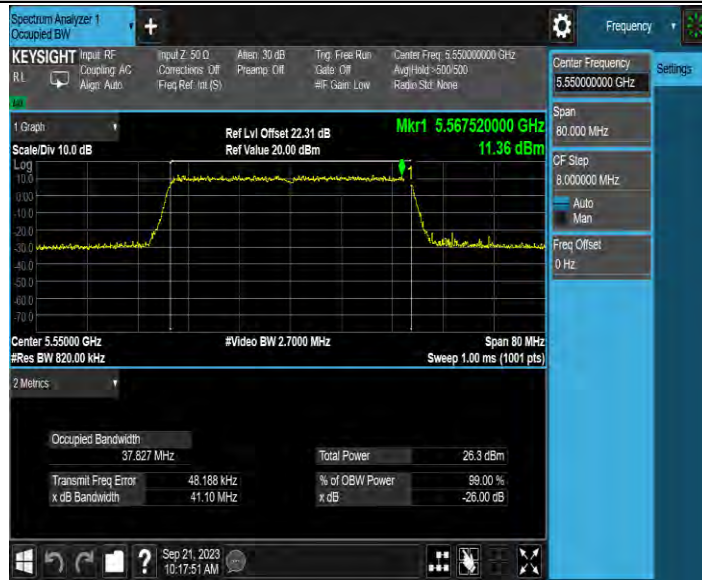
11AX40MIMO_Ant3_5550
