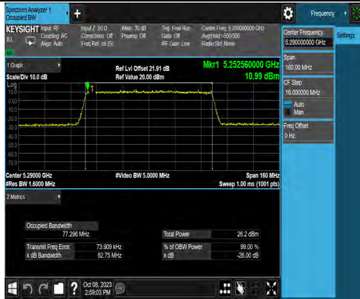
11AX80MIMO_Ant4_5290
