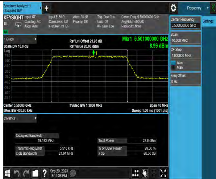
11AX20MIMO_Ant4_5500
