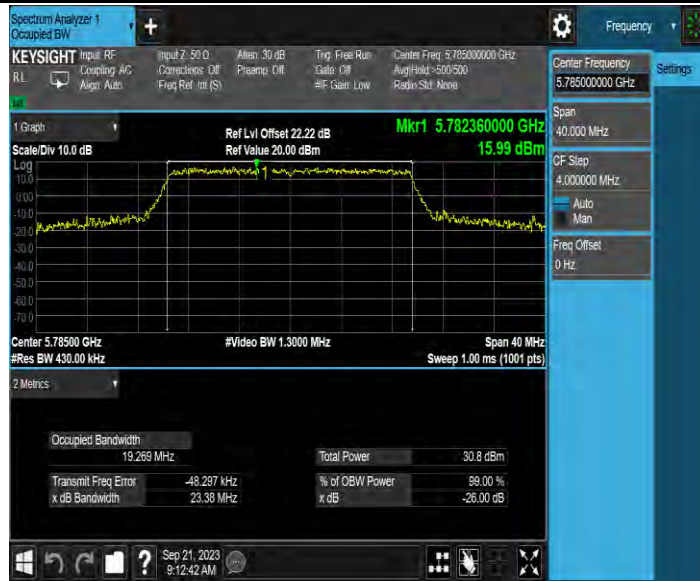
11AX20MIMO_Ant4_5785
