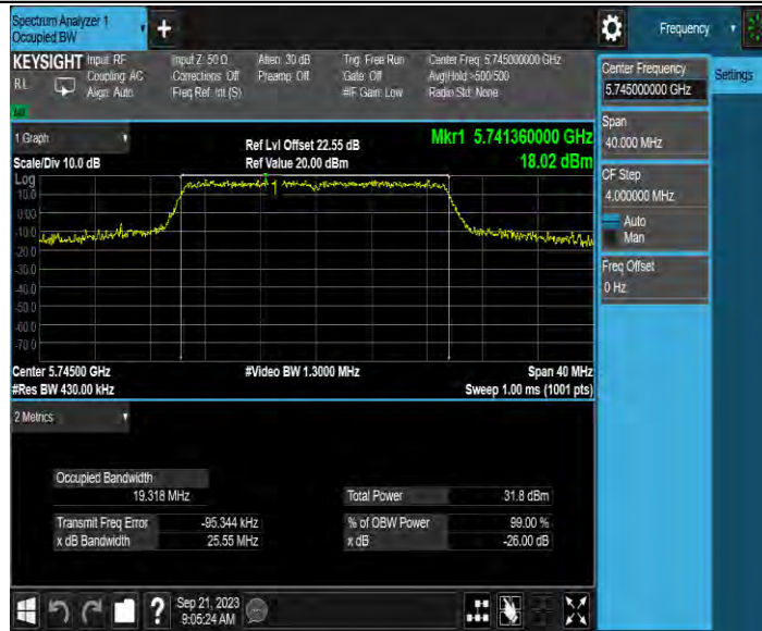
11AX20MIMO_Ant3_5745
