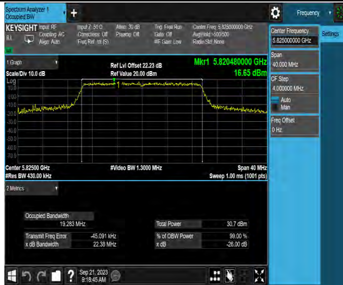
11AX20MIMO_Ant4_5825
