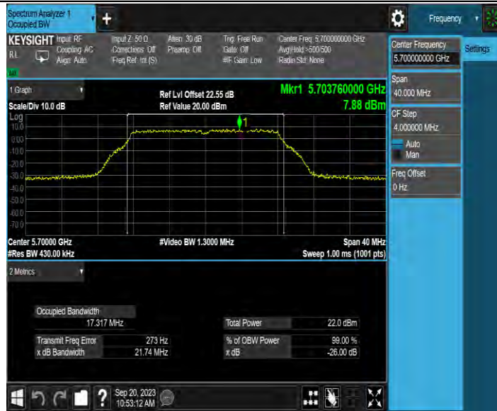
11A-MIMO_Ant3_5700
