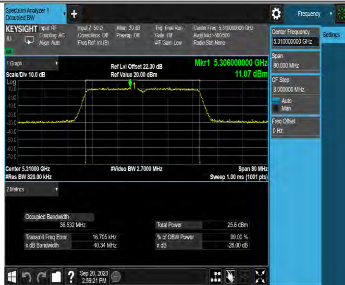
11N40MIMO_Ant3_5310
