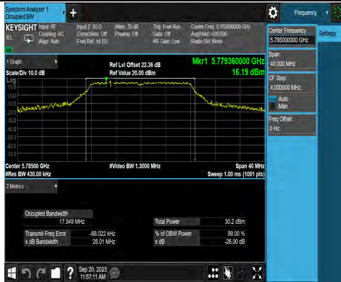
11A-MIMO_Ant2_5785
