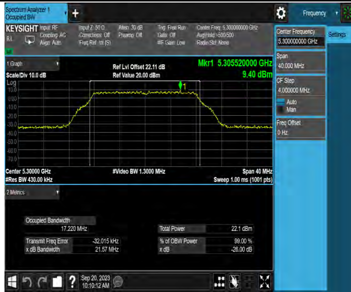
11A-MIMO_Ant2_5300
