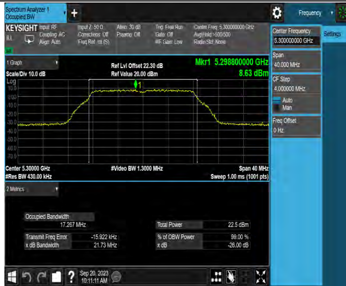
11A-MIMO_Ant3_5300
