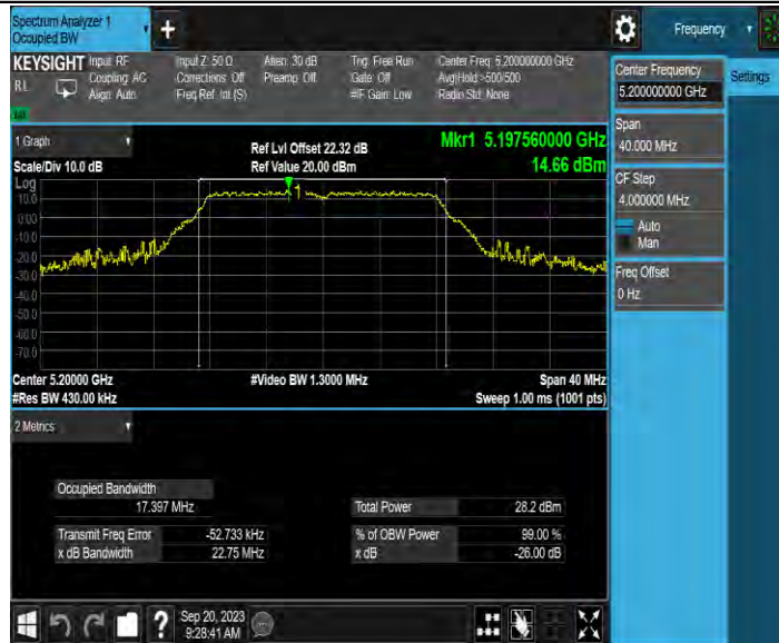
11A-MIMO_Ant3_5200
