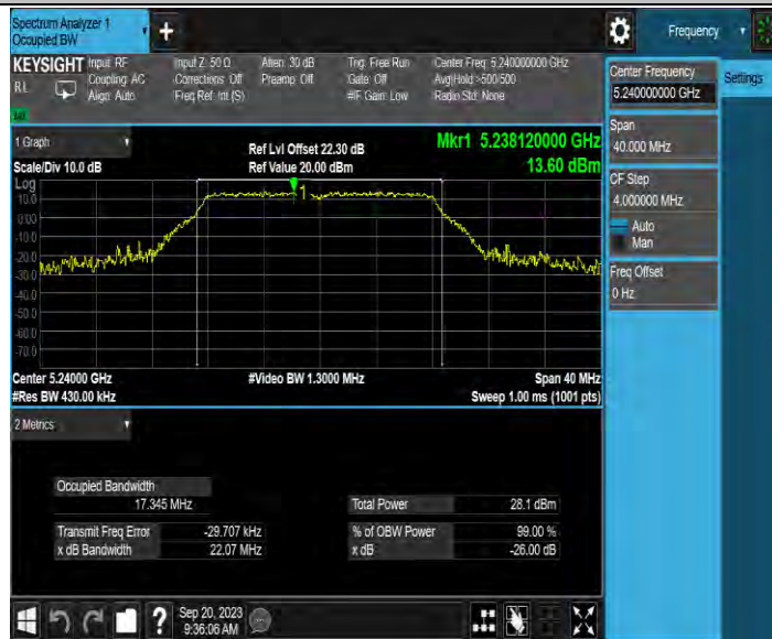
11A-MIMO_Ant3_5240
