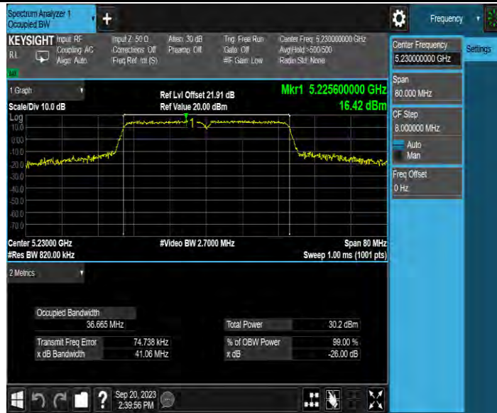
11N40MIMO_Ant4_5230
