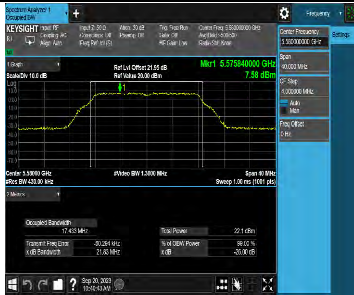
11A-MIMO_Ant4_5580
