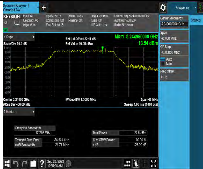
11A-MIMO_Ant2_5240
