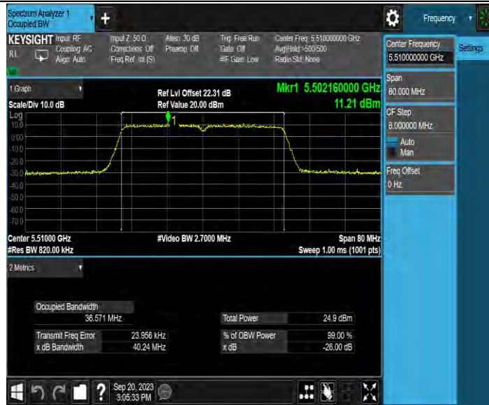
11N40MIMO_Ant3_5510
