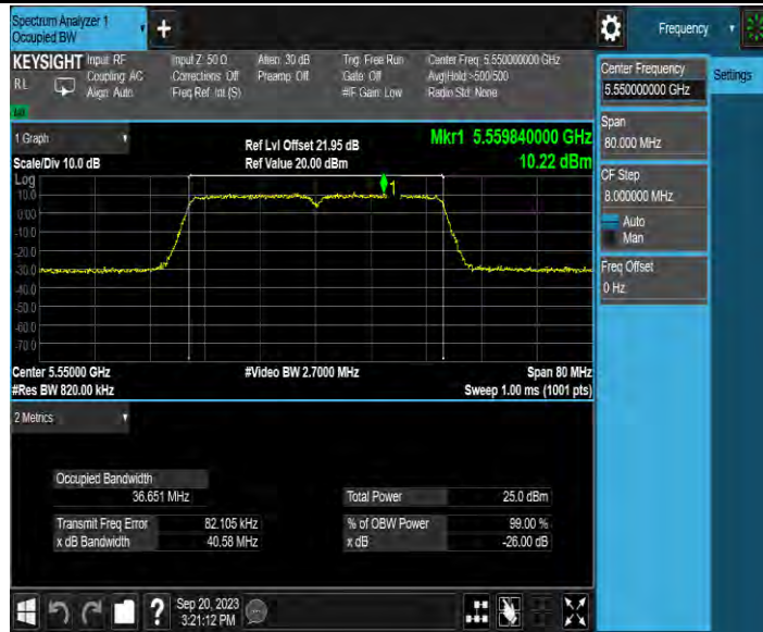
11N40MIMO_Ant4_5550
