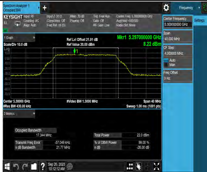
11A-MIMO_Ant4_5300
