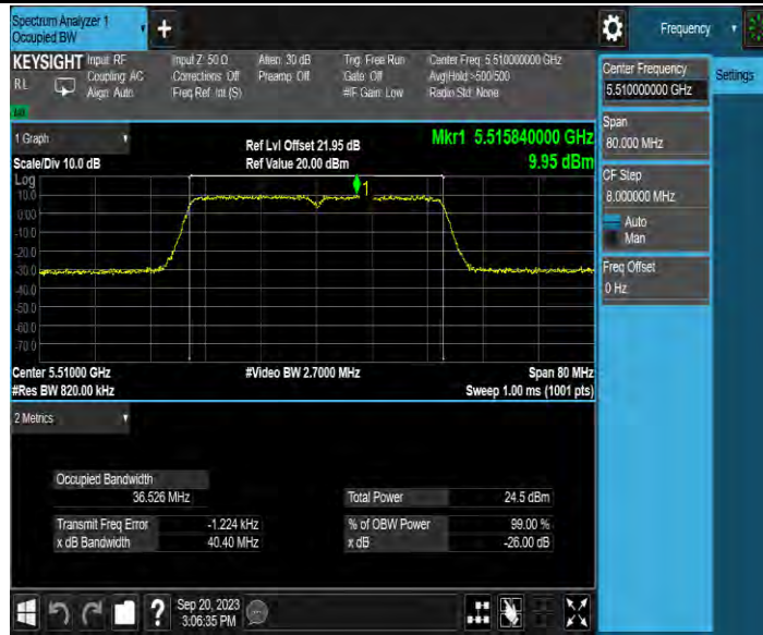
11N40MIMO_Ant4_5510
