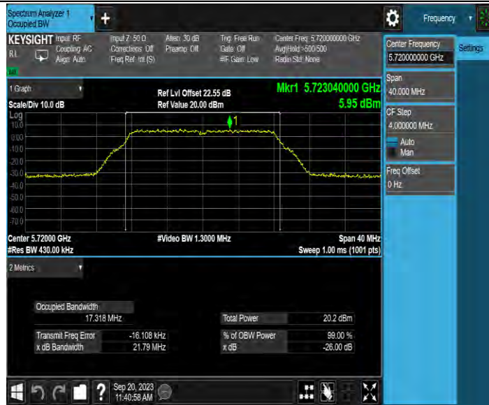
11A-MIMO_Ant3_5720
