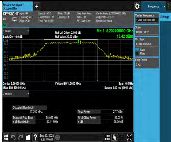
11A-MIMO_Ant2_5200
