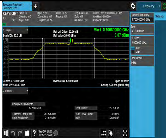
11A-MIMO_Ant2_5700
