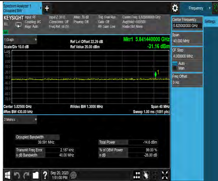
11A-MIMO_Ant2_5825
