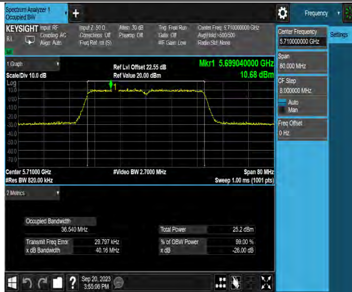
11N40MIMO_Ant3_5710
