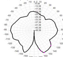
2420.0MHz Total(E+XZ), Max=-14.94dB
