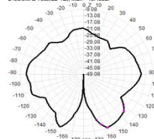
2410.0MHz Total(E+XZ), Max=-14.79dB
