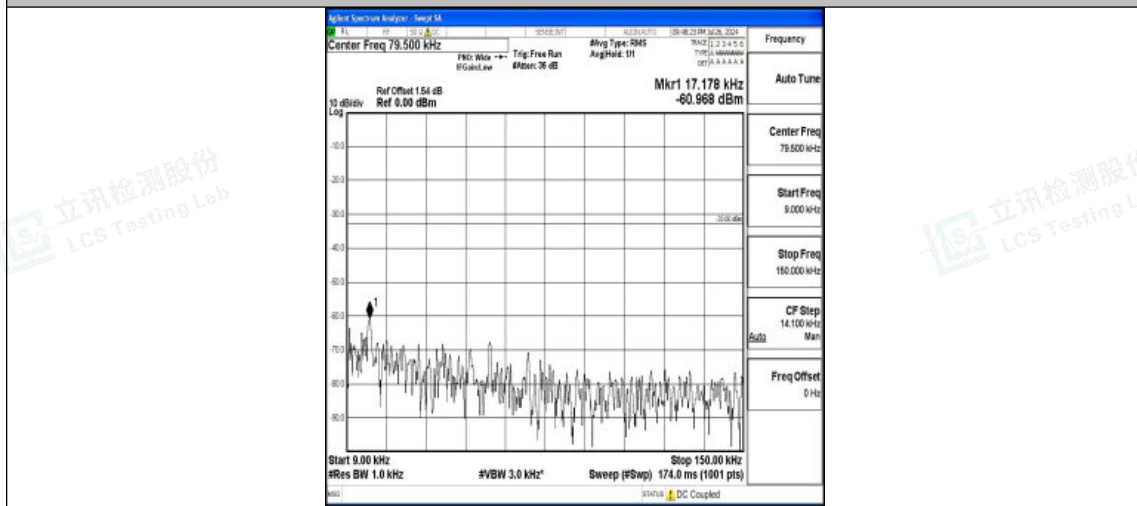
Band5-3MHz-QPSK-20635-1RB#0-0.009~0.15-PASS
