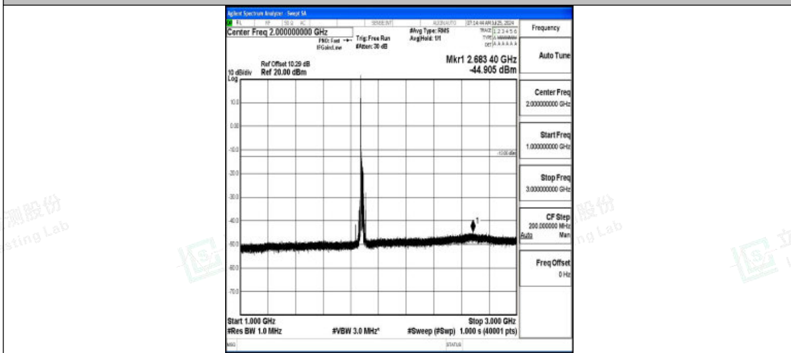
Band2-20MHz-QPSK-18900-1RB#0-1000~3000-PASS
