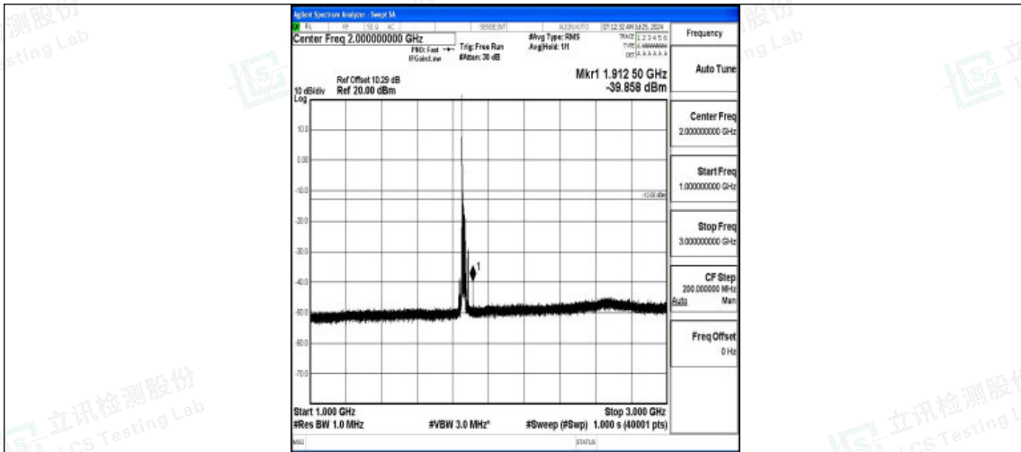
Band2-20MHz-QPSK-18700-1RB#0-1000~3000-PASS
