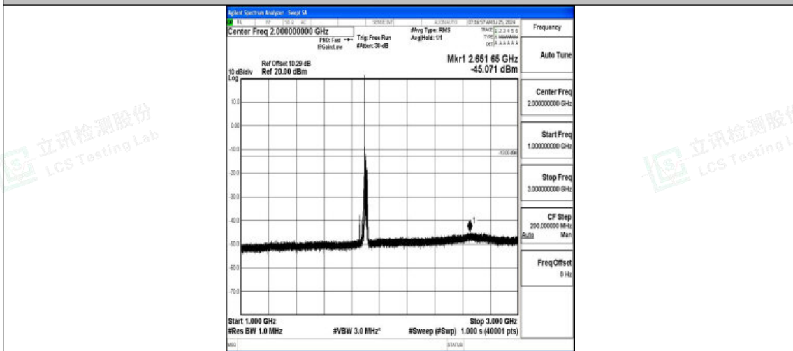
Band2-20MHz-QPSK-19100-1RB#0-1000~3000-PASS
