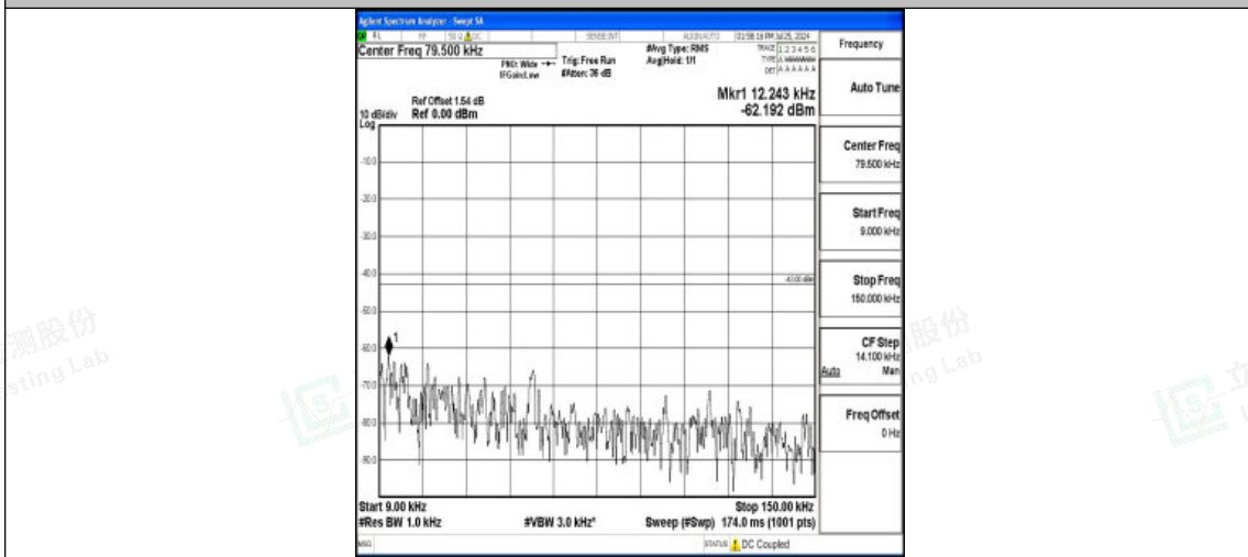
Band4-20MHz-QPSK-20175-1RB#0-0.009~0.15-PASS
