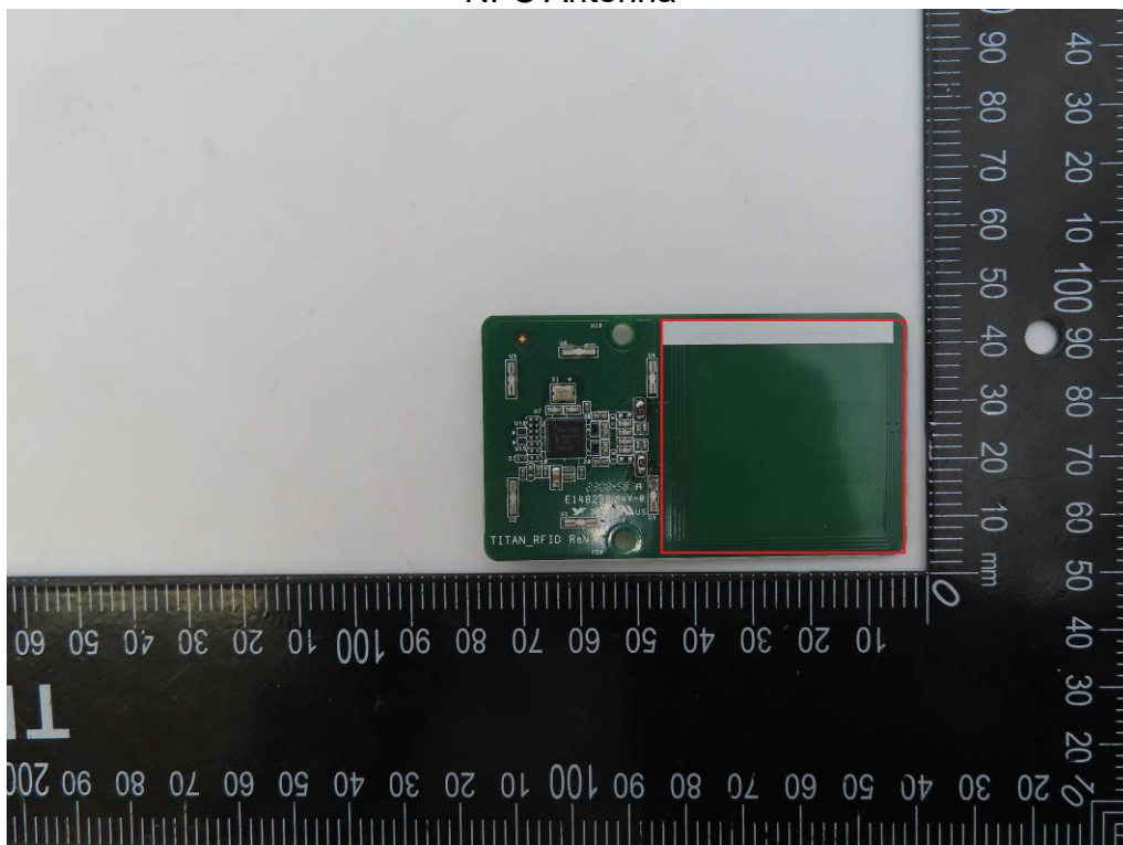
NFC Antenna
