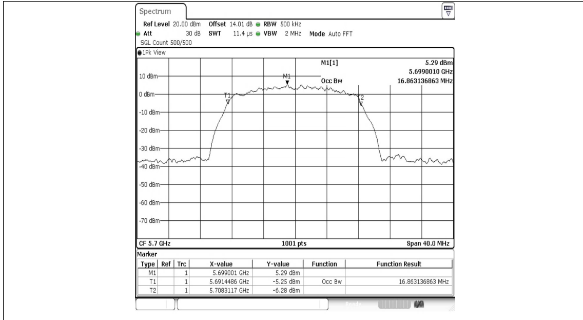
11A-Ant1-5700
