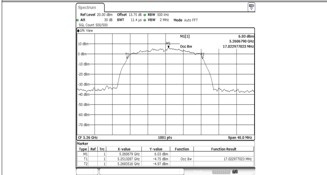
11A-Ant1-5260
