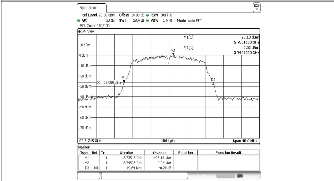
11A-Ant1-5745
