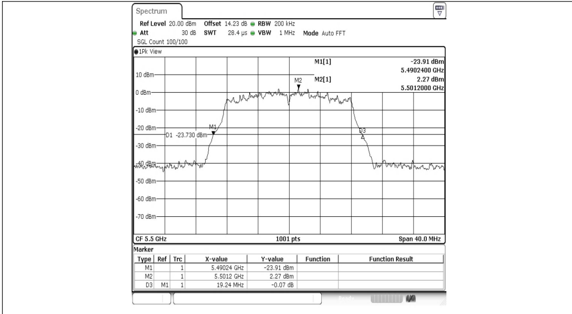
11A-Ant1-5500
