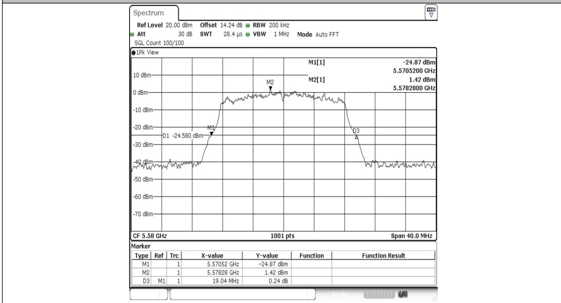
11A-Ant1-5580
