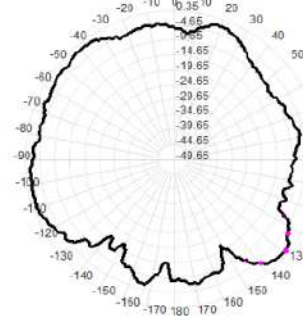
5750.0MHz Total(E1), Max=-0.83dBi
