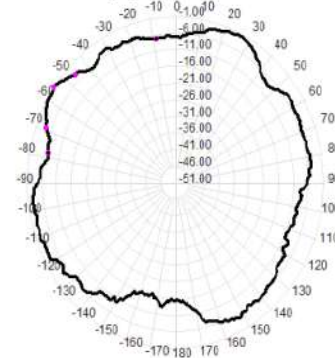
5850.0MHz Total(E2), Max=-1.00dBi
