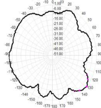
5850.0MHz Total(E1), Max=-1.37dBi
