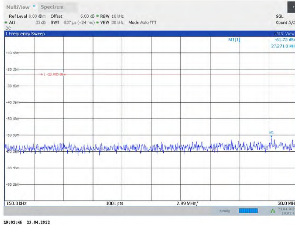
Band42-20MHz-QPSK-42190-1RB#0-Range2:0.15~30MHz
